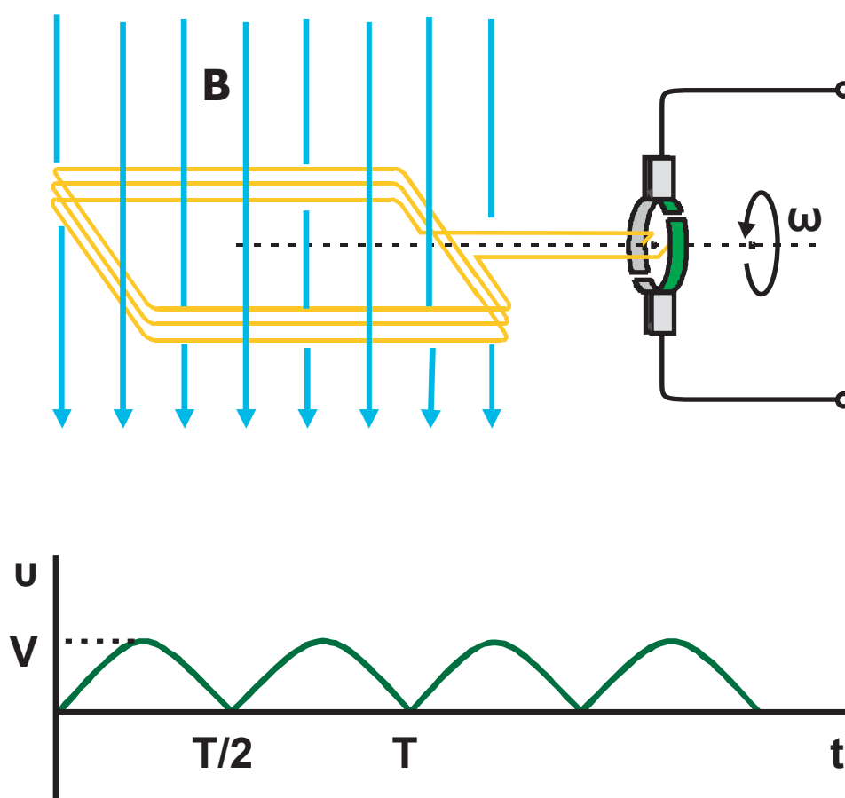
Σχ. 5.26 Αρχή λειτουργίας της γεννήτριας συνεχούς τάσεως.
