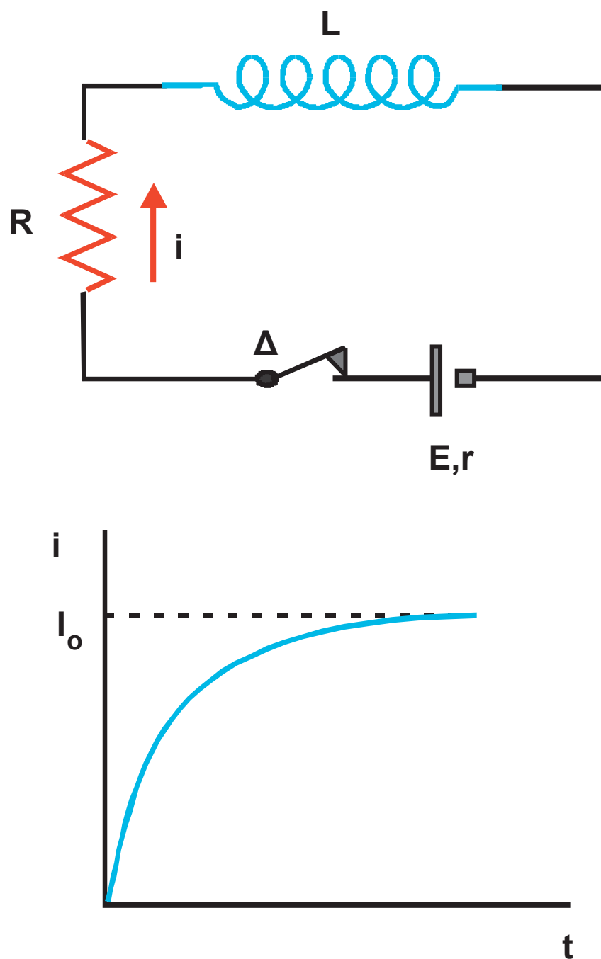
Σχ. 5.36 Μετά το κλείσιμο του διακόπτη το ρεύμα καθυστερεί να πάρει την τελική του τιμή.
