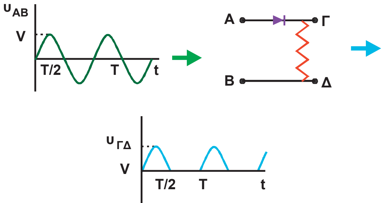
Σχ. 5.27 Διάταξη ανόρθωσης της εναλλασσόμενης τάσης. Η εναλλασσόμενη τάση u_{AB} στην είσοδο του κυκλώματος μετατρέπεται σε συνεχή u_{\Gamma\Delta} στην έξοδο.
