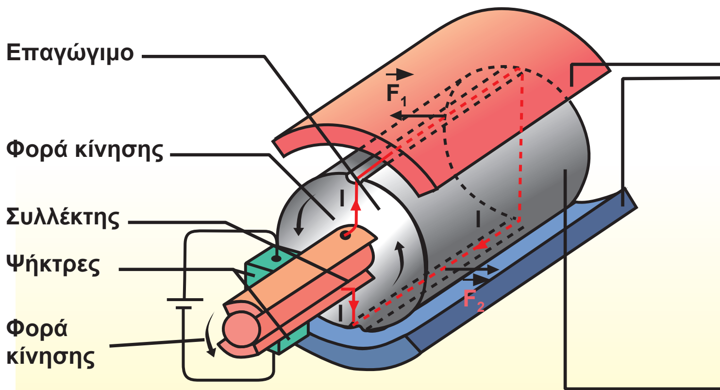
Σχ. 5.31 Ηλεκτροκινητήρας (αρχή λειτουργίας).
