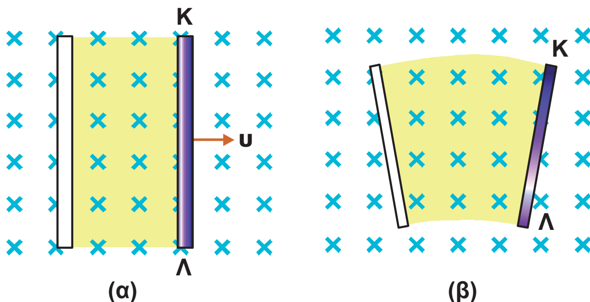
Σχ. 5.8 Στην περίπτωση ενός αγωγού που κινείται μέσα σε μαγνητικό πεδίο, \Delta\Phi είναι η μαγνητική ροή που διέρχεται από την επιφάνεια που ορίζει ο αγωγός με την κίνησή του.
