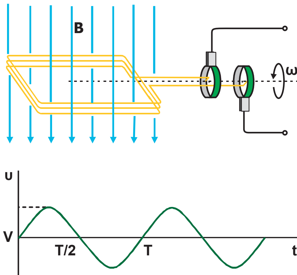
Σχ. 5.23 Αρχή λειτουργίας γεννήτριας εναλλασσόμενης τάσης (εναλλακτήρας).
