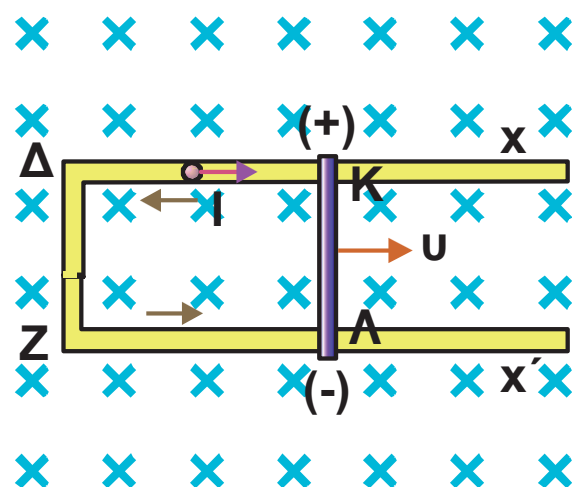
Σχ. 5.6 Ο αγωγός ΚΛ ολισθαίνει πάνω στους ακίνητους αγωγούς xΔZx'. Όλο το σύστημα βρίσκεται μέσα σε ομογενές μαγνητικό πεδίο. Η συσσώρευση φορτίου στα άκρα του αγωγού ΚΛ, προκαλεί κίνηση φορτίου στους ακίνητους αγωγούς.
