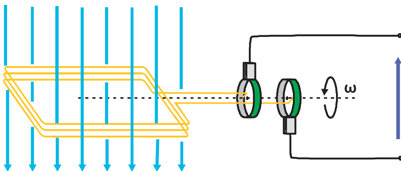
Σχ. 5.18 Το πλαίσιο στρέφεται με σταθερή γωνιακή ταχύτητα \omega μέσα σε ομογενές μαγνητικό πεδίο.
