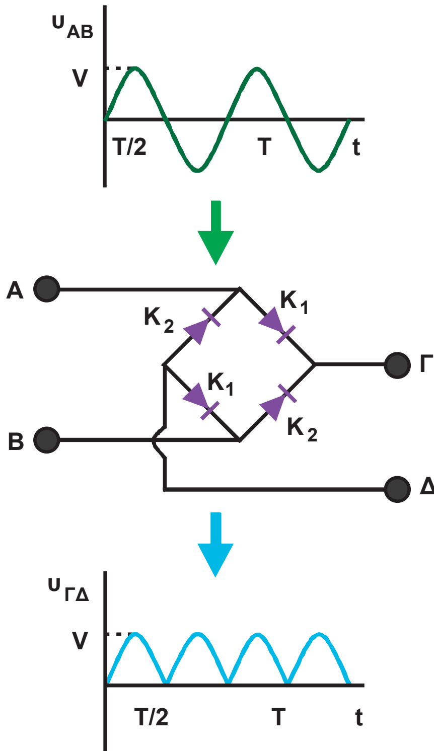
Σχ. 5.28 Διάταξη με τέσσερις διόδους που μετατρέπει την εναλλασσόμενη τάση σε πλήρως ανορθωμένη. Κατά τη μία ημιπερίοδο της τάσης εισόδου όταν το σημείο A είναι σε ψηλότερο δυναμικό από το σημείο B , άγουν οι διόδοι K_1 , ενώ κατά την άλλη ημιπερίοδο άγουν οι διόδοι K_2 .
