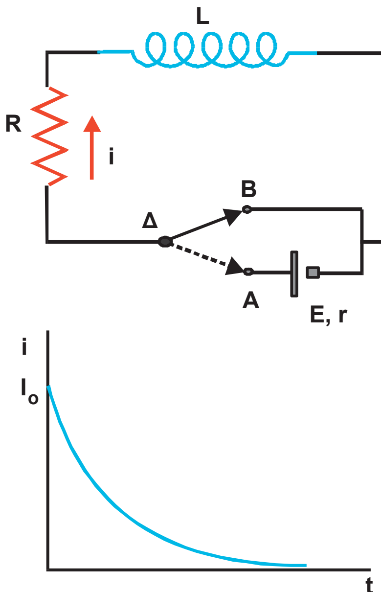
Σχ. 5.37 Η μετακίνηση του μεταγωγού από τη θέση A στη θέση B δε μηδενίζει αμέσως το ρεύμα στο κύκλωμα εξαιτίας της ηλεκτρεγερτικής δύναμης από αυτεπαγωγή που αναπτύσσεται στο πηνίο.
