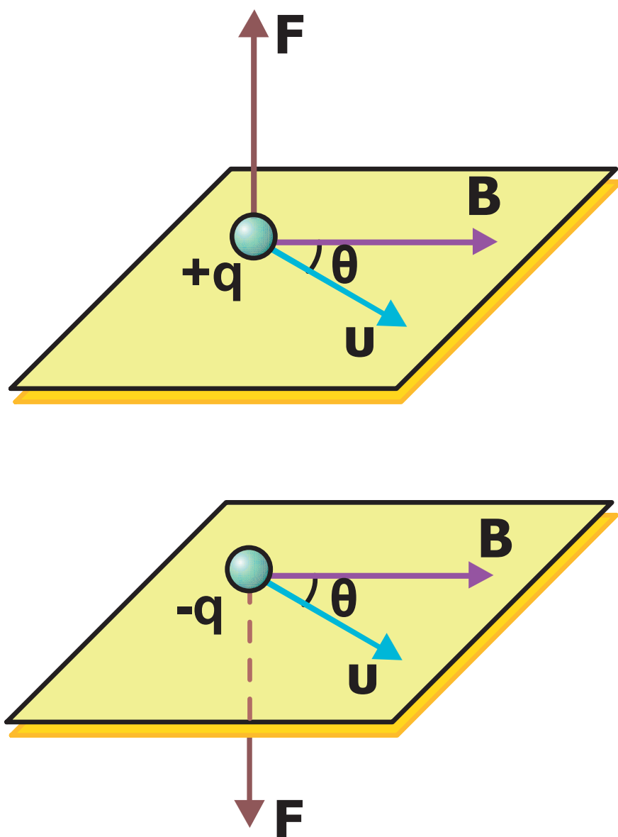
Σχ. 4.14 Η δύναμη που ασκείται από το μαγνητικό πεδίο σε ένα θετικό και ένα αρνητικό σωματίδιο που κινείται με ταχύτητα u .
