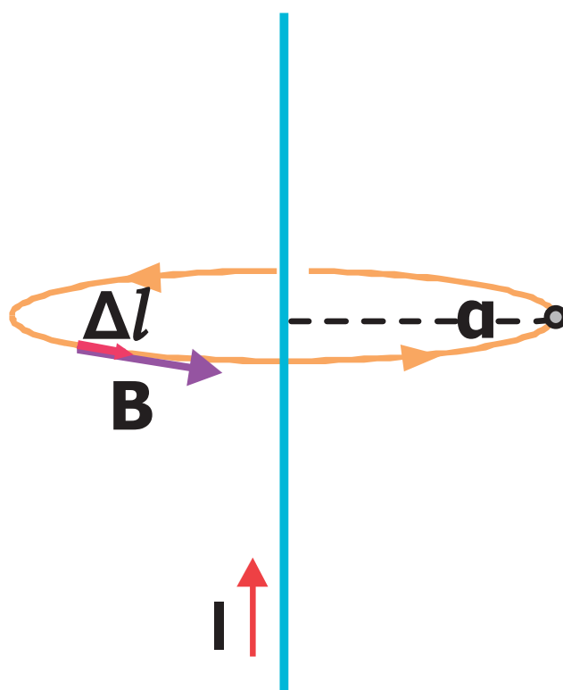
Σχ. 4.6 Κατά μήκος της δυναμικής γραμμής τα \Delta l και B είναι συγγραμμικά ( \theta = 0 ).
