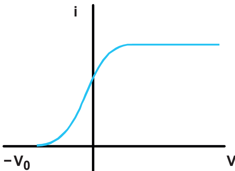
Διάγραμμα της έντασης του ρεύματος σε συνάρτηση με την τάση στο φωτοκύτταρο. Σχήμα 7-4.
