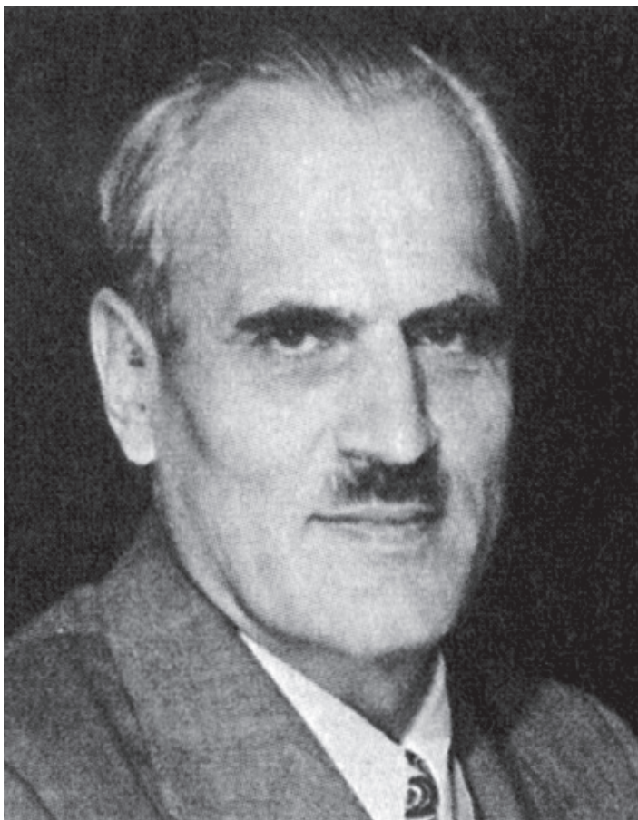
Arthur Holly Compton (1892-1962) Αμερική. Εικόνα 7.3
