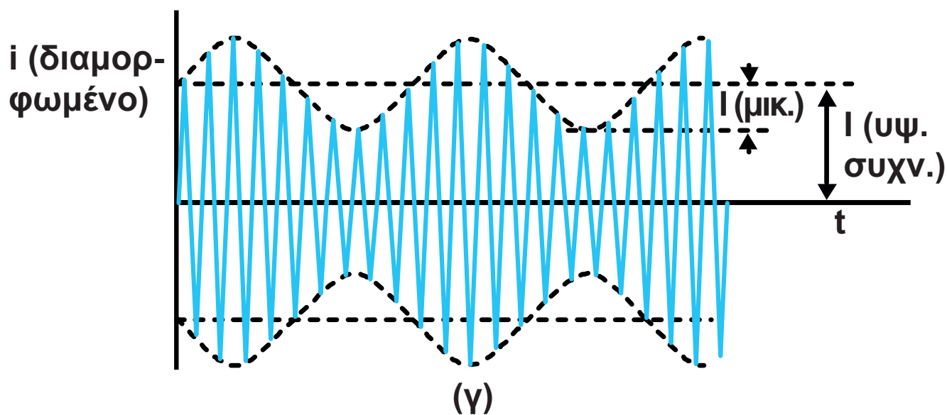
(α) Μικροφωνικό ρεύμα (β) ρεύμα υψηλής συχνότητας (γ) διαμορφωμένο ρεύμα. Σχήμα 2-22.
