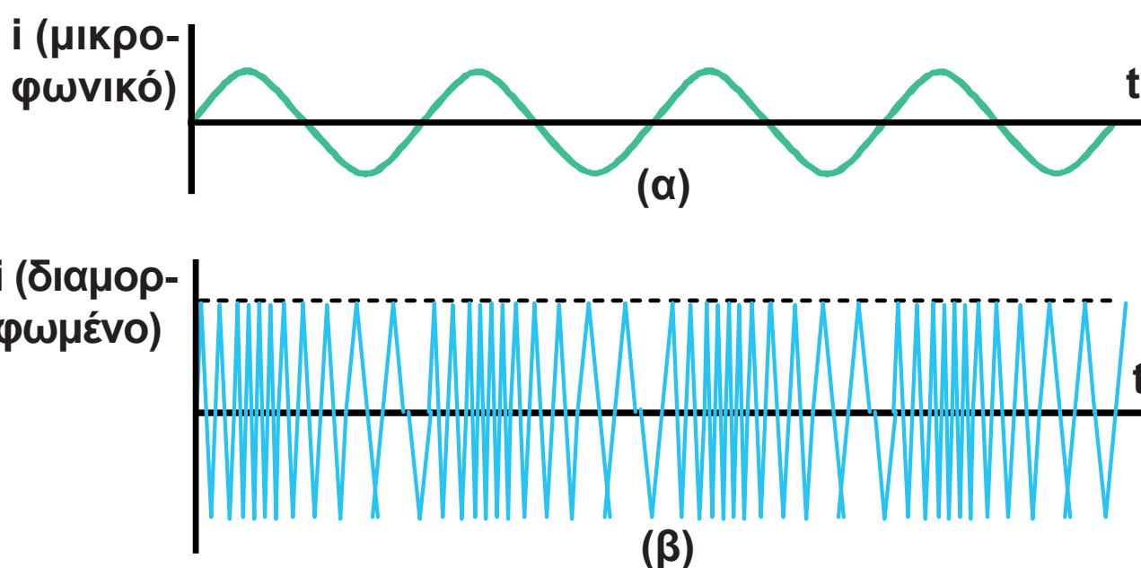
(α) Μικροφωνικό ρεύμα (β) ρεύμα διαμορφωμένο κατά συχνότητα Σχήμα 2-23.
