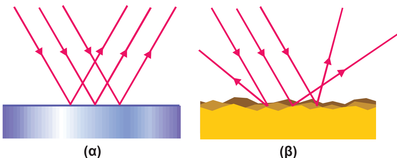
(α) Κατοπτρική ανάκλαση (β) διάχυση Σχήμα 2-27.
