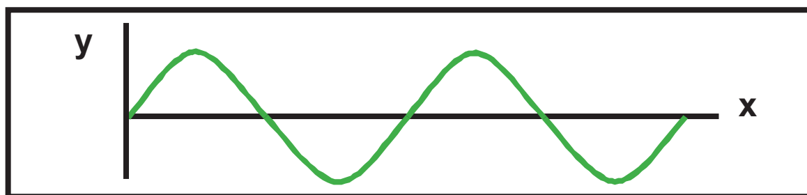
Στιγμιότυπο εγκάρσιου αρμονικού κύματος. Σχήμα 2-4.
