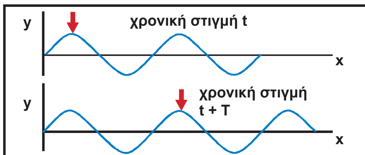
Μετά από χρόνο μιας περιόδου η κυματική εικόνα επαναλαμβάνεται. Σχήμα 2-5.
