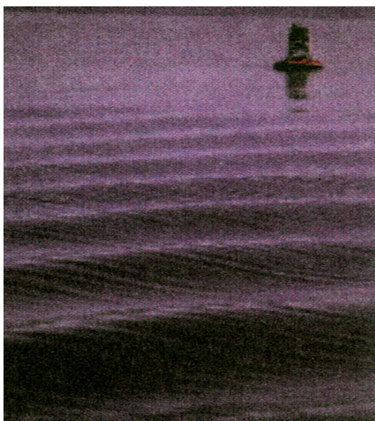
Κύμα στην επιφάνεια της θάλασσας. Εικόνα 2-1.
