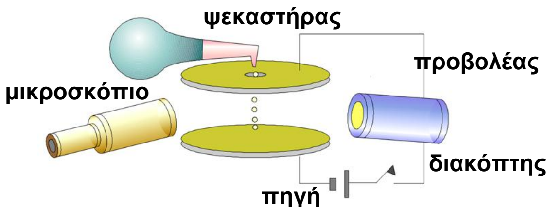
Σχ. 5.61 Το μοντέλο της συσκευής του Millikan
