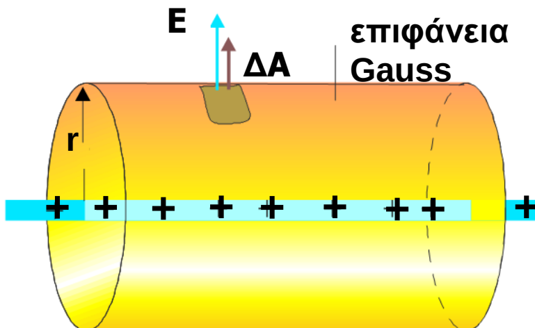
Σχ. 5.14 Επιλέγουμε επιφάνεια Gauss μια κυλινδρική επιφάνεια ομοαξονική με το σύρμα.
