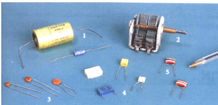
Εικ.5.6 Τύποι πυκνωτών
