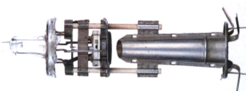
Εικ. 5.3 Τηλεβόλο ηλεκτρονίων.
