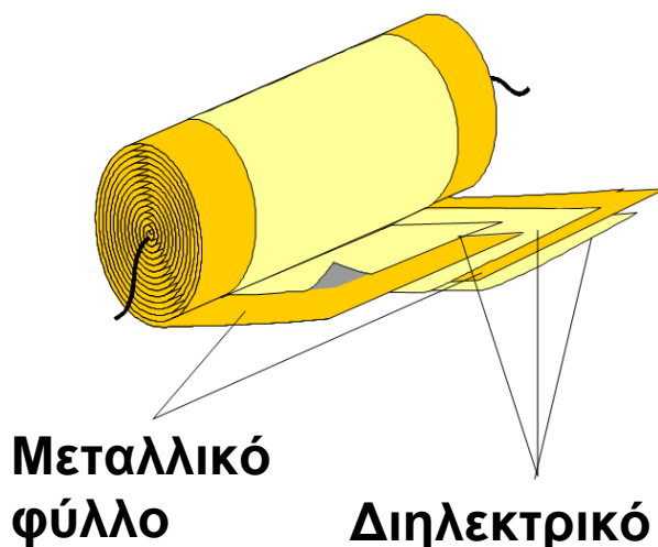
Σχ. 5.40 Πυκνωτής "σάντουιτς". Αποτελείται από δυο μεταλλικά φύλλα που διαχωρίζονται από διηλεκτρικό.
