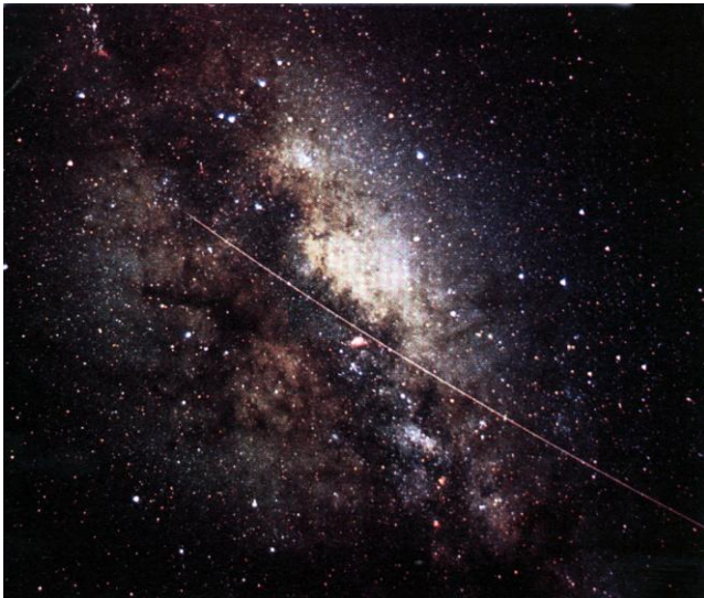
Εικ.5.9 Τμήμα του γαλαξία μας. Η συγκρότηση και η κίνηση των γαλαξιών οφείλεται σε βαρυτικές δυνάμεις. Η φωτεινή γραμμή που φαίνεται στη φωτογραφία είναι η τροχιά ενός μετεωρίτη που διασχίζει τη γήινη ατμόσφαιρα.
