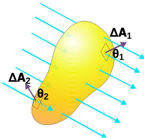
Σχ. 5.6 Κλειστή επιφάνεια μέσα σε ηλεκτρικό πεδίο. Τα κάθετα διανύσματα \Delta\mathbf{A} εξ ορισμού κατευθύνονται προς τα έξω.
