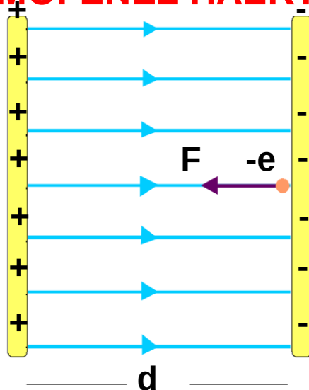
Σχ. 5.25 Ένα ηλεκτρόνιο αφήνεται μέσα σε ομογενές ηλεκτρικό πεδίο.
