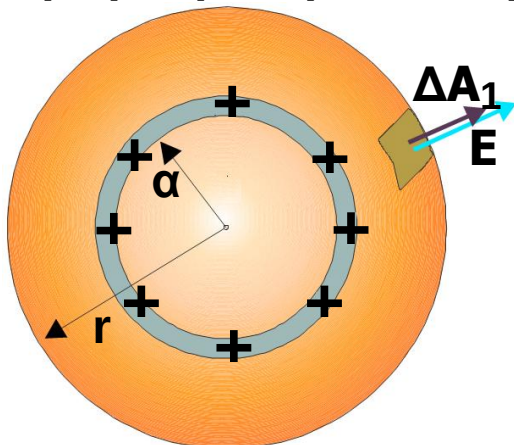
Σχ. 5.11 Η επιφάνεια Gauss είναι σφαίρα ομόκεντρη με το κέλυφος με ακτίνα μεγαλύτερη ή ίση της ακτίνας του κελύφους.
