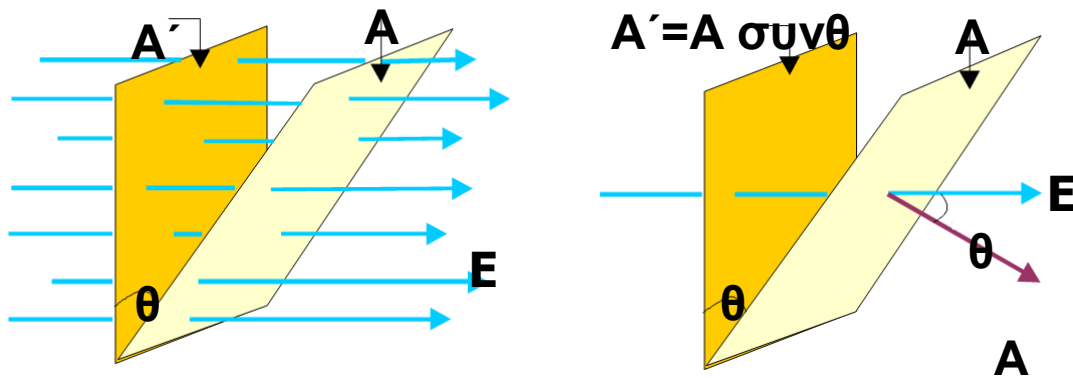
Σχ. 5.4 Από τις επιφάνειες A και A' περνάει η ίδια ηλεκτρική ροή αφού από τις δύο επιφάνειες διέχεται ο ίδιος αριθμός δυναμικών γραμμών.
