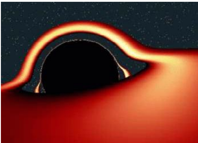
Εικ. 5.13 Προσομοίωση μαύρης τρύπας σε υπολογιστή. Η ύλη έλκεται από μια μαύρη τρύπα σχηματίζοντας γύρω της ένα περιστρεφόμενο δίσκο.
