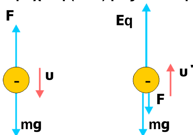
Σχ. 5.62 (α) Οι δυνάμεις στην σταγόνα που πέφτει με την οριακή της ταχύτητα u . (β) Οι δυνάμεις παρουσία του ηλεκτρικού πεδίου.
