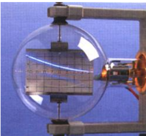
Εικ. 5.2 Πειραματική διάταξη για τη μελέτη της απόκλισης μιας δέσμης ηλεκτρονίων μέσα σε ομογενές ηλεκτρικό πεδίο
