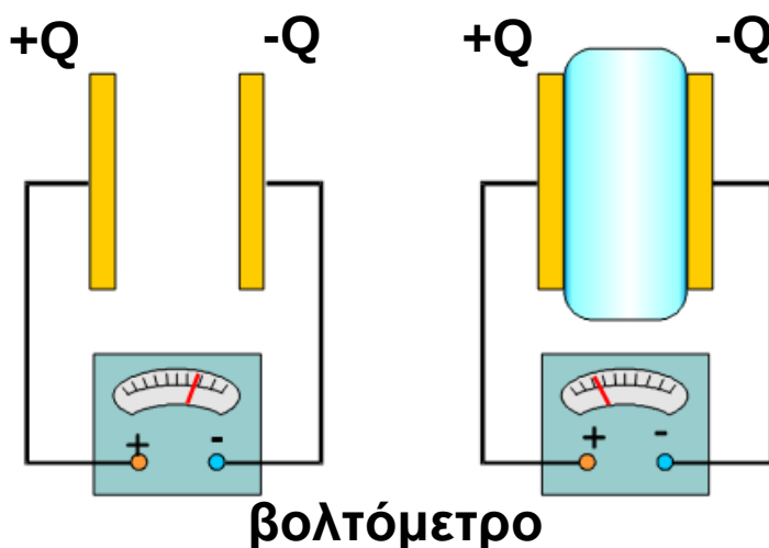
Σχ. 5.41 Εάν τοποθετήσουμε διηλεκτρικό ανάμεσα στους οπλισμούς φορτισμένου πυκνωτή το βολτόμετρο δείχνει ότι η διαφορά δυναμικού μειώνεται.
