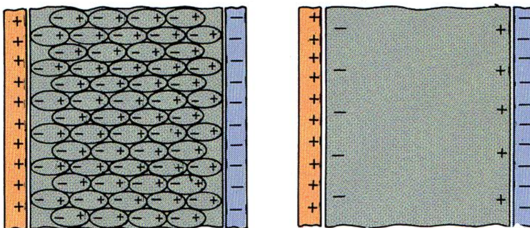
Σχ. 5.44 Το διηλεκτρικό μέσα στο ομογενές πεδίο του πυκνωτή πολώνεται. Τα επαγόμενα φορτία στις επιφάνειες του διηλεκτρικού ελαττώνουν το ηλεκτρικό πεδίο στο εσωτερικό του πυκνωτή.
