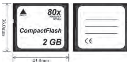
Εικόνα 100: Compactflash
