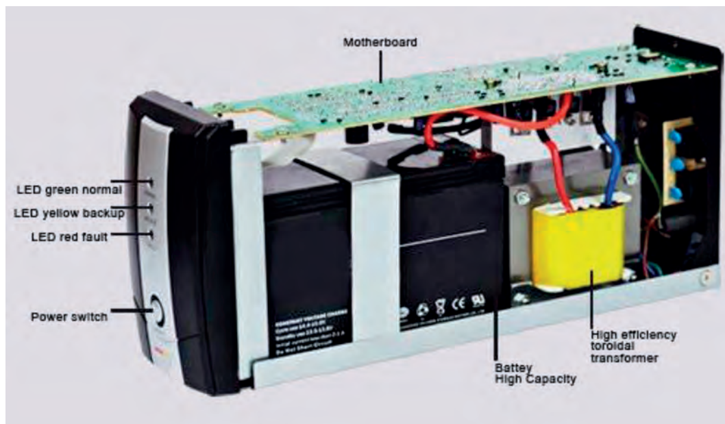
Εικόνα 86: Εσωτερικό ενός UPS
