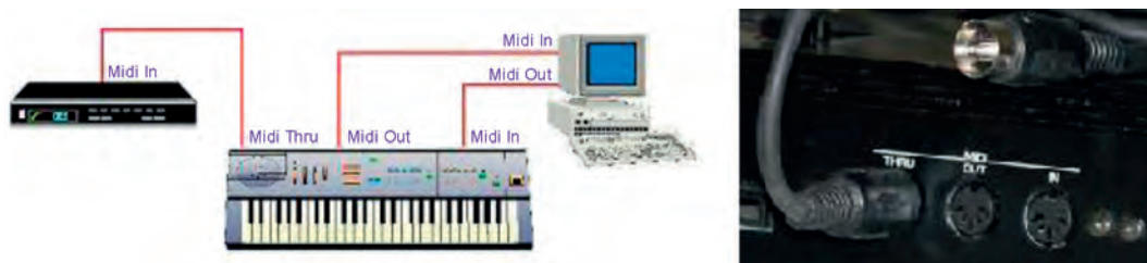
Εικόνα 95: Υποδοχές
