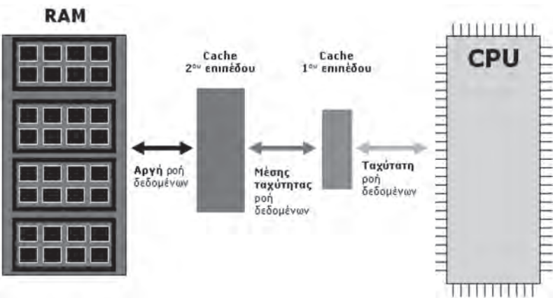
Εικόνα 22: Cache
