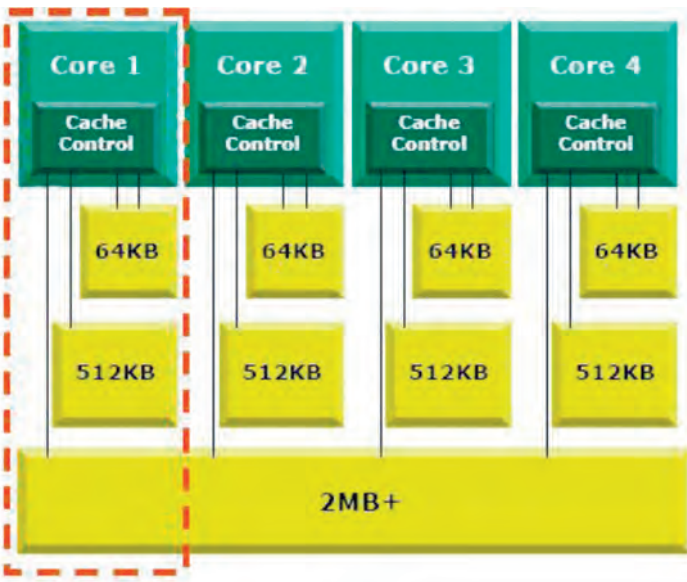
Εικόνα 23: Cache
