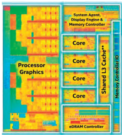
Εικόνα 19: Πυρήνες Επεξεργαστή
