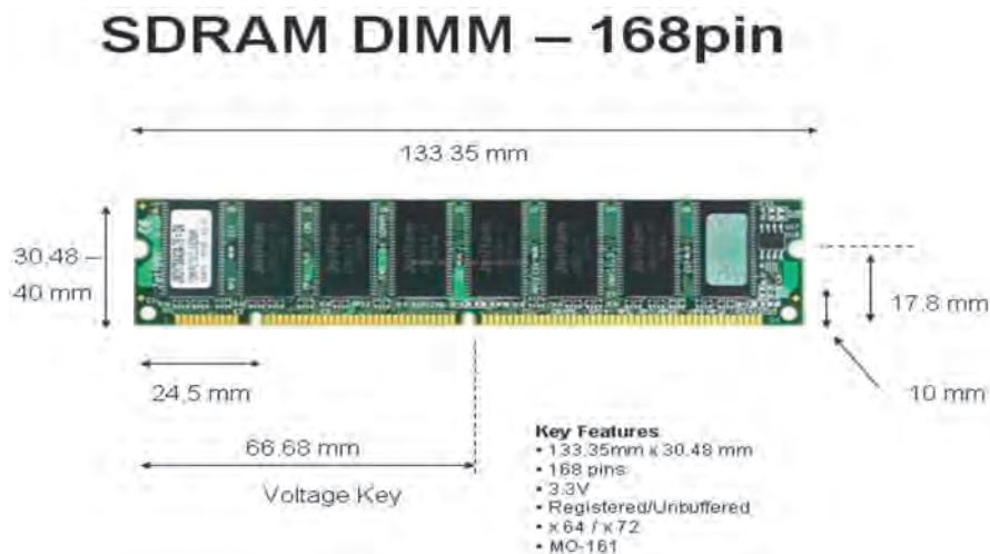
Εικόνα 26: SDRAMDIMM
