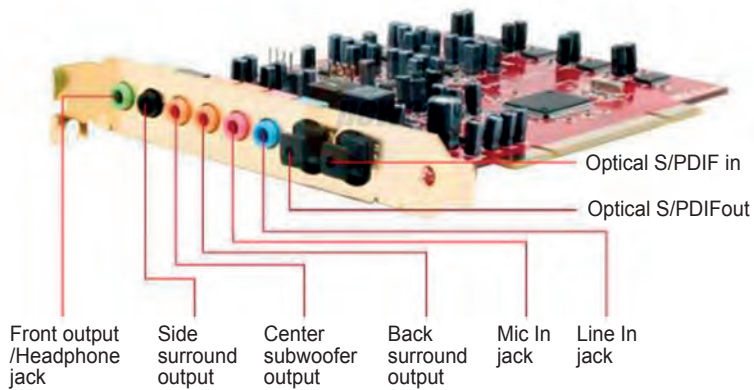
Εικόνα 91: Κάρτα ήχου
