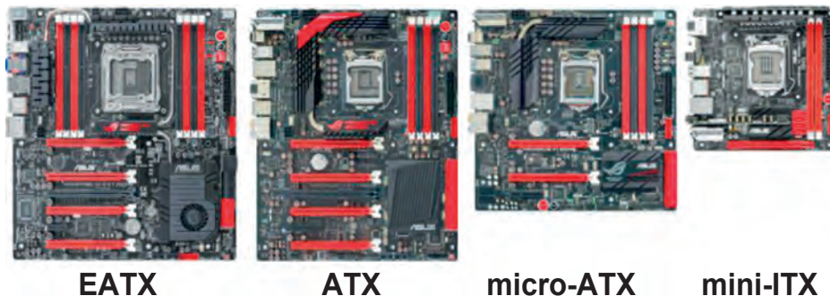
Εικόνα 8: Μητρικές πλακέτες
