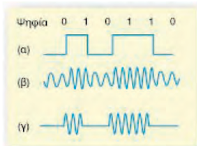
Σχ. 2.6. Απλά παραδείγματα ASK διαμόρφωσης.
