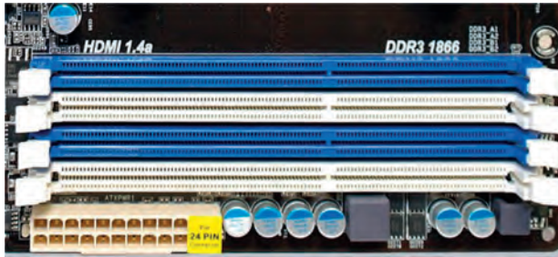
Εικ. 1.13. Υποδοχές για αρθρώματα μνήμης RAM (RAM memory slots) τύπου DDR3.
