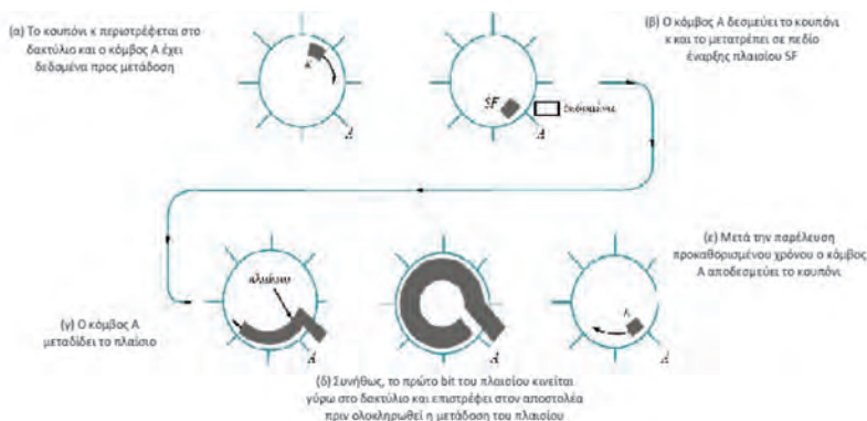
Σχ. 4.11. Σχηματική αναπαράσταση τρόπου λειτουργίας του δικτύου IEEE 802.5
