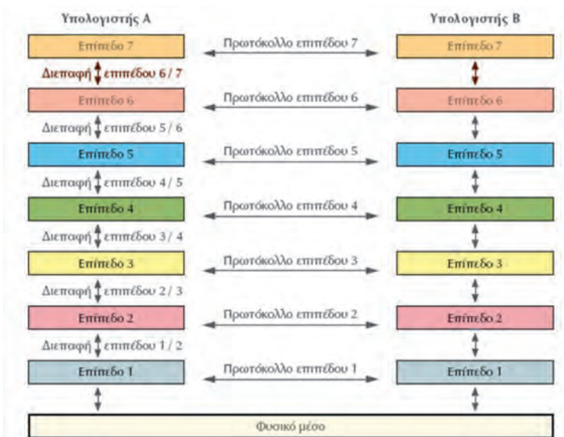
Σχ.3.3. Σχηματική αναπαράσταση αρχιτεκτονικής επιπέδων.
