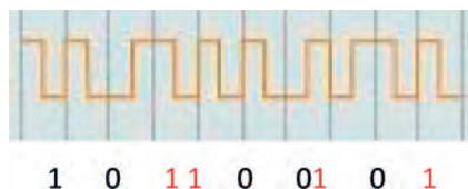
Σχ. 2.10. Διαφορική Κωδικοποίηση Manchester.
