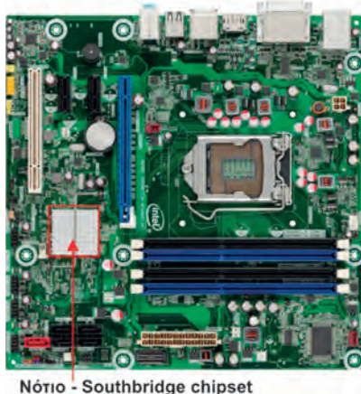
Εικ. 1.12: Μητρική πλακέτα για σύγχρονους επεξεργαστές που ενσωματώνουν το northbridge chip.
