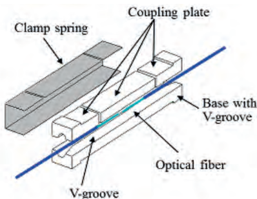
Σχ. 5.5. Μηχανική Σύνδεση Οπτικής Ίνας
