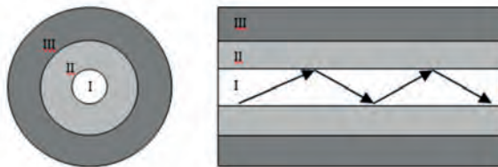
Σχ. 5.3. Δομή Οπτικής Ίνας
