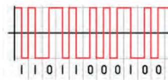
Σ.χ. 2.9. Βασική Κωδικοποίηση Manchester.
