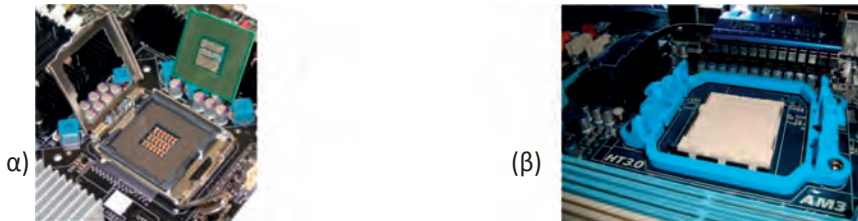
Εικ. 1.10.(α) Socket επεξεργαστών της Intel, (β) Socket επεξεργαστών της AMD
