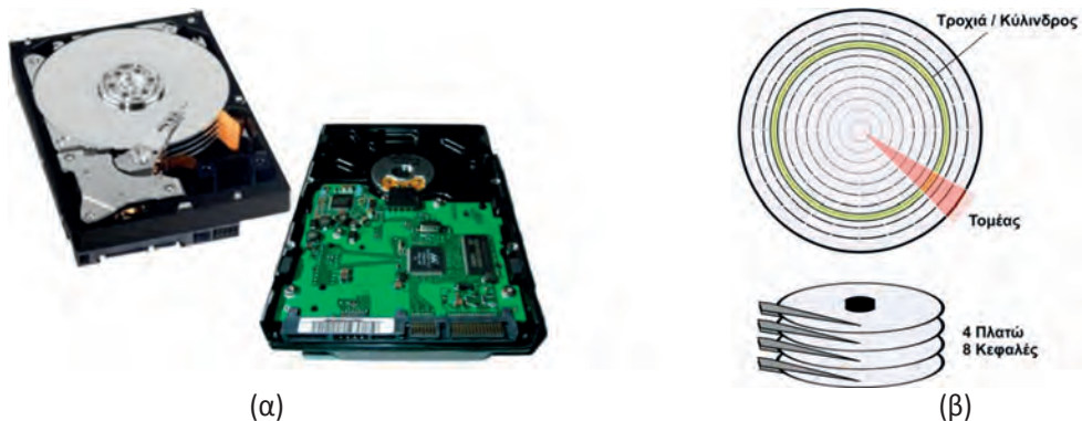
Εικ.1.20 : (α) Το εσωτερικό ενός σκληρού δίσκου, (β) Λογική οργάνωση ενός «πλαττώ».
