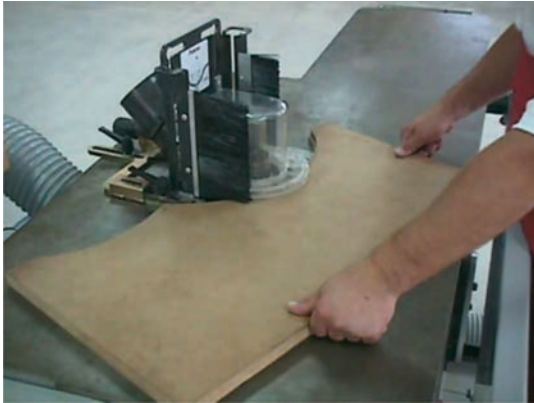
Εικ. 8.9 Μορφοποίηση καμπύλων επιφανειών με τη βοήθεια οδηγού δακτυλίου σε σβούρα.
