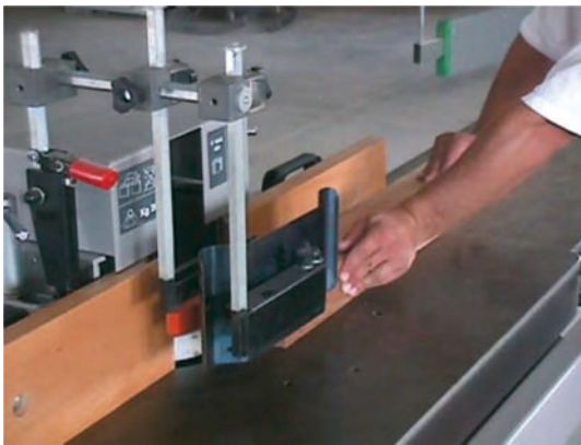
Εικ. 8.7 Κατά μήκος κατεργασία ξυλοτεμαχίου.
