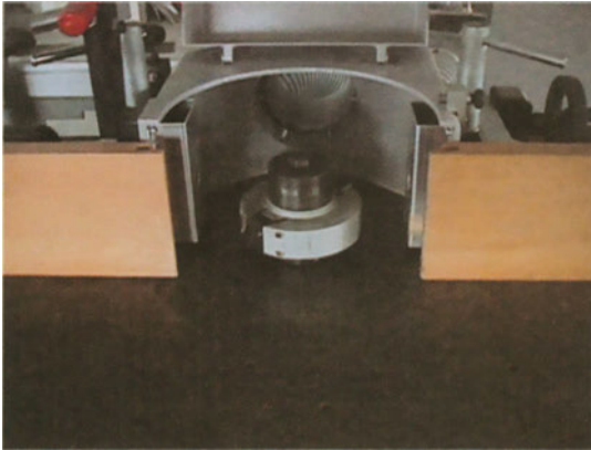
Εικ. 8.4 Κοπτικό που προεξέχει ολόκληρο πάνω από την τράπεζα εργασίας.
