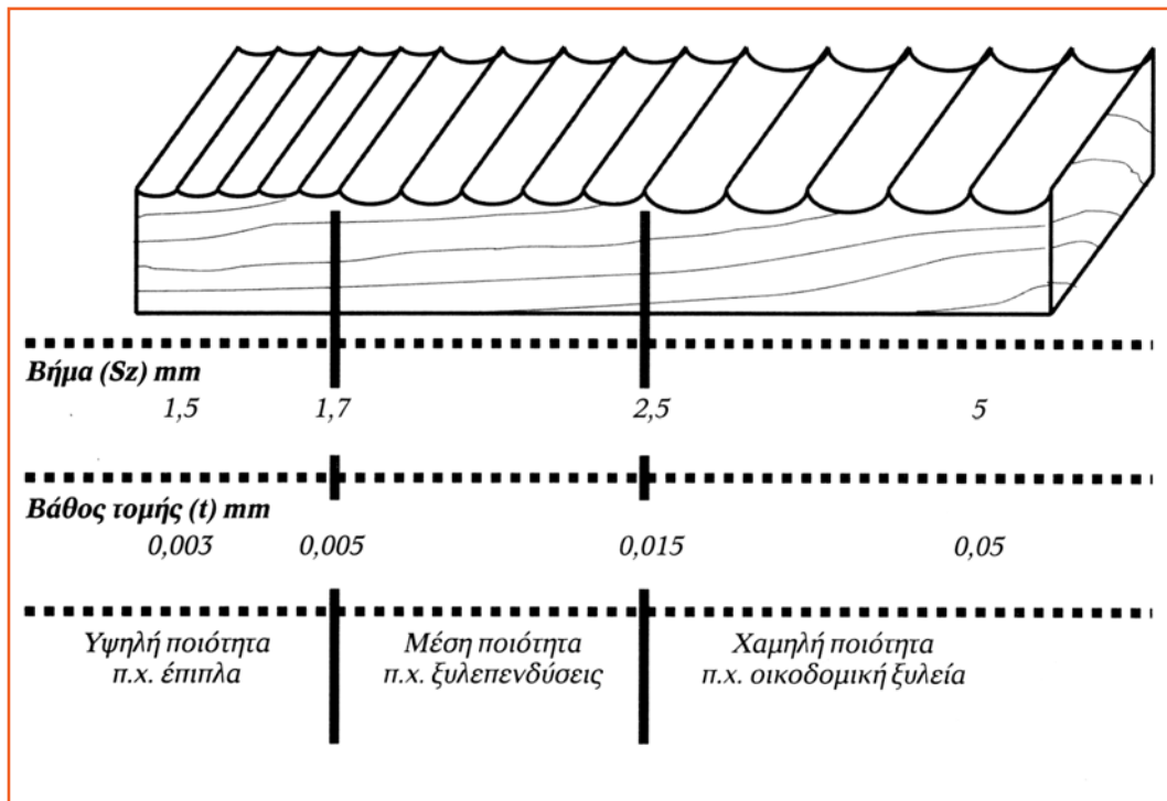
Σχ. 6.2 Σχέση βήματος ( S_z ) και βάθους τομής ( t ) με την ποιότητα πλάνισματος.
