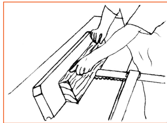
Σχ. 6.5 Λοξό πλάνισμα πριστοτεμαχίου.
