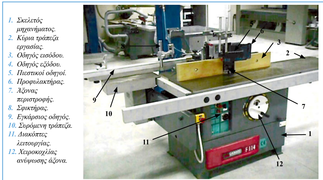
Εικ. 8.1 Τα κύρια στοιχεία της σβούρας.
