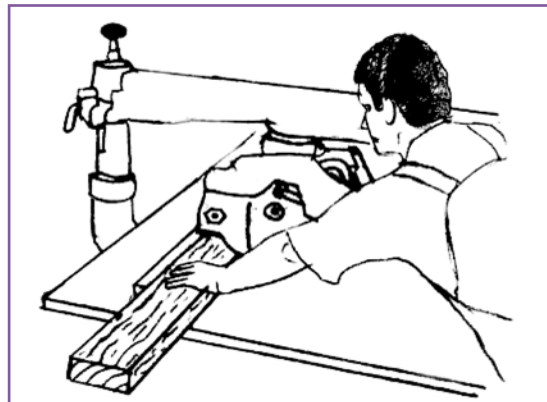
Σχ. 4.9 Δημιουργία πατούρας.
