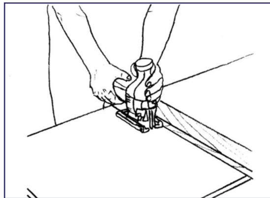
Σχ. 5.8 Πρίση ξύλου μεγάλου πλάτους.
