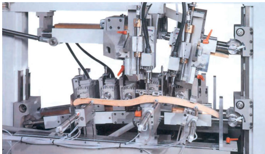
Εικ. 11.3 Η περιοχή κατεργασίας του αυτόματου μορσοτρύπανου.
