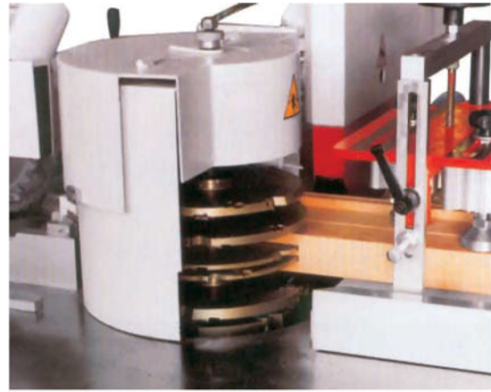
Εικ. 16.8 Δημιουργία μόρσων στην εγκάρσια επιφάνεια ξυλοτεμαχίου.
