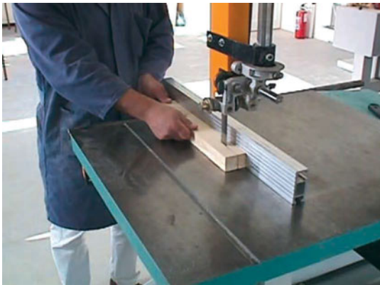
Εικ. 1.1 Πρίση με ταινιοπρίονο.
