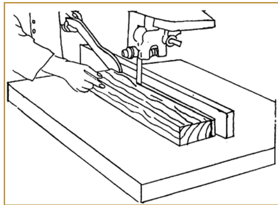
Σχ. 3.7 Τελική προώθηση ξυλοτεμαχίου με προωθητήρα.
