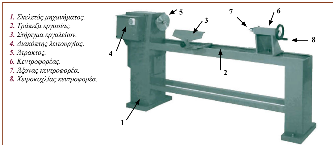
Εικ. 10.1 Τα κύρια στοιχεία του απλού τόννου.
