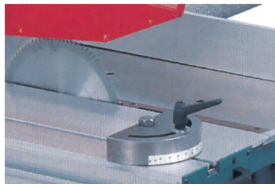
Εικ. 4.3 Εγκάρσιος οδηγός στο επιτραπέζιο δισκοπρίονο.
