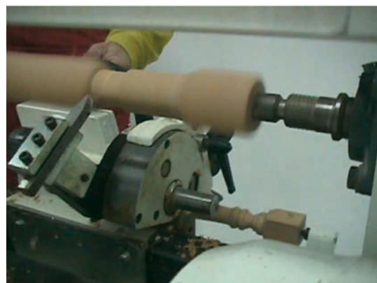
Εικ. 10.8 Τórνευση ξύλου με το σταθερό μαχαίρι.
