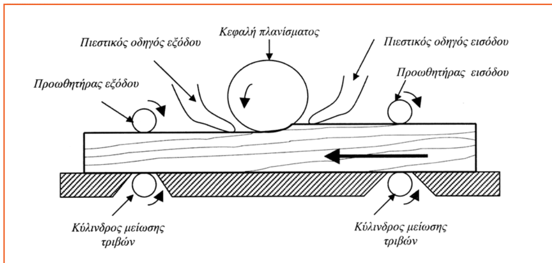
Σχ. 6.6 Σχηματική παράσταση στοιχείων ξεchonδριστήρα.
