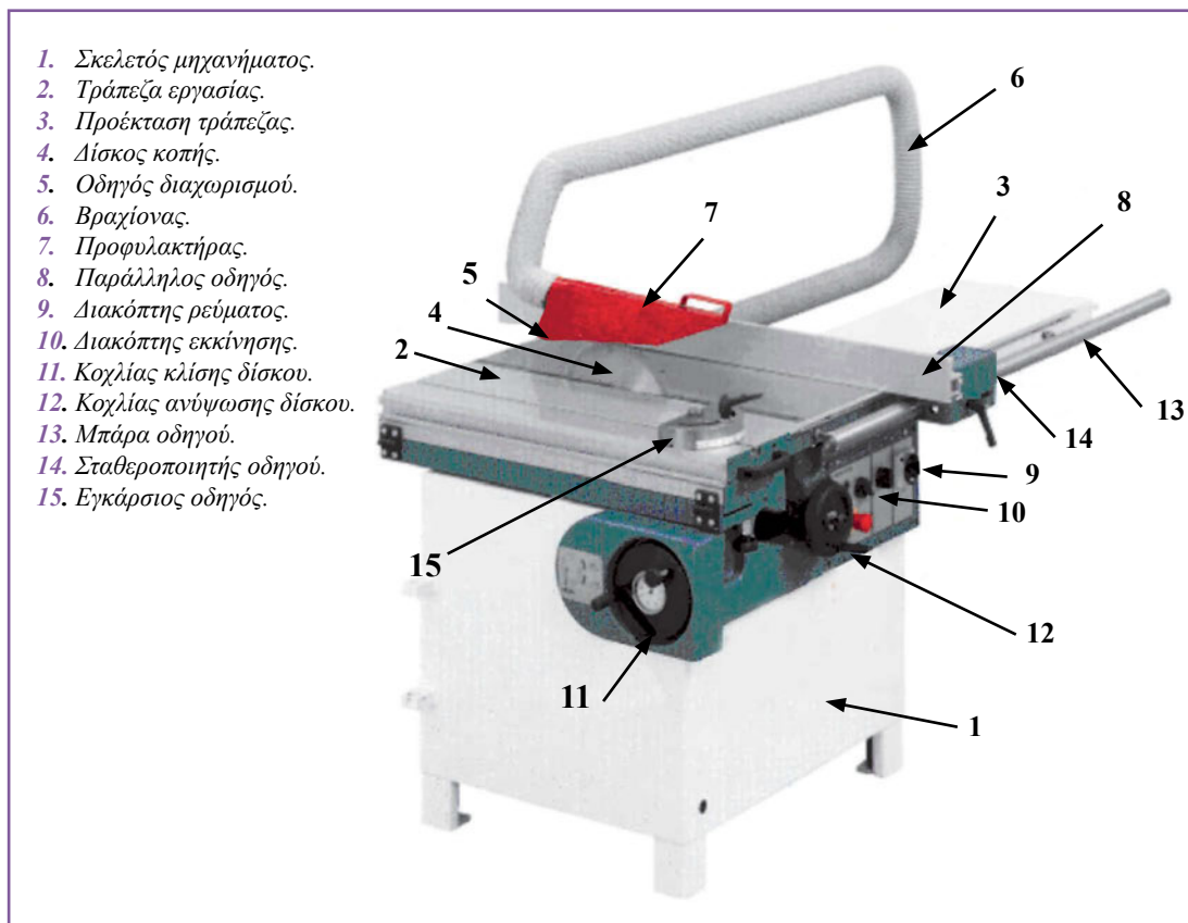
Εικ. 4.2 Επιτραπέζιο δισκοπρίονο.
