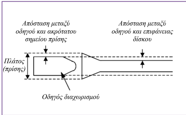
Σχ. 4.2 Ο οδηγός διαχωρισμού σε σχέση με το πλάτος πρίσης και το πάχος του σώματος του δίσκου.
