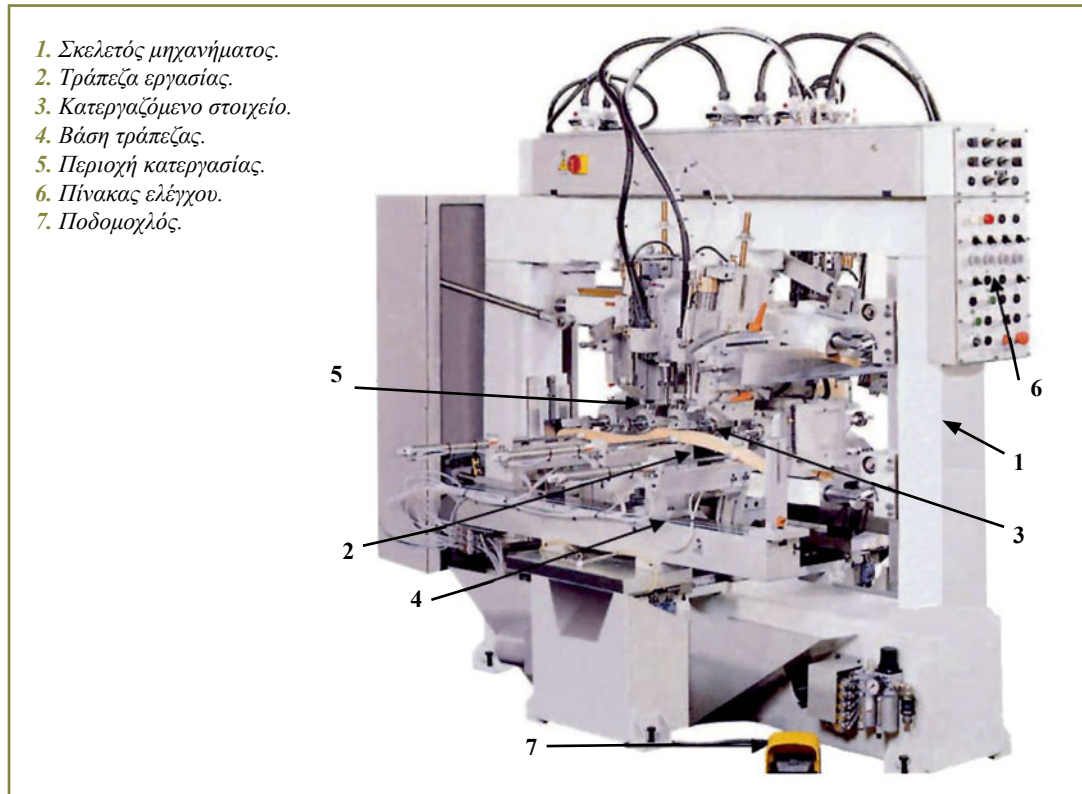
Εικ. 11.2 Τα κύρια μέρη του αυτόματου μορσοτρύπανου.
