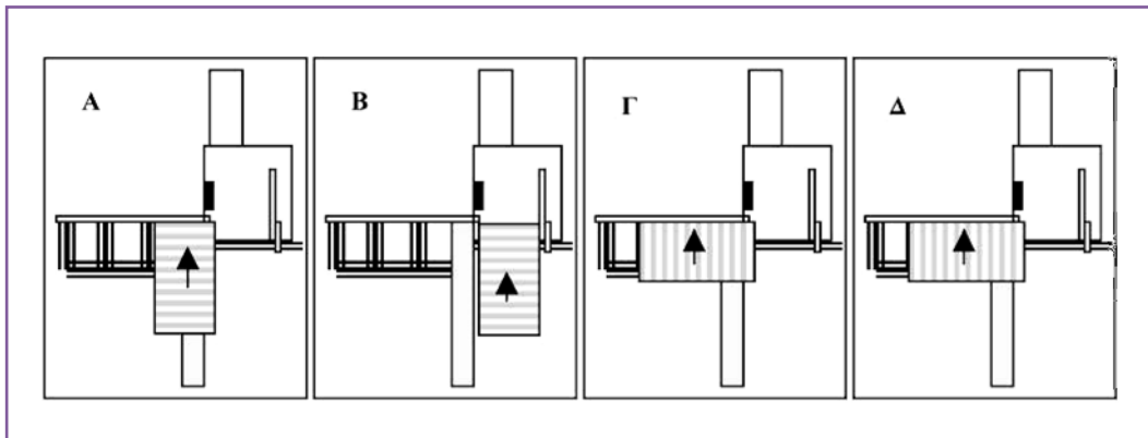
Σχ. 4.10 Στάδια τεμαχισμού ξυλοπλάκας με το δισκοπρίονο τεμαχισμού.
