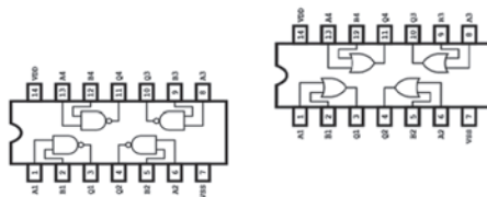
Ολοκληρωμένα κυκλώματα με 4 πύλες
