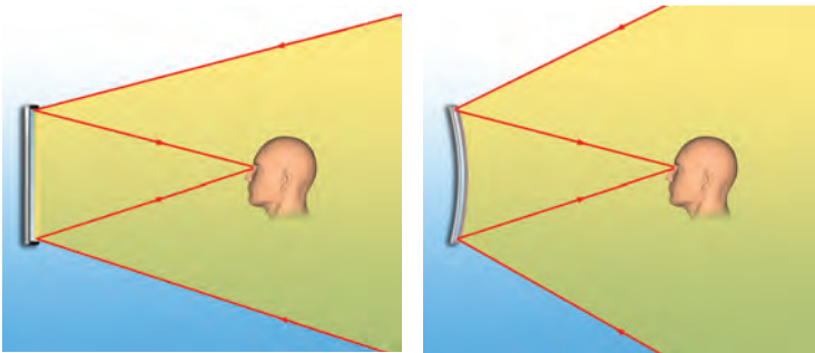
Εικόνα 7.14 ◀ Οπτικό πεδίο επίπεδου και κυρτού σφαιρικού καθρέφτη.
