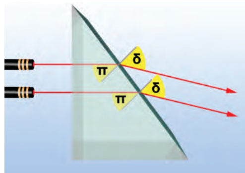
Εικόνα 8.18 Οι μονοχρωματικές φωτεινές δέσμες παραμένουν παράλληλες μετά την έξοδό τους από το πρίσμα.
