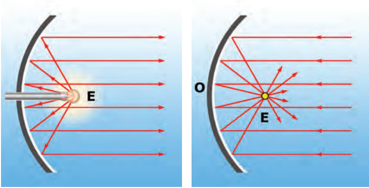
Εικόνα 7.13 ◀ Η αντίστροφη πορεία του φωτός Η αντίστροφη πορεία του φωτός σε έναν κοίλο καθρέφτη.
