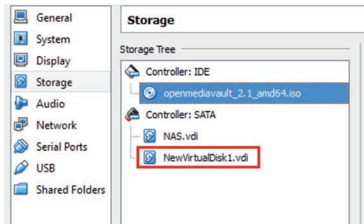
Εικόνα 6.12: Η εικονική μηχανή με δύο εικονικούς δίσκους
