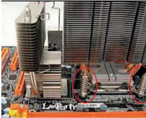
Εικόνα 2.3: Ψύκτρα με μηχανισμό στήριξης
