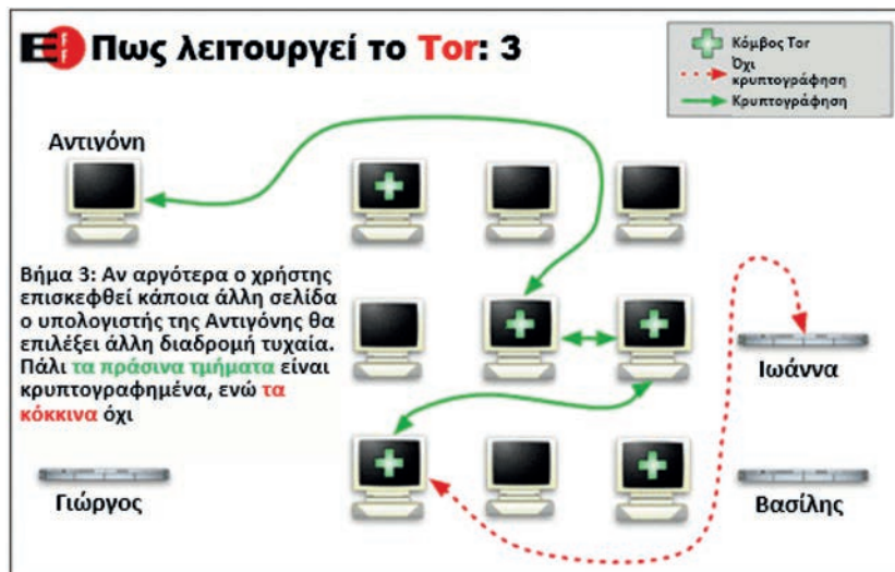
Εικόνα 8.22: Λειτουργία του Tor (βήμα 3).
