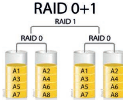
Εικόνα 3.3. Συστοιχία RAID 0+1.
