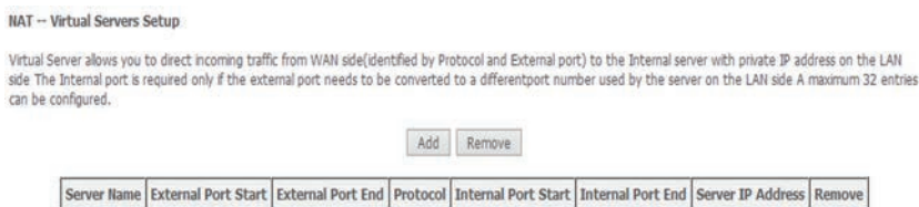
Εικόνα 7.50: Προώθηση θύρας
