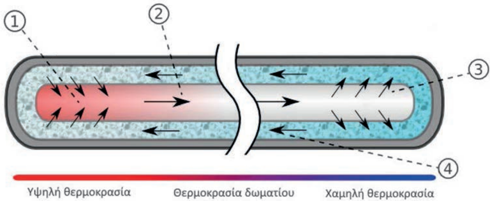
Εικόνα 2.8: Αρχή λειτουργίας θερμοαγωγού (Πηγή: https://en.wikipedia.org/wiki/Heat_pipe )
