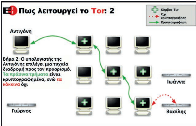
Εικόνα 8.21: Λειτουργία του Tor (βήμα 2).
