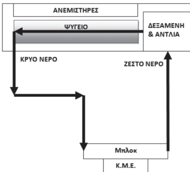
Εικόνα 2.6: Βασική λειτουργία υδρόψυξης
