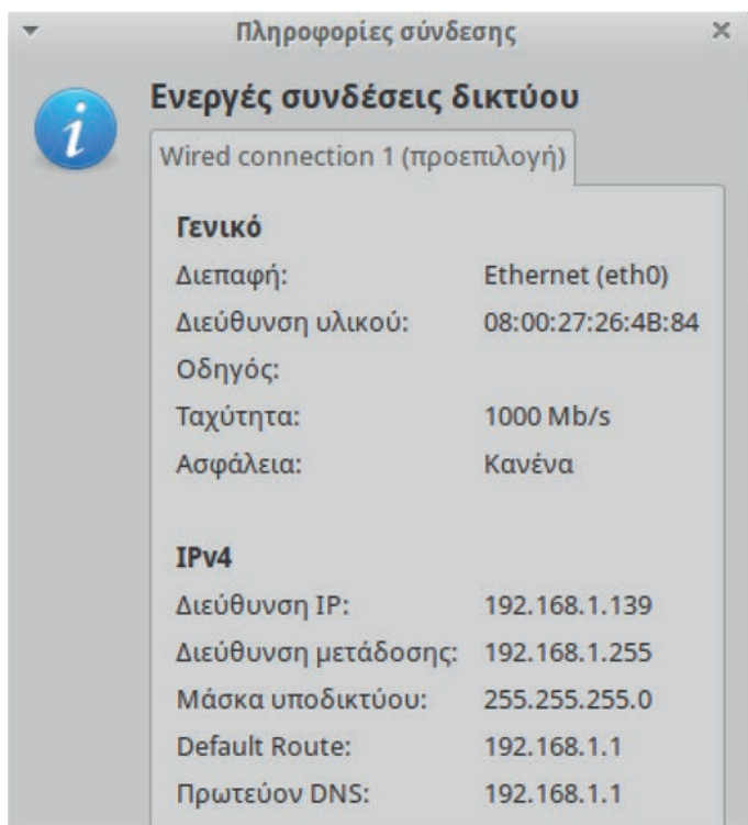
Εικόνα 5.7: Πληροφορίες κάρτας δικτύου
