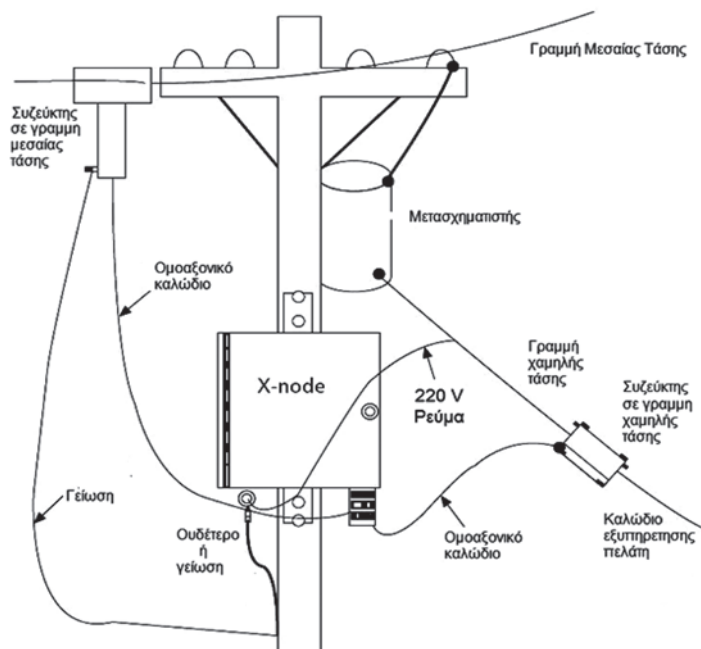
Σχήμα 11.1: Τρόπος εγκατάστασης τεχνολογίας Powerline
