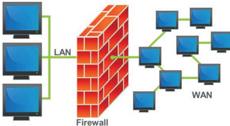
Εικόνα 8.13: Τείχος Προστασίας.
