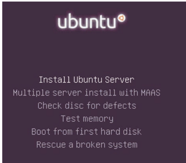
Εικόνα 7.11: Έναρξη εγκατάστασης
