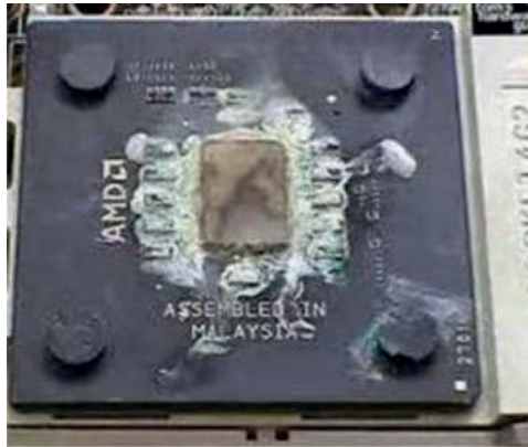
Εικόνα 2.1: Κατεστραμμένη Κ.Μ.Ε., λόγω υπερθέρμανσης
