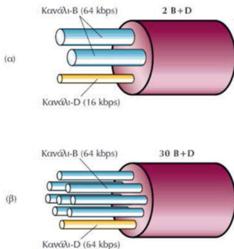
Σχήμα 5.1.3.α. Διεπαφή βασικού ρυθμού BRA (α) και Διεπαφή πρωτεύοντος ρυθμού PRI (β)
