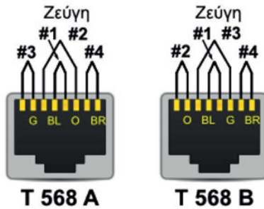
Εικόνα 2.4.1.α: Συρμάτωση
