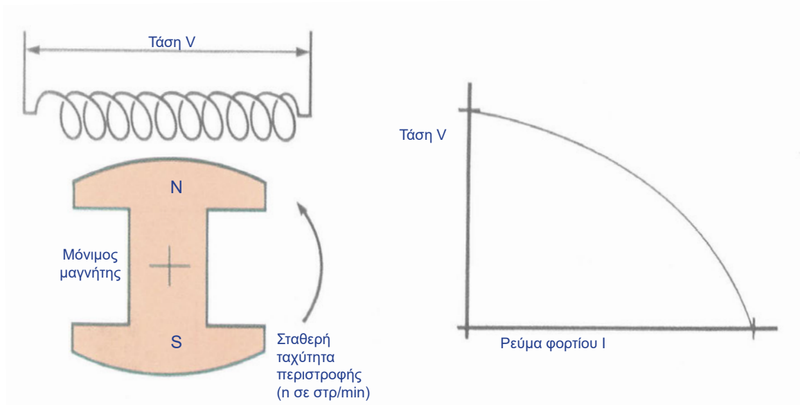
Σχήμα 5.1: Γεννήτρια με διέγερση μόνιμου μαγνήτη και η χαρακτηριστική φορτίου της
