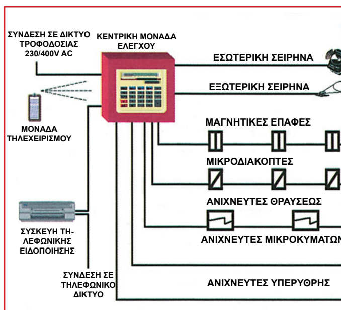
Σχήμα 6.4 : Συνδεσμολογία κεντρικής μονάδας ελέγχου
