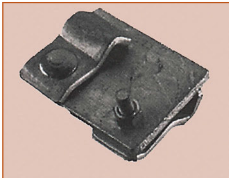
Σχήμα 4.12: Σύνδεσμος σπλισμού
