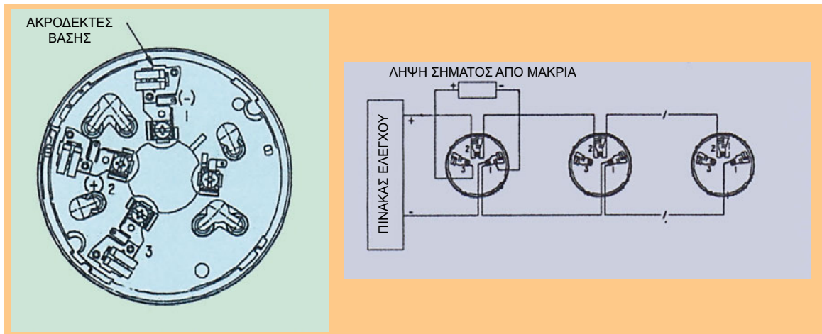
Εικόνα 1.5: Βάση πυρανιχνευτή και σύνδεση πυρανιχνευτών
