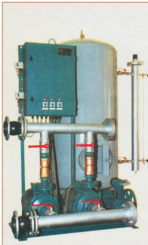
Εικόνα 8.4: Πιεστικό συγκρότημα
