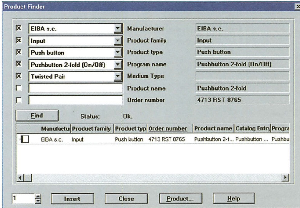
Σχήμα 4.7: Παράμετροι συσκευών
