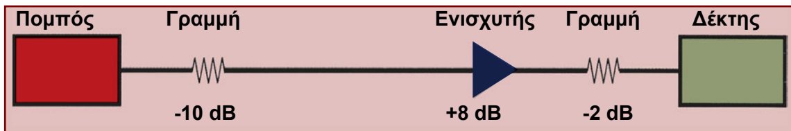
Σχήμα 3.1: Παράδειγμα χρήσης ενισχυτών και αποσβέσεων.
