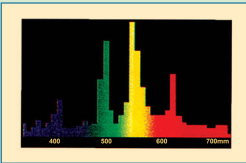
Σχήμα 3.35: Φασματική κατανομή λαμπτήρα ατμών υδραργύρου, βελτιωμένου φάσματος
