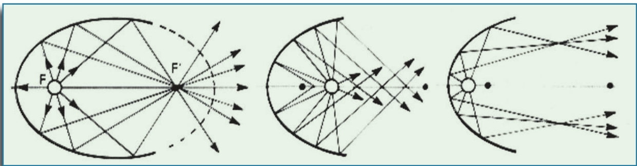
Σχήμα 1.3: Αποκλίνουσα, παράλληλη, συγκλίνουσα φωτεινή δέσμη
