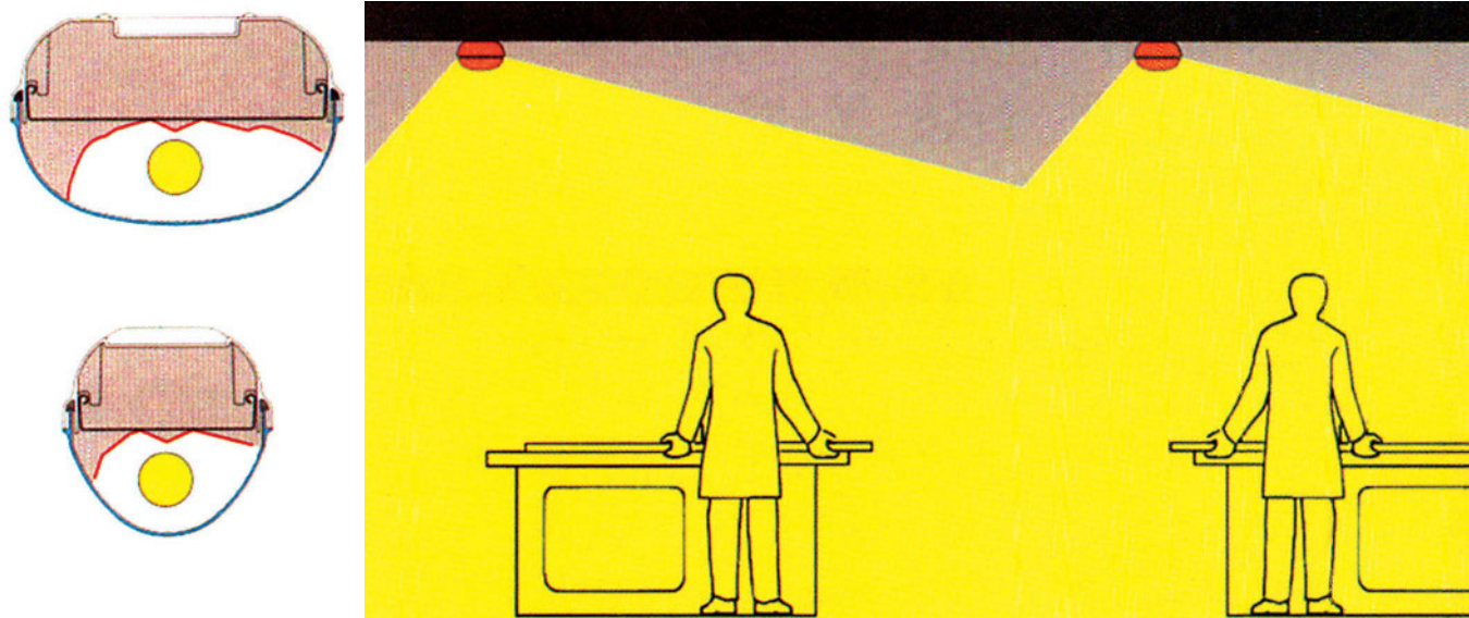
Σχήμα 4.13: Κατανομή φωτός με ανταυγαστήρα ασύμμετρης δέσμης
