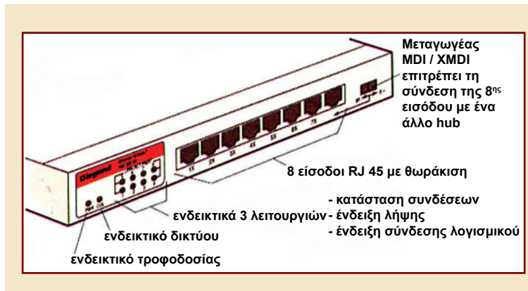
Σχήμα 1.12: Συγκεντρωτής (hub).
