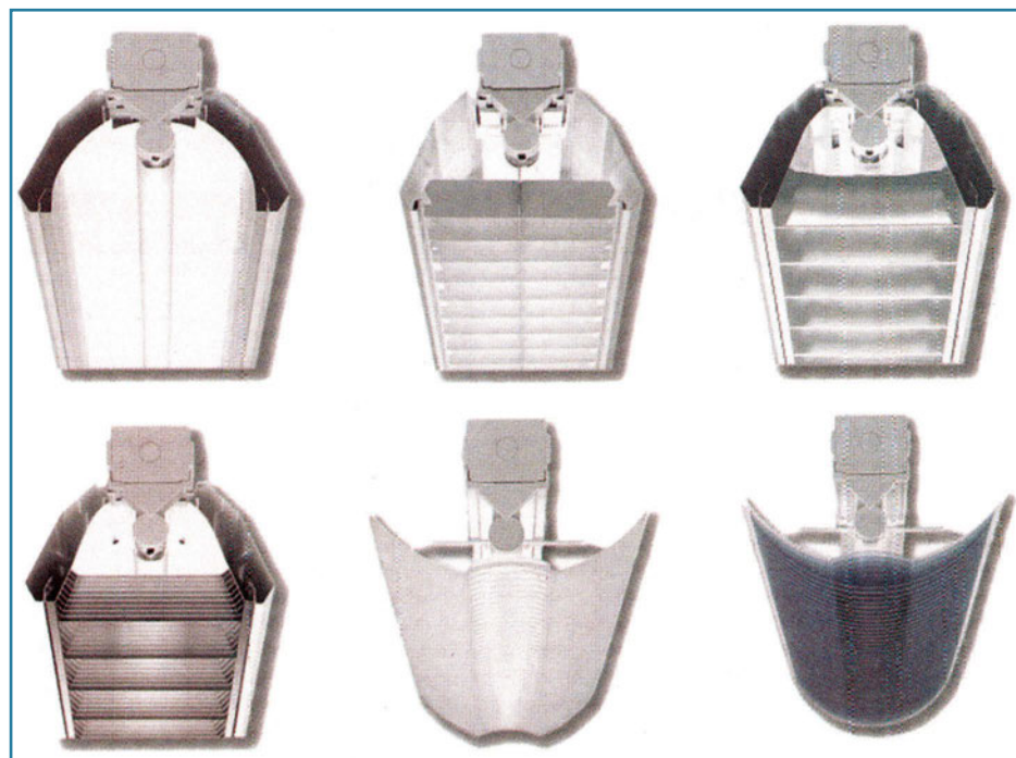
Σχήμα 4.14: Τύποι ανταυγαστήρων
