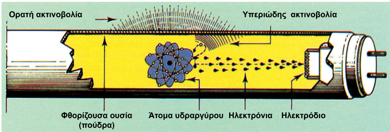
Σχήμα 3.19: Το εσωτερικό του λαμπτήρα φθορισμού.
