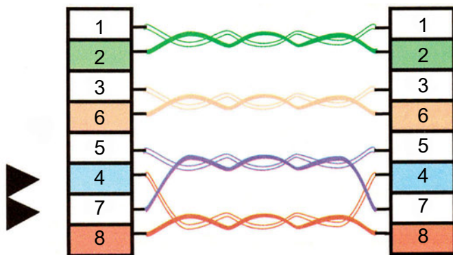
Σχήμα 4.3: Το λάθος της διασταύρωσης ζευγαριού.
