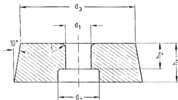
Σχήμα 14.25: Τυποποιημένη μήτρα κοίλανσης
