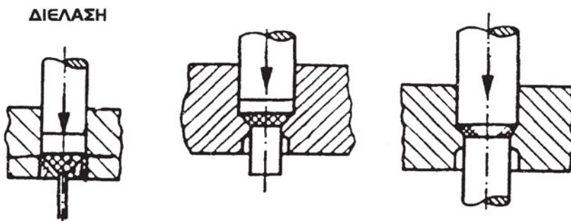
Σχήμα 12.14: Διέλαση ή Εξώθηση
