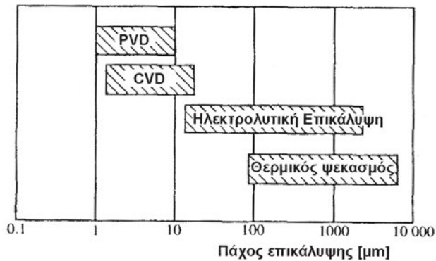
Σχήμα 17.7: Μεταβολή του πάχους επικάλυψης για διάφορες κατεργασίες με απόθεση υλικού
