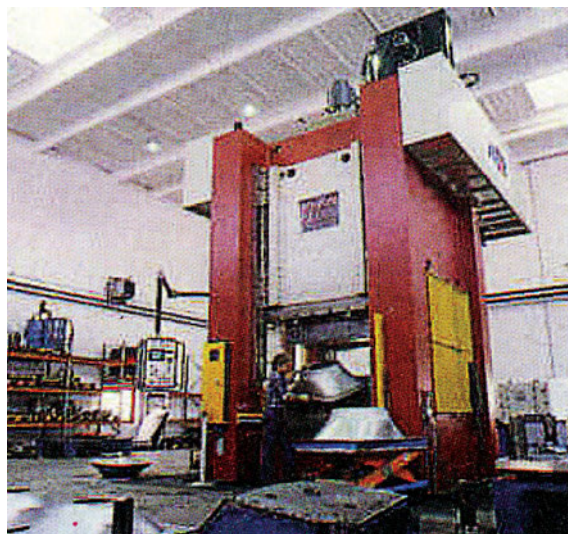
Σχήμα 14.18: Πρέσα που πραγματοποιεί κοίλανση
