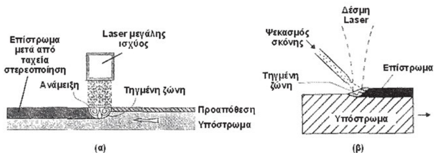
Σχήμα 18.9: Τεχνικές επικάλυψης με δέσμη laser: (α) με προαπόθεση σκόνης και (β) με ταυτόχρονο ψεκασμό σκόνης
