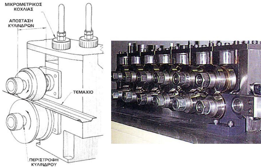
Σχήμα 13.22: Έλαστρα με μία και διαδοχικές θέσεις παραμόρφωσης
