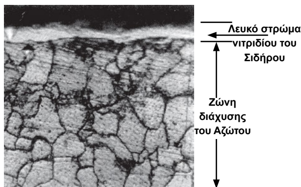
Σχήμα 5.12: Οπτική μικρογραφία εναζωτώμενου χάλυβα. Διακρίνεται η λευκή επιφανειακή στιβάδα, η οποία αποτελείται αποκλειστικά από νιτρίδιο του σιδήρου, ενώ και η υποκείμενη ζώνη είναι εμπλουτισμένη με άζωτο (μεγέθυνση X600).
