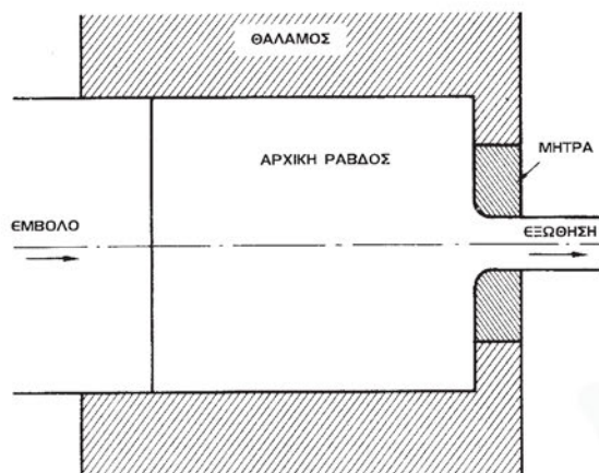
Σχήμα 13.32: Άμεση εξώθηση
