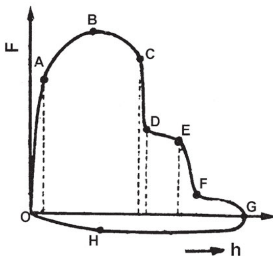
Σχήμα 14.7: Κύκλος απότμησης
