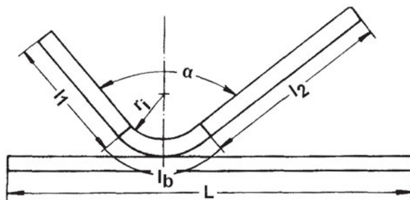
Σχήμα 14.35: Ανάπτυγμα ελάσματος
