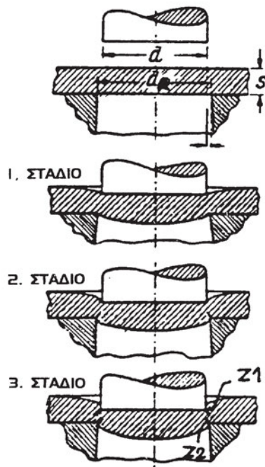
Σχήμα 14.5: Στάδια απότμησης
