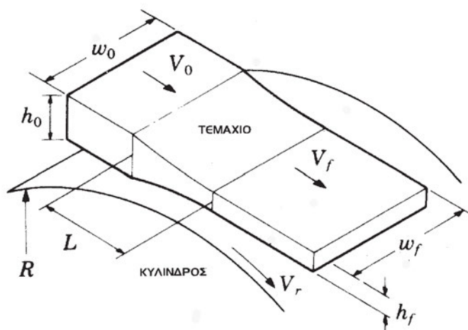
Σχήμα 13.14: Επίπεδη έλαση
