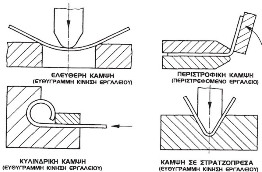
Σχήμα 14.40: Είδη κάμψης I
