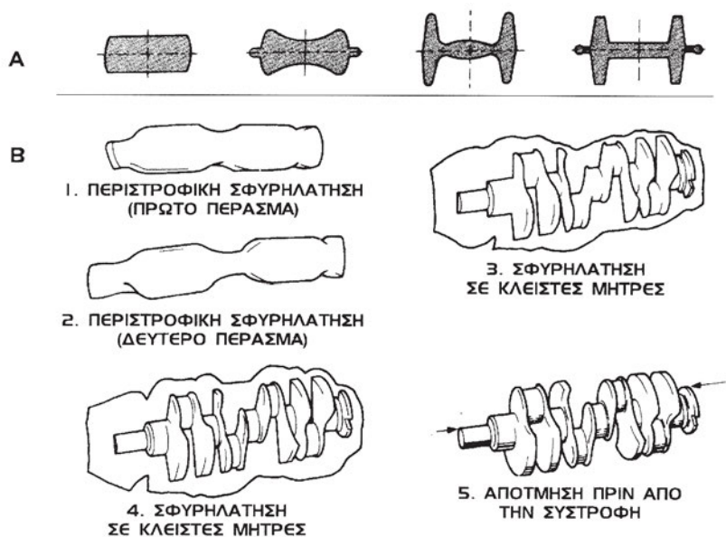
Σχήμα 13.8: Σφυρηλάτηση δοκού τυπτοποιημένης διατομής Η και στροφαλοφόρου άξονα ΜΕΚ
