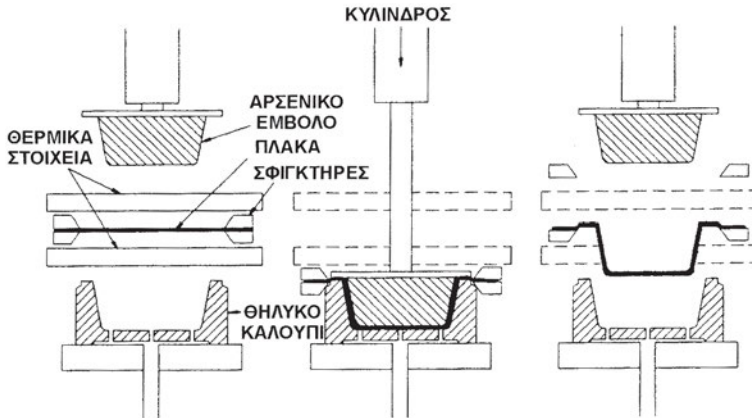
Σχήμα 15.17: Θερμοδιαμόρφωση
