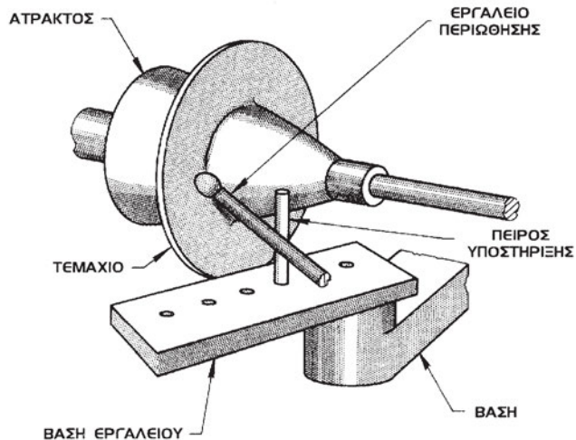
Σχήμα 14.47: Εξοπλισμός περιώθησης
