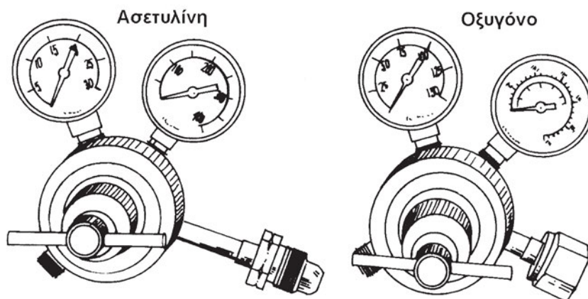
Σχήμα 16.4: Μανοεκτονωτές
