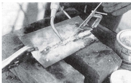
Σχήμα 16.27: Μπρουντζοκόλληση
