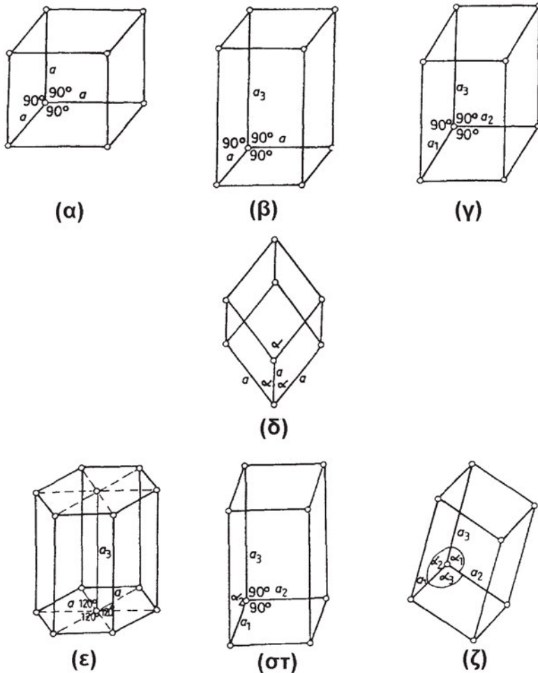
Σχήμα 2.4: Τα επτά βασικά κρυσταλλικά συστήματα: (α) κυβικό, (β) τετραγωνικό, (γ) ορθορομβικό, (δ) ρομβοεδρικό, (ε) εξαγωνικό, (στ) μονοκλινές και (ζ) τρικλινές.
