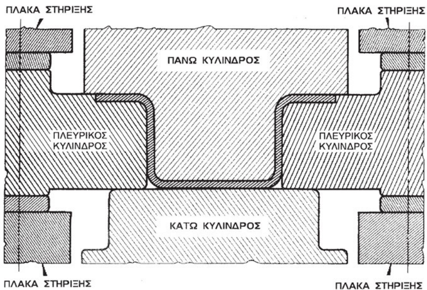
Σχήμα 13.23: Κύλινδροι υποστήριξης
