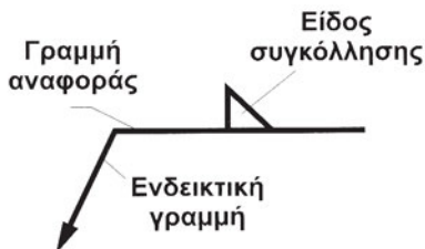
Σχήμα 16.1: Σύμβολο συγκόλλησης
