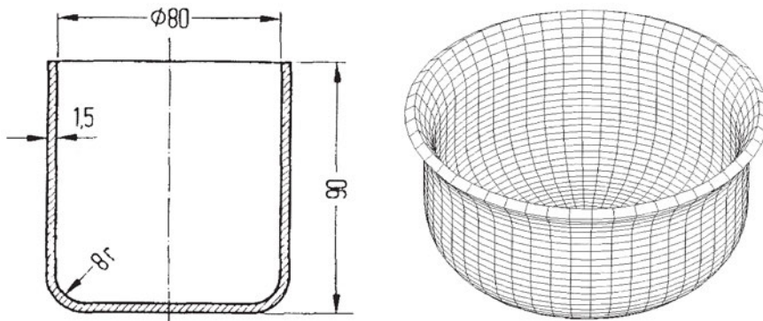
Σχήμα 14.28: Εφαρμογή στην κοίλανση
