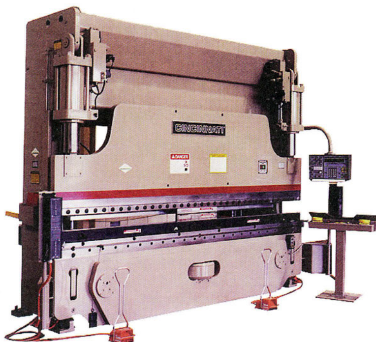
Σχήμα 14.30: C.N.C. Στραντζόπρεσα
