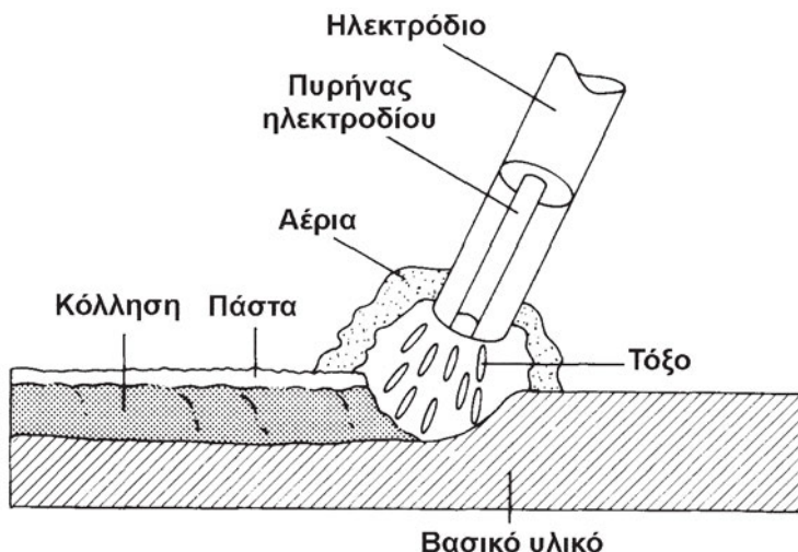
Σχήμα 16.13: Διαδικασία ηλεκτροσυγκόλλησης
