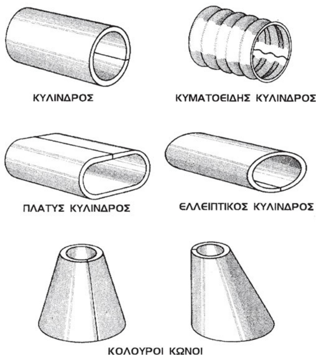
Σχήμα 13.19: Παραδείγματα αντικειμένων που παράγονται από περιστροφική έλαση
