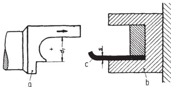
Σχήμα 14.38: Κυλινδρική κάμψη
