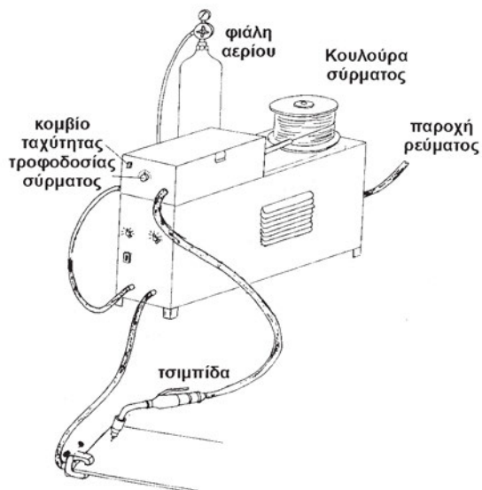
Σχήμα 16.18: Διάταξη συγκόλλησης M.A.G.
