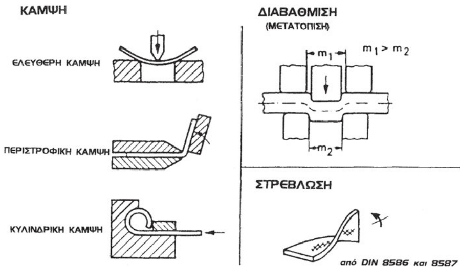
Σχήμα 12.9: Κάμψη, διαβάθμιση, στρέβλωση
