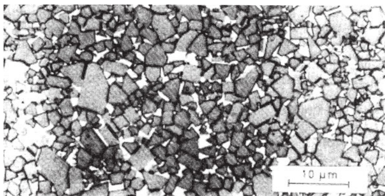
Σχήμα 8.4: Μικροδομή κεραμικού εργαλείου που αποτελείται από WC μέσα σε μήτρα κοβαλτίου ( Co ).
