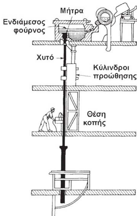
Σχήμα 10.16: Συνεχής χύτευση
