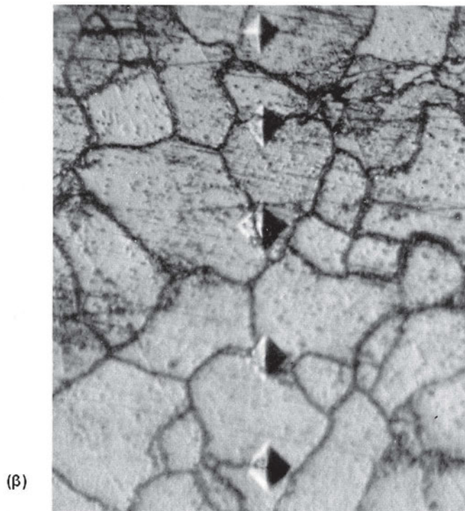
Σχήμα 3.1: (α) Μορφή αποτυπώματος κατά τη σκληρομέτρηση Vickers. (β) Οπτική μικρογραφία διαδοχικών μικροσκληρομετρήσεων σε μαλακό χάλυβα (μεγέθυνση X400).
