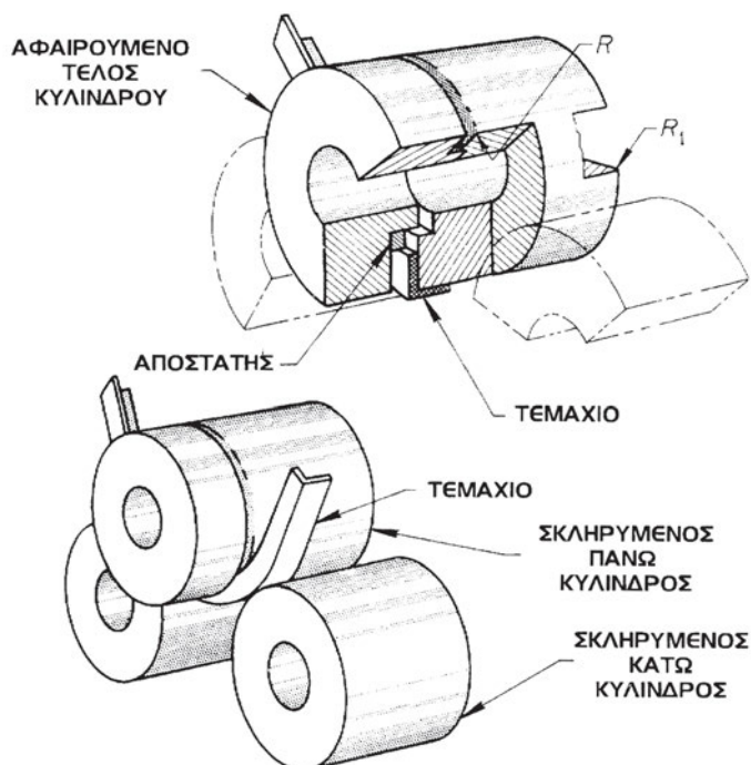
Σχήμα 13.20: Έλαση δοκού τύπου L
