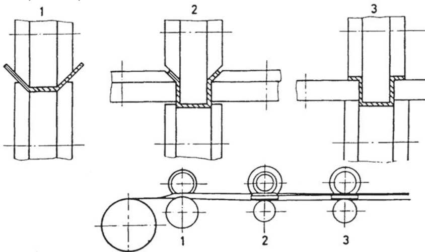
Σχήμα 14.42: Κάμψη μορφής με περιστρεφόμενα εργαλεία
