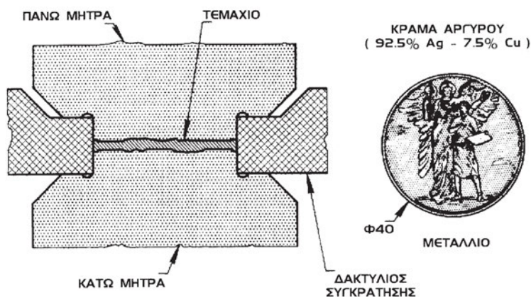
Σχήμα 15.2: Διαμόρφωση μεταλλίων
