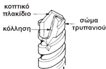
Σχήμα 16.27: Μπρουντζοκόλληση
