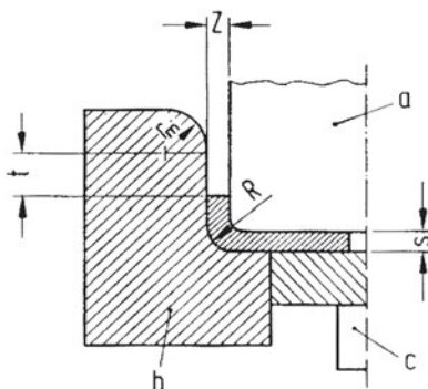
Σχήμα 14.44: Εργαλείο κάμψης U
