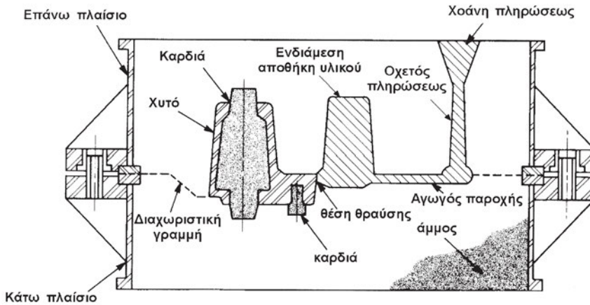
Σχήμα 10.2: Τομή καλουπιού για χύτευση σε άμμο
