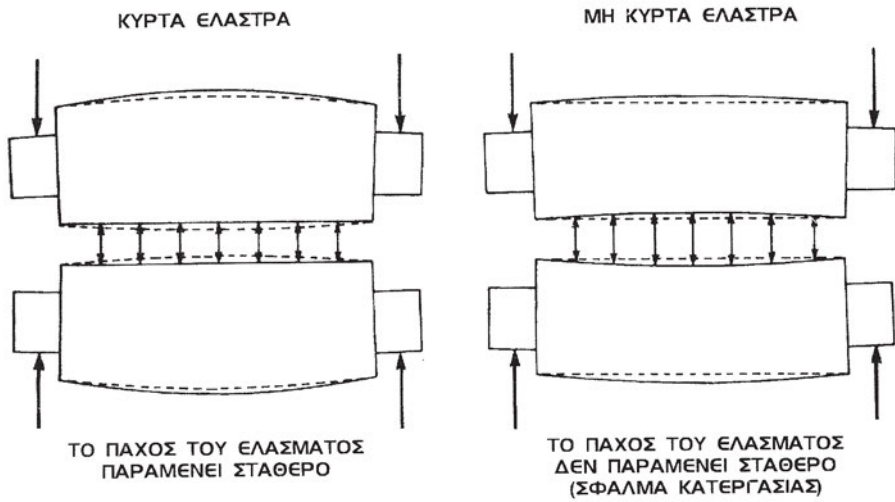
Σχήμα 13.25: Κύρτωση κυλίνδρων
