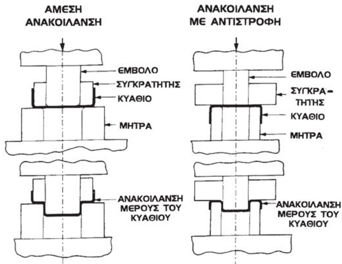
Σχήμα 14.26: Είδη ανακοίλανσης
