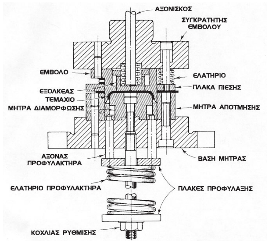
Σχήμα 14.24: Σύνθετο εργαλείο κοίλανσης
