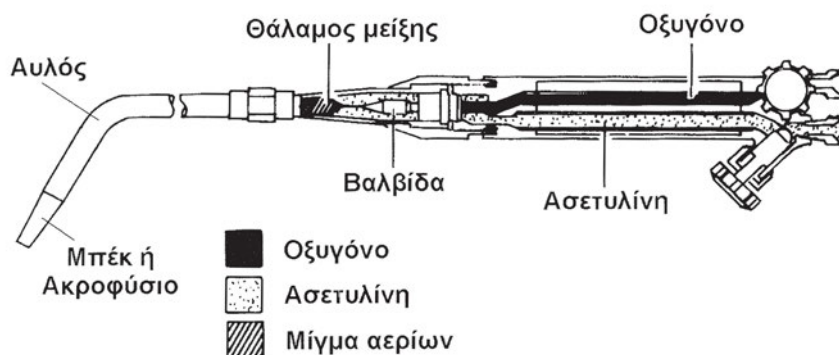
Σχήμα 16.5: Καυστήρας οξυγονοκόλλησης
