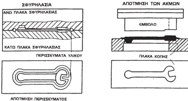
Σχήμα 13.11: Σφυρηλάτηση κλειδιού
