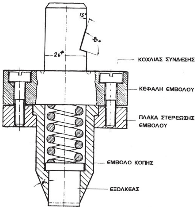
Σχήμα 14.15: Εργαλείο απότμησης
