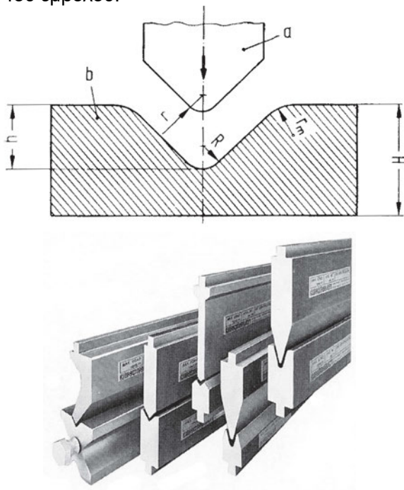
Σχήμα 14.43: Εργαλεία κάμψης V
