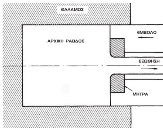
Σχήμα 13.33: Έμμεση εξώθηση
