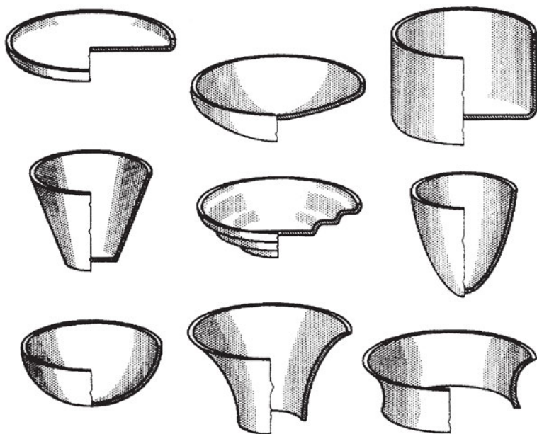
Σχήμα 14.45: Προϊόντα περιώθησης
