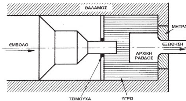
Σχήμα 13.36: Υδροστατική εξώθηση.
