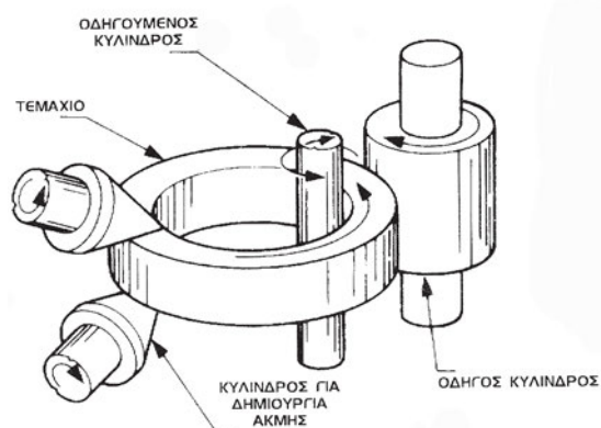
Σχήμα 13.28: Έλαση δακτυλίου
