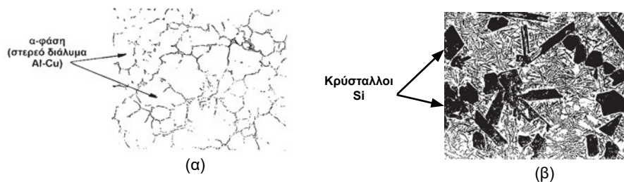
Σχήμα 7.2: (α) Δομή κράματος Al-Cu (σειρά 2000). Διακρίνονται κόκκοι της α-φάσης (κ.ε.) η οποία είναι το στερεό διάλυμα Al-Cu. (β) Δομή κράματος Al-Si (σειρά 4000). Διακρίνονται οι κρύσταλλοι Si (σκούρα φάση) μέσα σε ευτηκτικό Al-Si. (Μεγέθυνση X100).
