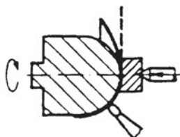
Σχήμα 12.12: Ολκή, Βαθεία κοίλανση, Περίωθηση
