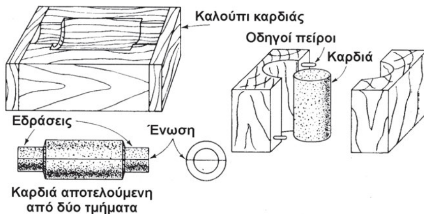
Σχήμα 10.5: Κατασκευή καρδιών
