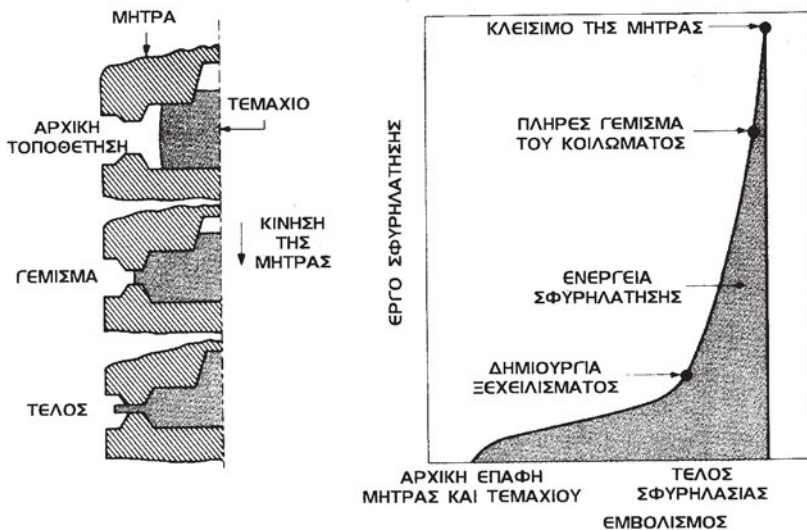
Σχήμα 13.7: Διάγραμμα έργου-εμβολισμού σε σφυρηλασία με κλειστές μήτρες
