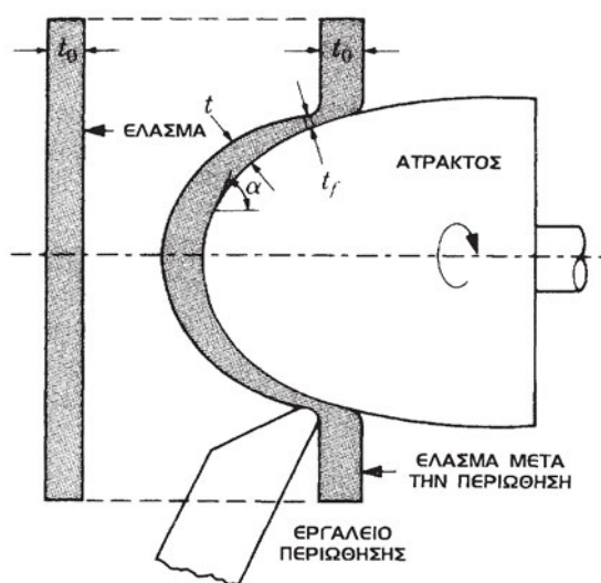
Σχήμα 14.50: Δοκιμή περιώθησης
