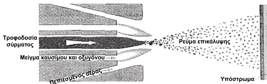
Σχήμα 18.6: Σχηματική παράσταση του ψεκασμού φλόγας
