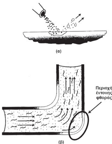
Σχήμα 17.4: Σχηματική παράσταση της μηχανικής διάβρωσης, (α) λόγω πρόσκρουσης στερεών σωματιδίων πάνω στην επιφάνεια του υλικού (π.χ. αμμοβολή) και (β) λόγω της ροής μειγμάτων υγρών/στερεών.
