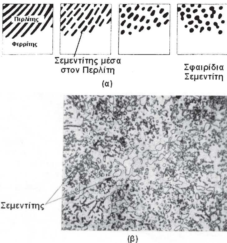
Σχήμα 5.2: (α) Σχηματική παράσταση του μηχανισμού σφαιροποίησης του σεμεντίτη μέσα στον περλίτη. (β) Οπτική μικρογραφία χάλυβα μετά από ανόπτηση σφαιροποίησης, X500.
