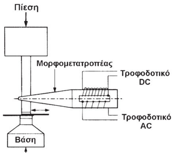
Σχήμα 16.23: Συγκόλληση με υπερήχους
