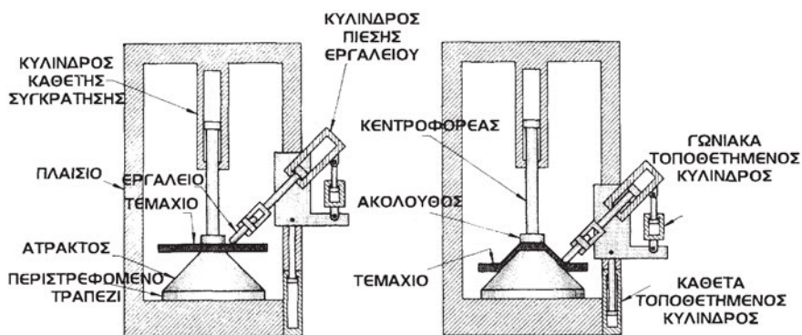
Σχήμα 14.53: Μηχανική περιώθηση
