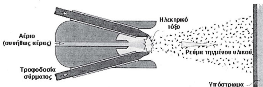
Σχήμα 18.7: Σχηματική παράσταση του ψεκασμού με ηλεκτρικό τόξο.
