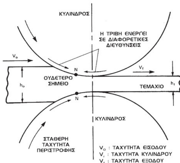
Σχήμα 13.16: Ουδέτερο σημείο
