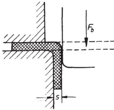
Σχήμα 14.37: Κάμψη σκέλους
