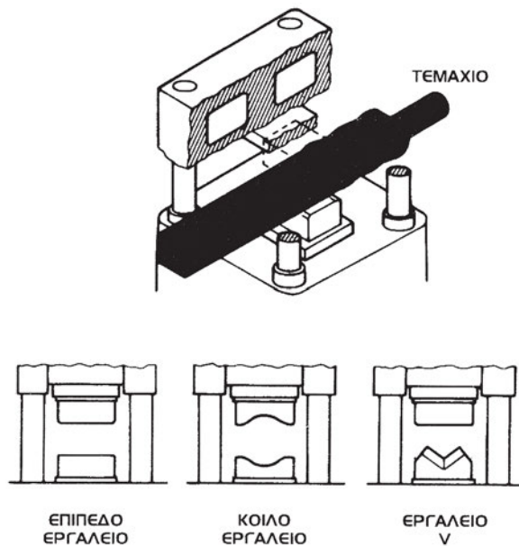
Σχήμα 13.4: Τύποι από ανοικτές μήτρες
