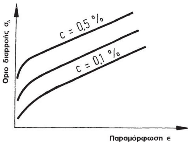
Σχήμα 12.6: Επίδραση περιεκτικότητας σε C στο όριο διαρροής χαλύβων σε σχέση με την παραμόρφωση
