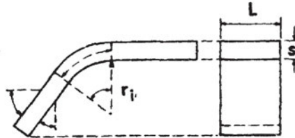
Σχήμα 14.32: Ορολογία κάμψης
