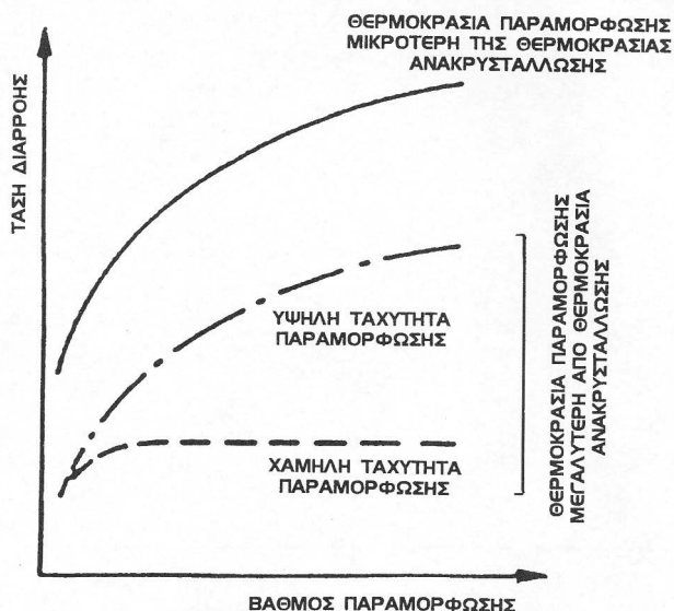
Σχήμα 12.5: Επίδραση της ταχύτητας παραμόρφωσης στο όριο διαρροής
