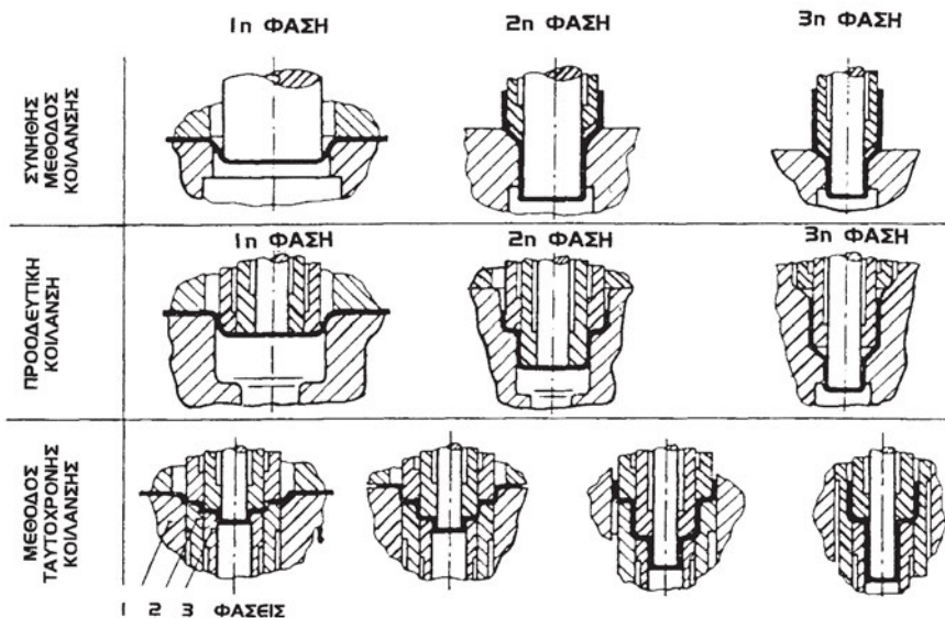
Σχήμα 14.27: Μέθοδοι ανακοίλανσης
