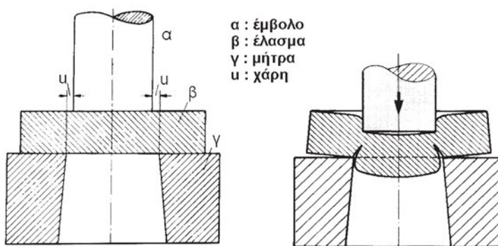
Σχήμα 14.1: Απότμηση
