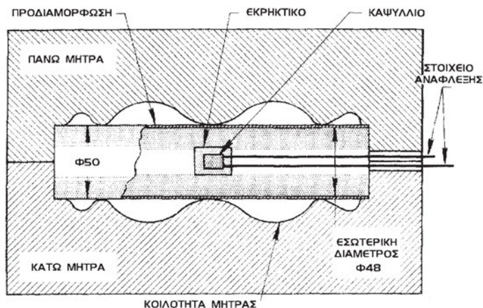
Σχήμα 15.8: Κλειστό σύστημα εκρηκτικής διαμόρφωσης ελάσματος
