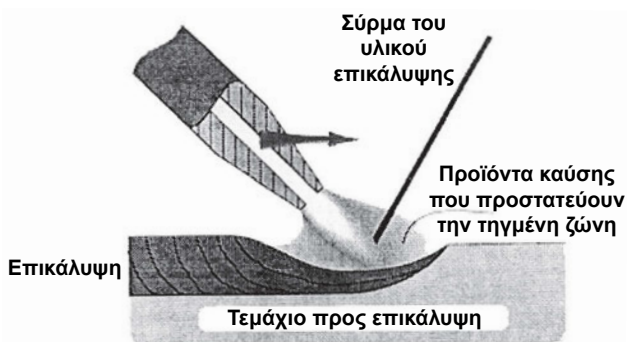
Σχήμα 18.5: Απόθεση υλικού με τη βοήθεια φλόγας καυσίμου-οξυγόνου
