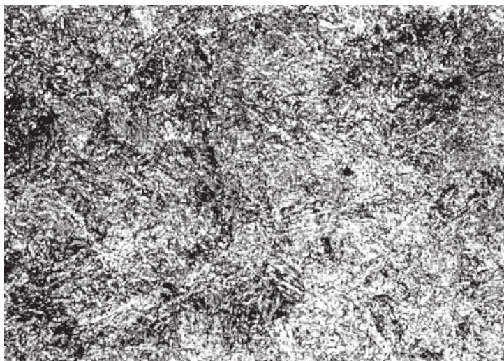
Σχήμα 5.11: Οπτική μικρογραφία χάλυβα μετά από επαναφορά (μαρτενσίτης από επαναφορά), Χ100.
