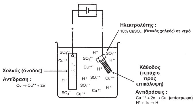
Σχήμα 18.3: Ηλεκτρολυτικό κελί επιχάλκωσης
