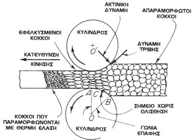
Σχήμα 13.17: Ουδέτερο σημείο
