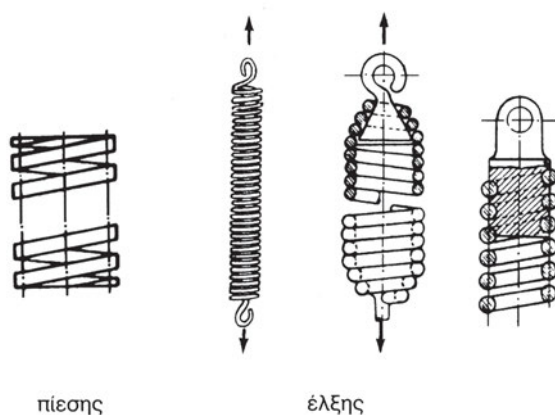
Εικ.7.6β Κυλινδρικά ελικοειδή ελατήρια
