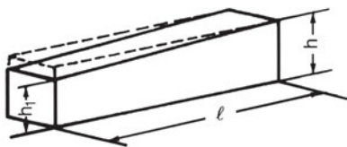
Εικ. 7.5β Τυπική σφήνα
