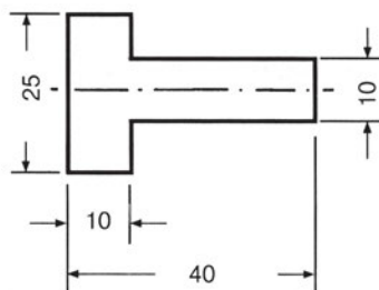
Εικ. 6.3ε Οι γραμμές διαστάσεων δεν πρέπει να κόβουν τις γραμμές του σχεδίου
