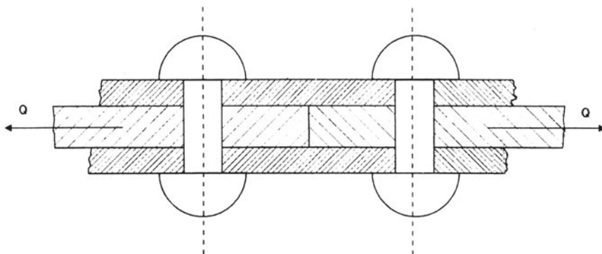
Εικ. 14.3β Ήλωση παραδείγματος 1
