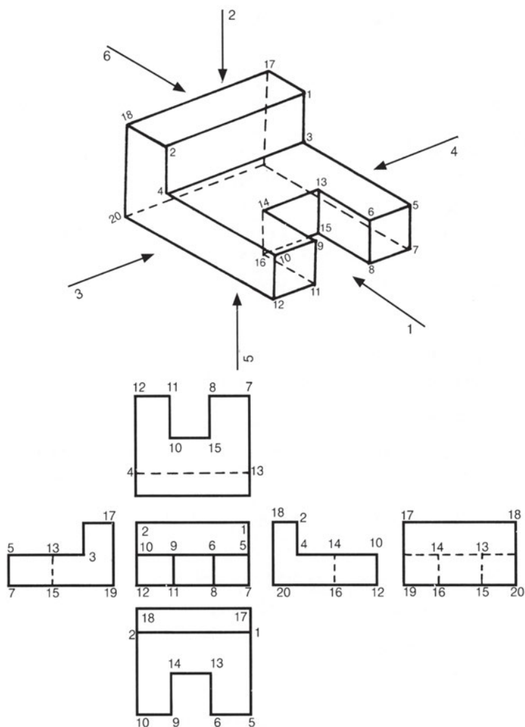
Εικ. 6.2γ Τοποθέτηση των όψεων κατά το Ευρωπαϊκό σύστημα
