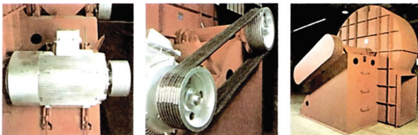
Εικ. 14.9α Ιμαντοκίνηση παραδείγματος εφαρμογής
