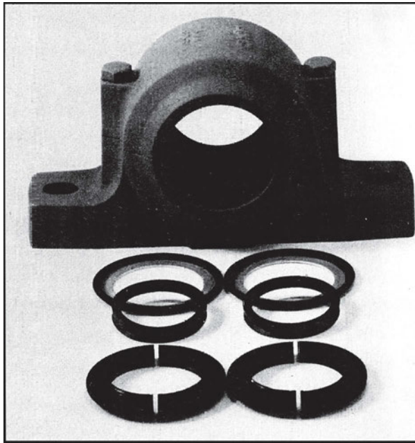
Εικ. 9.2ια “Θήκη” στήριξης ρουλμάν
