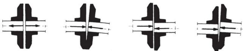
Εικ. 9.3ια Γεωμετρικά σφάλματα τοποθέτησας εύκαμπτων συνδέσμων
