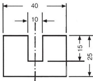
Εικ. 6.3β Κάθε διάσταση πρέπει να αναγράφεται μία μόνο φορά και στην πιο κατάλληλη θέση λαμβάνοντας υπόψη τον τρόπο κατασκευής του εξαρτήματος
