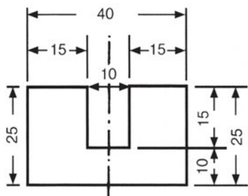
Εικ. 6.3β Κάθε διάσταση πρέπει να αναγράφεται μία μόνο φορά και στην πιο κατάλληλη θέση λαμβάνοντας υπόψη τον τρόπο κατασκευής του εξαρτήματος
