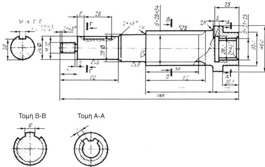
Εικ. 9.1ζ Σχεδιασμός ατράκτου
