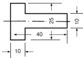
Εικ. 6.3ε Οι γραμμές διαστάσεων δεν πρέπει να κόβουν τις γραμμές του σχεδίου
