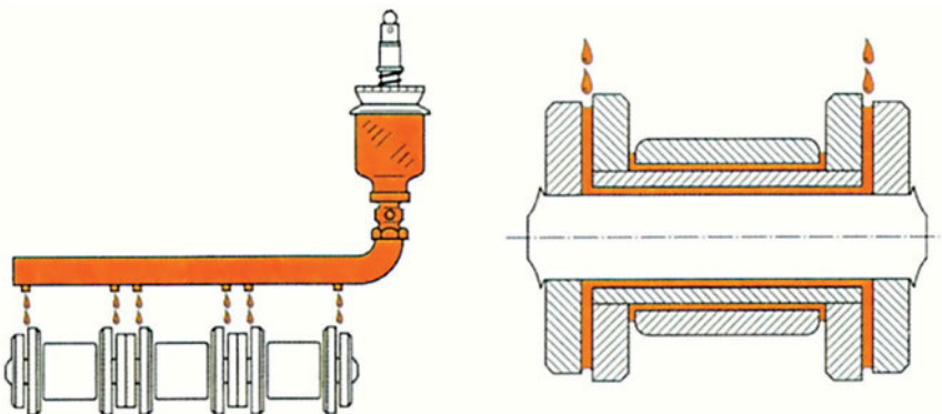
Εικ.10.3ιδ Λίπανση σταγόνων. Δεξιά φαίνονται τα σημεία που πρέπει να λιπανθούν
