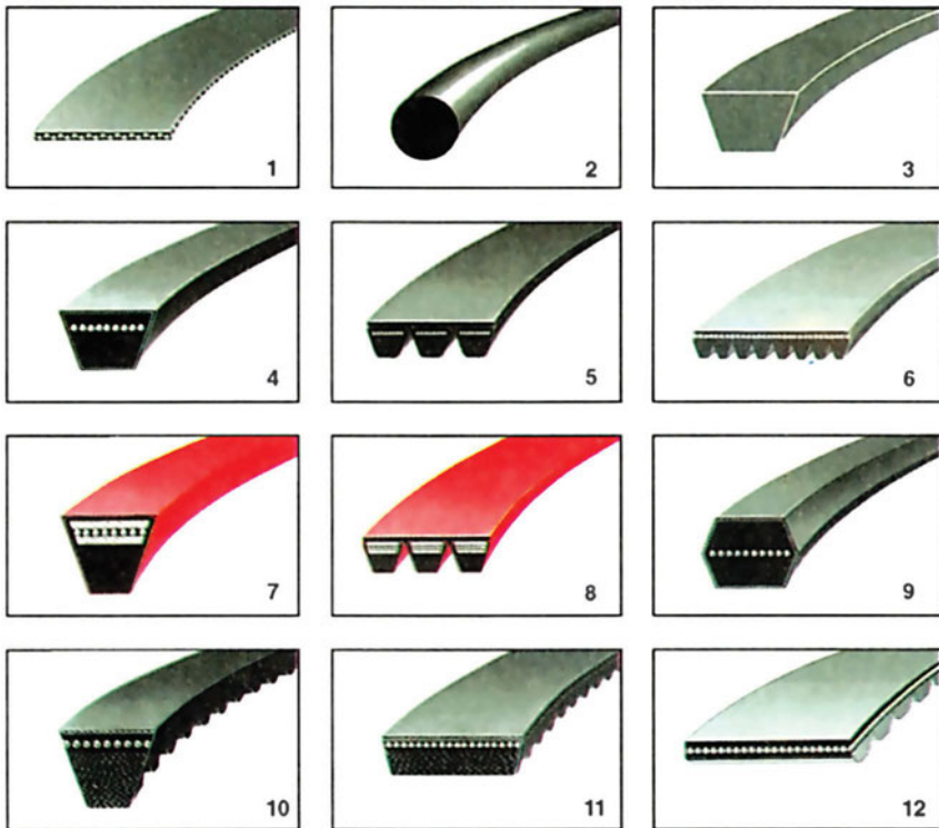
Εικ. 10.26 Τύποι ιμάντων: 1) επίπεδος, 2) κυκλικός, 3) κοινός τραπεζοειδής, 4,5,6) ενισχυμένοι τραπεζοειδείς, 7,8) στενοί ενισχ. τραπεζοειδείς, 10,11,12) ιμάντες χρονισμού με οδόντωση
