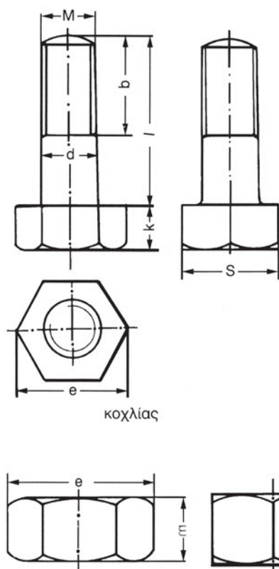
Εικ. 7.3ιγ Σχεδίαση εξάγωνου κοχλίας και περικοχλίου
