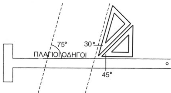
Εικ. 2.3δ Χρήση των οργάνων σχεδίασης για τη δημιουργία των 75^\circ
