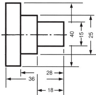
Εικ. 6.3στ Οι κύριες γραμμές διαστάσεων δεν πρέπει να διασταυρώνονται μεταξύ τους ή με τις βοηθητικές. Οι μεγαλύτερες διαστάσεις τοποθετούνται “έξω” από τις μικρότερες
