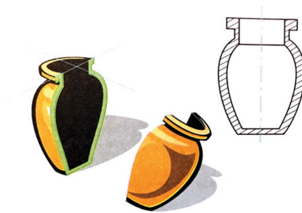
Εικ. 4.2η Βάζο σε κανονική τομή
