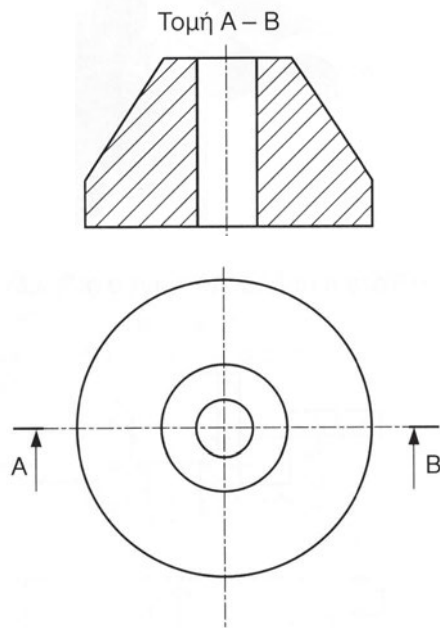
Εικ.4.2ε Σχεδίαση και σήμανση της τομής
