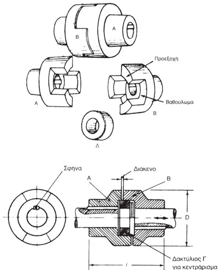
Εικ. 9.33 “Αξονικά” κινητοί σύνδεσμοι
