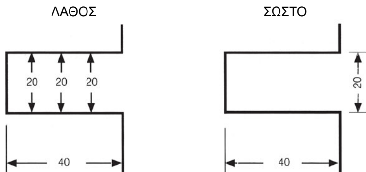
Εικ. 6.30 Οι αριθμοί των διαστάσεων στο μηχανολογικό σχέδιο συμβολίζουν πάντα mm , γι' αυτό και δεν αναγράφεται η μονάδα μέτρησης δίπλα τους. Οι αριθμοί των διαστάσεων είναι γραμμένοι κατακόρυφα ή οριζόντια (στροφή 90^\circ αντίστροφα από τους δείκτες του ωρολογίου)
