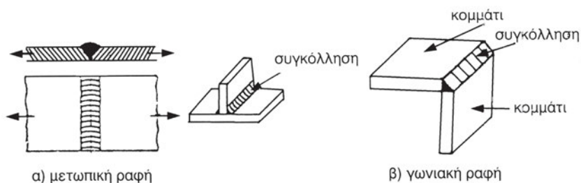
Εικ. 7.4δ Μορφές ραφών
