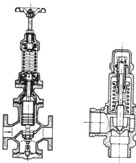
Εικ.12.4στ Ασφαλιστικά όργανα
