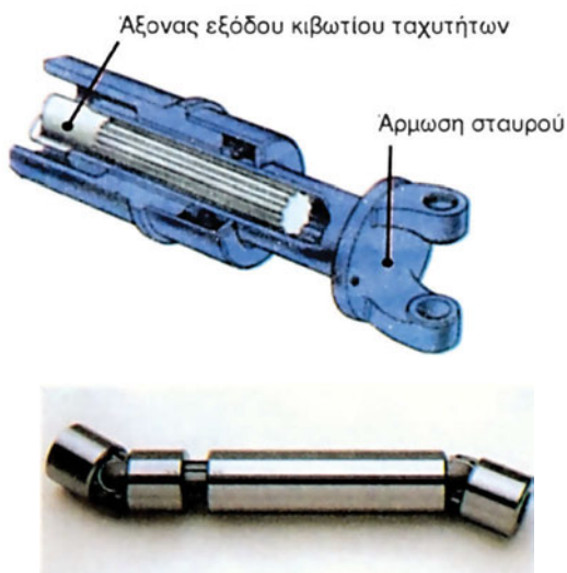
Εικ. 9.3στ “Αξονικά” κινητοί σύνδεσμοι
