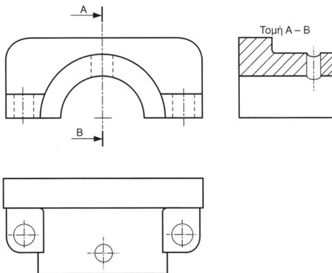
Εικ. 4.2β Σχεδίαση της τομής αντικειμένου
