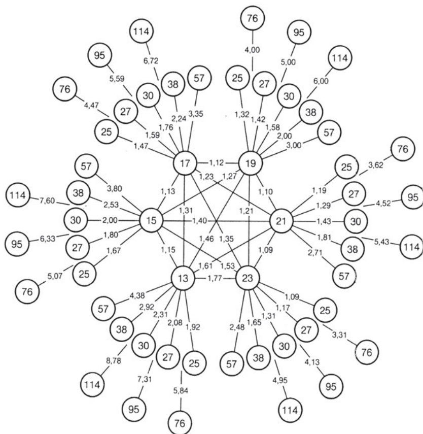
Εικ. 10.3ιβ Αριθμοί δοντιών τυποποιημένων αλυσοτροχών και αντίστοιχες δυνατές σχέσεις μετάδοσης
