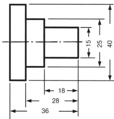
Εικ. 6.3στ Οι κύριες γραμμές διαστάσεων δεν πρέπει να διασταυρώνονται μεταξύ τους ή με τις βοηθητικές. Οι μεγαλύτερες διαστάσεις τοποθετούνται “έξω” από τις μικρότερες
