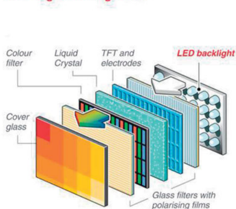
Εικόνα 72: LCD & LED οθόνες
