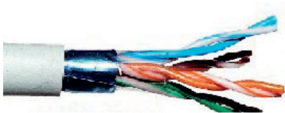
Εικ. 5.4. Καλώδιο FTP.
