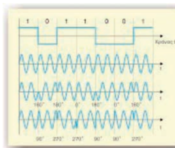
Σχ. 2.8. Διαμόρφωση PSK (σταθερής αναφοράς).
