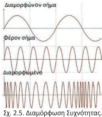
Σχ. 2.5. Διαμόρφωση Συχνότητας.
