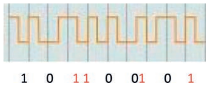
Σχ. 2.10. Διαφορική Κωδικοποίηση Manchester.
