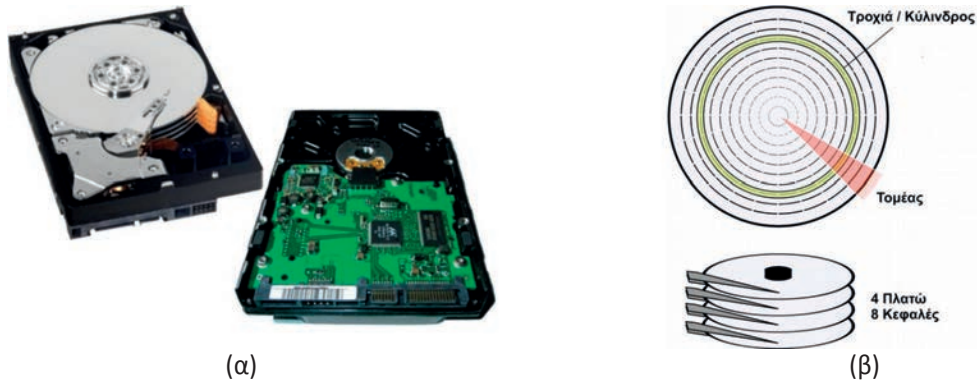
Εικ.1.20 : (α) Το εσωτερικό ενός σκληρού δίσκου, (β) Λογική οργάνωση ενός «πλατώ».
