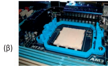
Εικ. 1.10.(α) Socket επεξεργαστών της Intel, (β) Socket επεξεργαστών της AMD
