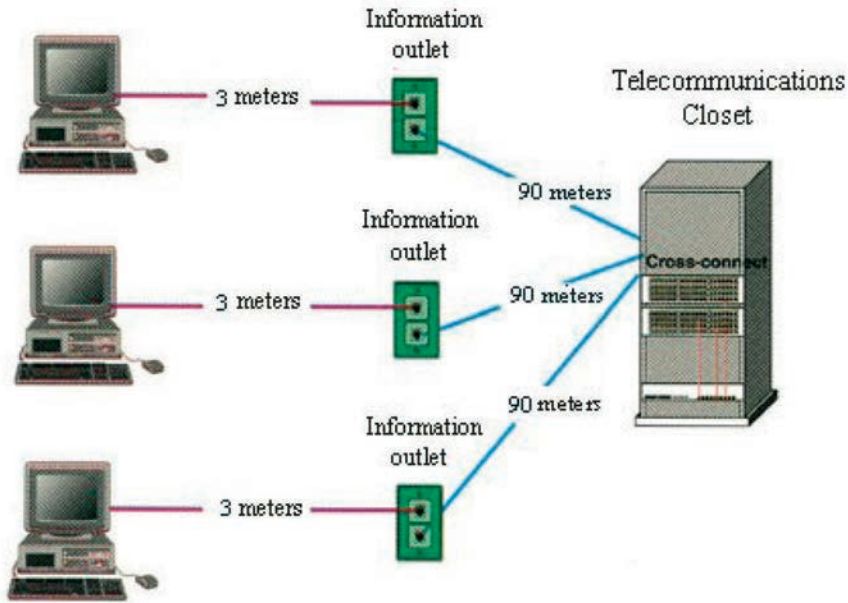
Σχ. 5.8. Οριζόντια καλωδίωση.
