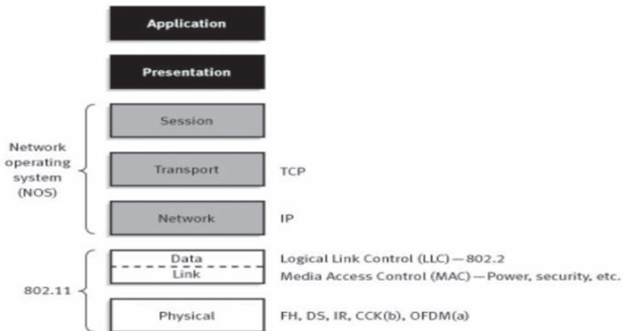
Σχ. 4.12. Σχηματική αναπαράσταση του δικτύου IEEE 802.11 στο μοντέλο αναφοράς OSI
