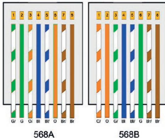
Σχ. 5.2. Διάταξη καλωδίων TP.
