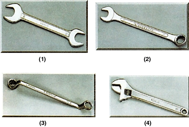
Σχήμα 4.4.2α -1. Γερμανικό κλειδί, -2. Πολυγωνικό κλειδί, -3. Κλειδί συνδυασμένου τύπου, -4. Γαλλικό κλειδί
