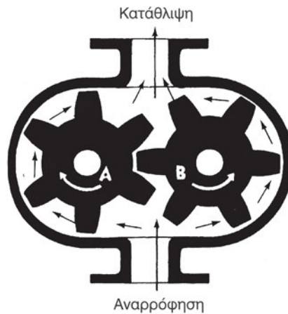
Σχήμα 16.1.1β Αντλία με οδοντωτούς τροχούς A: Κινητήριος οδοντωτός τροχός B: Κινούμενος οδοντωτός τροχός
