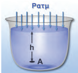
Εικόνα 4.20. Η πίεση στο Α είναι: p_A = p_{\text{ατμοσφαιρική}} + \rho \cdot g \cdot h
