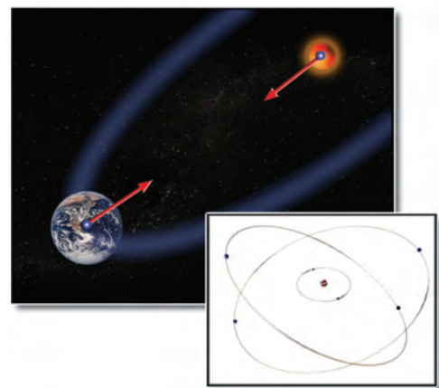
Εικόνα 3.36. Η δύναμη που ασκεί ο πυρήνας στο ηλεκτρόνιο προκαλεί την κίνησή του γύρω απ' αυτόν. Η βαρυντική έλξη που ασκεί ο ήλιος στη γη, προκαλεί την περιφορά της γύρω του.
