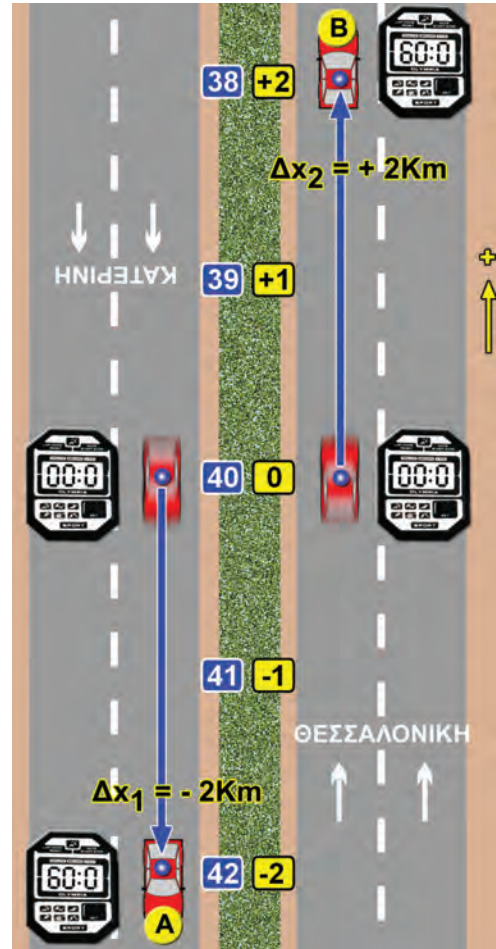
Εικόνα 2.9. Ως αρχή μέτρησης του χρόνου επιλέχθηκε η χρονική στιγμή που τα δυο αυτοκίνητα βρίσκονταν στο 40ό km. Τη χρονική στιγμή t = 60 \text{ s} το A βρέθηκε στο 42ο km και το B στο 38ο km.
