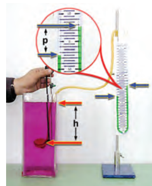
Εικόνα 4.8. Η επιφάνεια βρίσκεται σε βάθος h και είναι: (α) οριζόντια, (β) κατακόρυφη.
