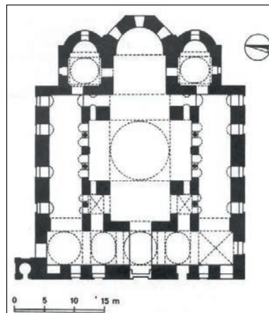
Κάτοψη τρουλαίας Βασιλικής (Ι.Ν. της του Θεού Σοφίας Θεσσαλονίκης)
