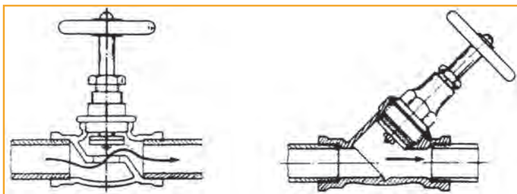
Εικόνα 7.8 Διακόπτες ροής
