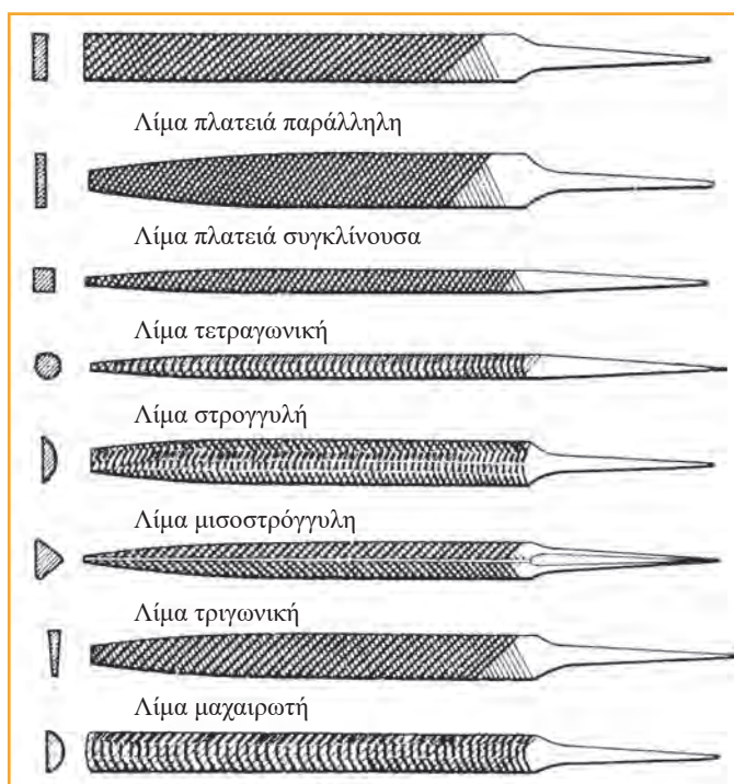
Εικόνα 3.9 Διάφορες λίμες
