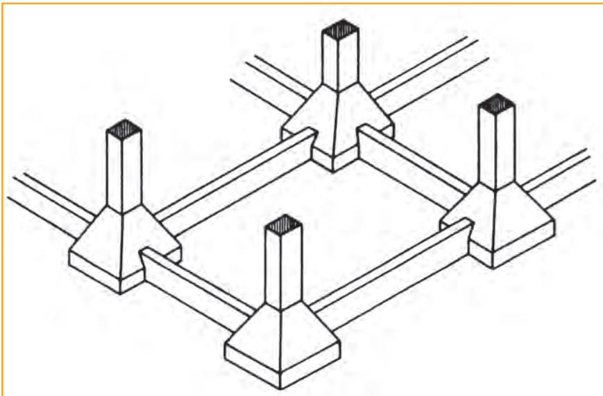
Εικόνα 4.3 Θεμελίωση μερικής κατάστρωσης
