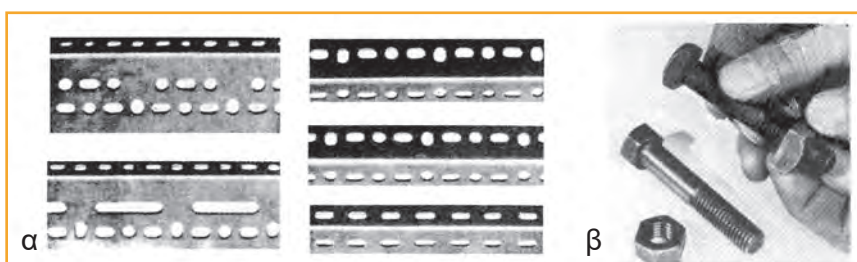
Εικόνα 3.3 α. Διάτρητα γωνιακά ελάσματα τύπου ντέξιον β. Μπουλόνια και παξιμάδια
