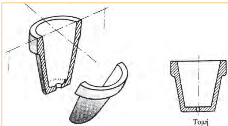
Εικόνα 1.37 Τομή αντικειμένου
