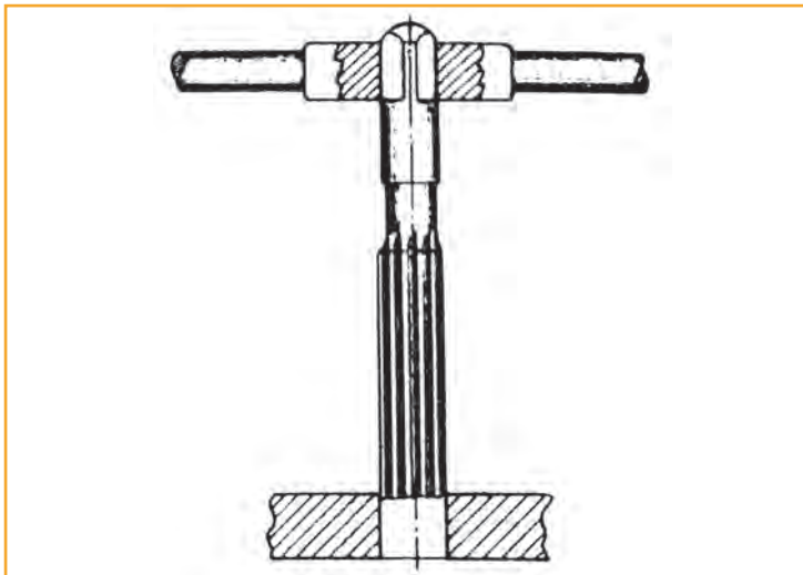
Εικόνα 3.21 Γλύφανο
