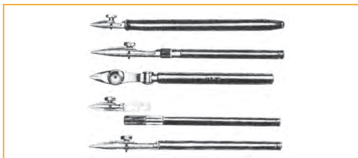
Εικόνα 1.21 Γραμμοσύρτες
