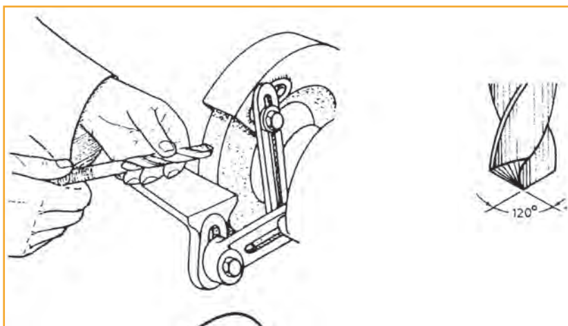
Εικόνα 3.25 Τρόχισμα τρυπανιού
