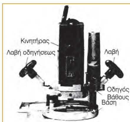
Εικόνα 2.16 Γενική φρέζα χειρός
