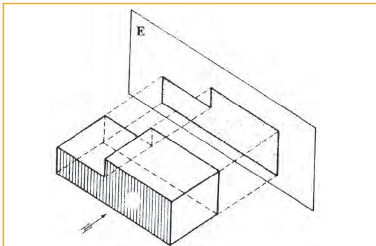
Εικόνα 1.36 Πρόσωση αντικειμένου
