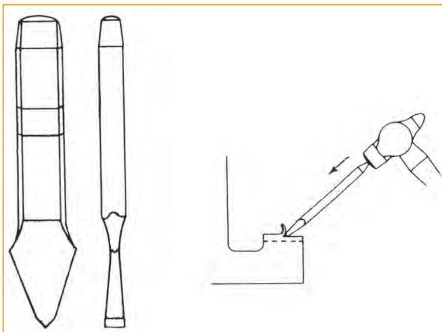
Εικόνα 3.11 Διάφορα κοπίδια και κοπίδιασμα
