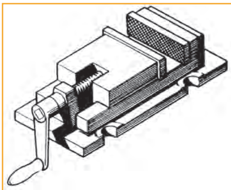
Εικόνα 3.7 Μέγγενη εργαλειομηχανών
