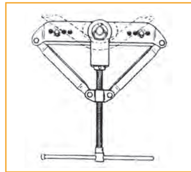
Εικόνα 7.2 Κουρμπαδόρος
