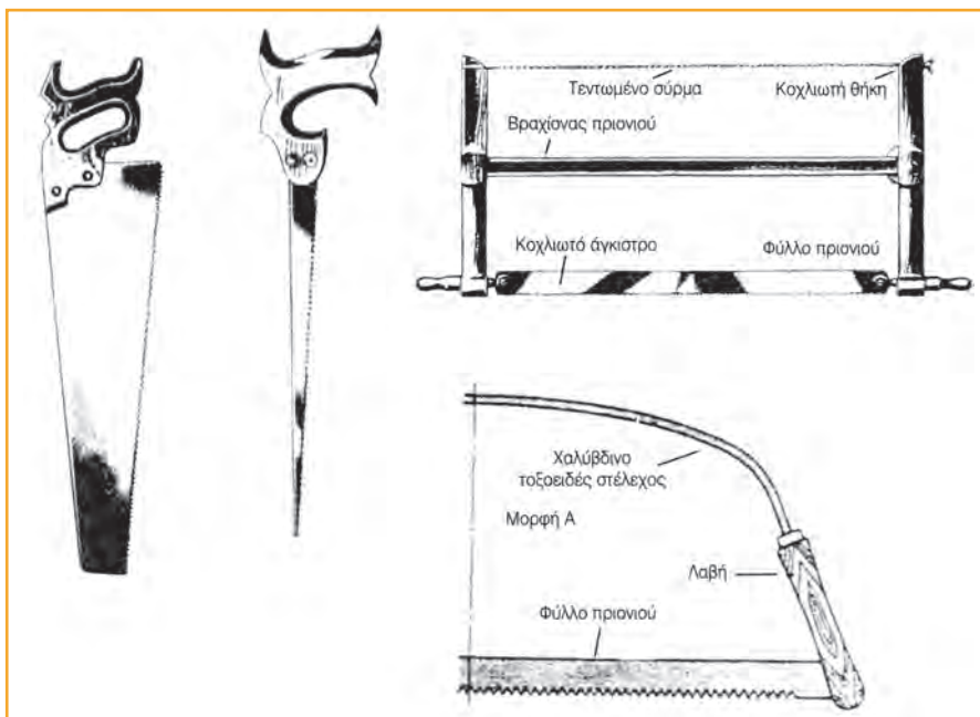
Εικόνα 2.1 Διάφορα πριόνια
