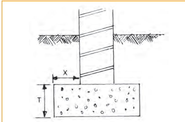
Εικόνα 4.2 Θεμέλιο με βάση
