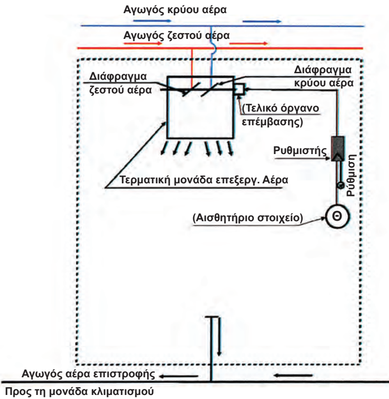
Σχήμα 2.55: Σχηματική παράσταση ελέγχου της θερμοκρασίας του χώρου με κλειστό κύκλωμα.
