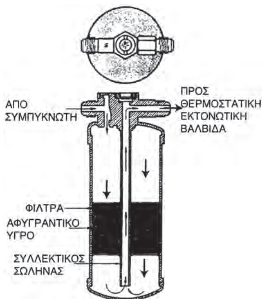
Σχήμα 6.19: Συλλέκτης υγρού.
