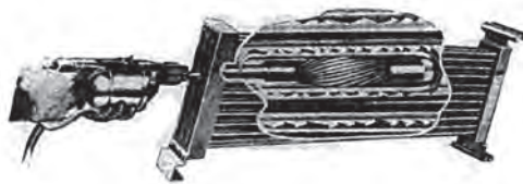
Εικόνα 2.6: Μηχανικός καθαρισμός εσωτερικών σωλήνων υδρόψυκτης συμπυκνωτή παράλληλων ομοαξονικών σωλήνων.
