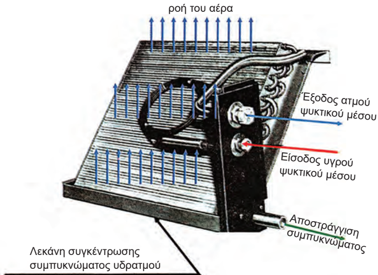
Σχήμα 2.37: Κεκλιμένο στοιχείο ατμοποίησης.
