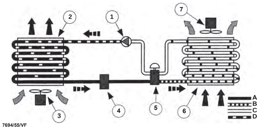
Σχήμα 6.4: Κύκλωμα ψυκτικού με βαλβίδα εκτόνωσης.
