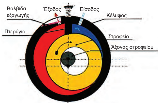
Σχήμα 2.5: Σχηματική παράσταση (σε τομή) βασικών δομικών στοιχείων περιστροφικού συμπίεστή με σταθερό σύρτη (πτερύγιο) και έκκεντρο στροφέιο.
