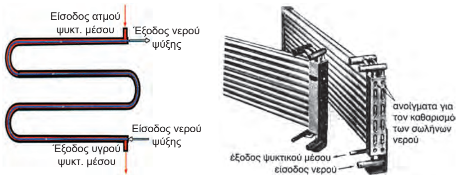
Σχήμα 2.20: Σπειροειδής ομοαξονικός σωλήνας (1) και στοιχείο υδρόψυκτης συμπυκνωτή με παράλληλους ομοαξονικούς σωλήνες. (2). Ο μηχανικός καθαρισμός των σωλήνων νερού γίνεται αφού πρώτα αφαιρεθεί το πλευρικό σχετικό κάλυμμα.
