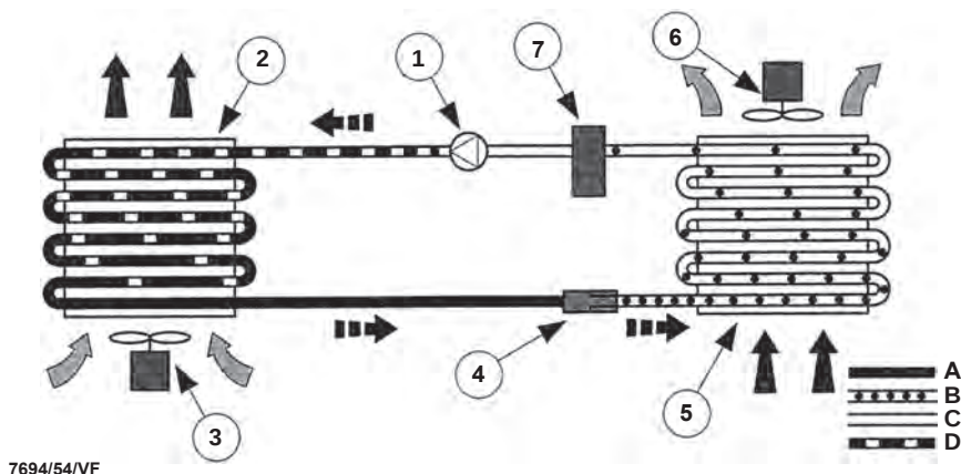
Σχήμα 6.3: Κύκλωμα ψυκτικού με σωλήνα σταθερής διαμέτρου.
