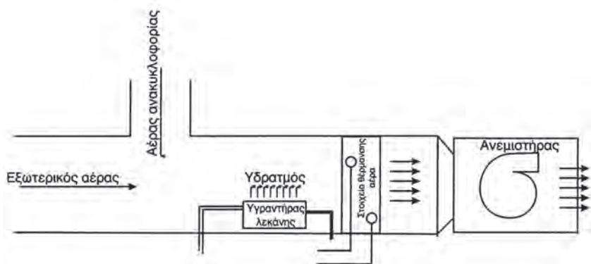
Σχήμα 2.44: Σχηματική παράσταση ύγρανσης του αέρα με υγραντήρα λεκάνης.
