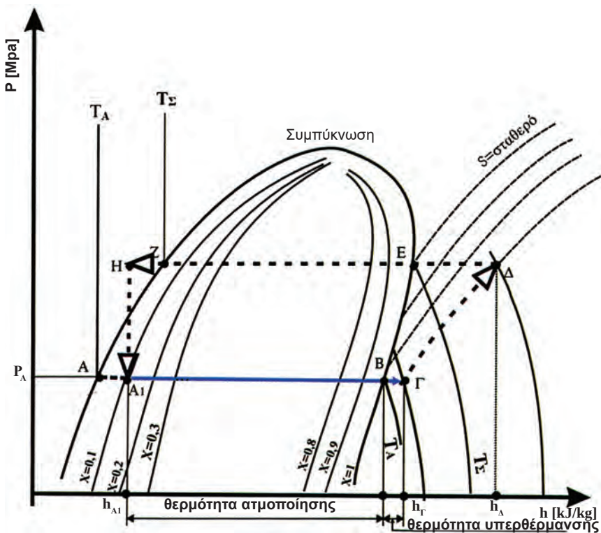
Σχήμα 2.34: Σχηματική παράσταση της πορείας της ατμοποίησης (Α,Β) και της υπερθέρμανσης, εάν αυτή προβλέπεται (ΒΓ) ενός ψυκτικού μέσου, σε διάγραμμα πίεσης – ενθαλπίας (p-h).
