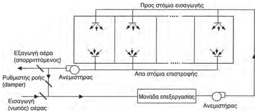
Σχήμα 5.2: Σχηματικό διάγραμμα κεντρικού κλιματισμού και κυκλοφορίας του αέρα.
