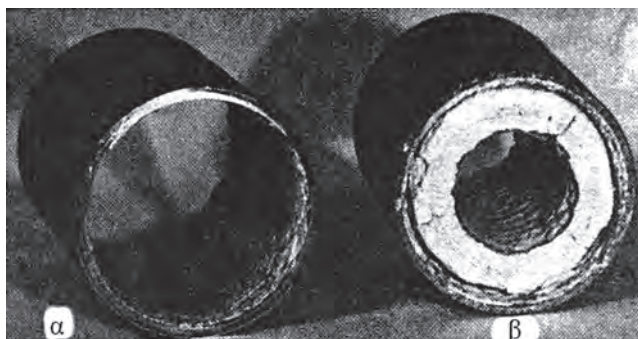
Εικόνα 2.5: Σχηματισμός κρούστας στους σωλήνες ενός υδρόψυκτου συμπυκνωτή. Επικαθήσεις όταν χρησιμοποιείται: α) αποσκληρυμένο νερό και β) με σκληρό νερό (δεν έχει γίνει αποσκληρίυνση).
