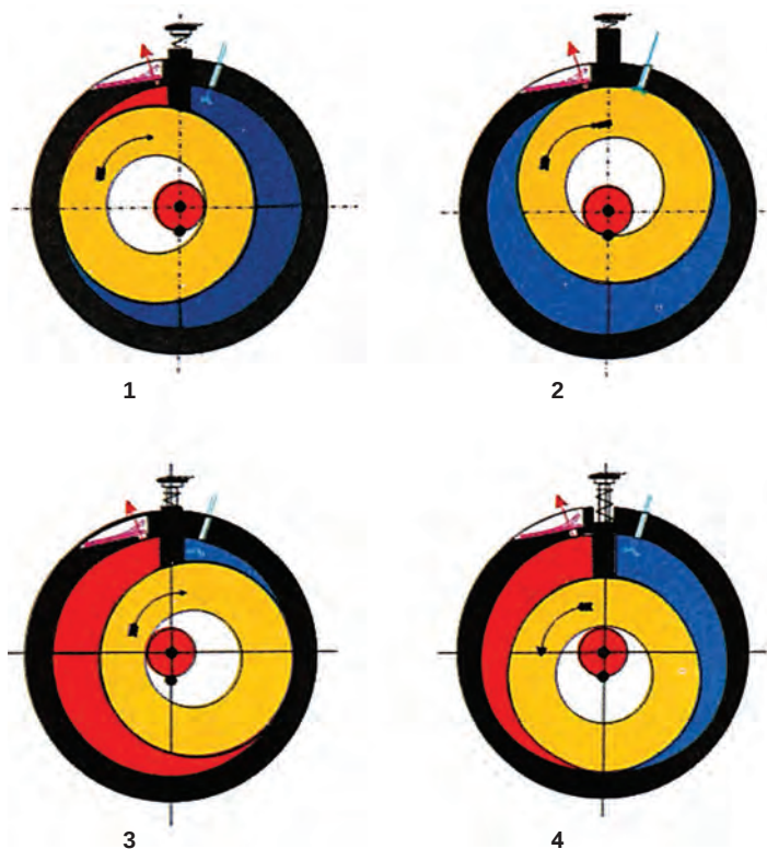
Σχήμα 2.6: Σχηματική παράσταση αρχής λειτουργίας περιστροφικού συμπίεστή με σταθερό σύρτη και έκκεντρο στροφέιο.
