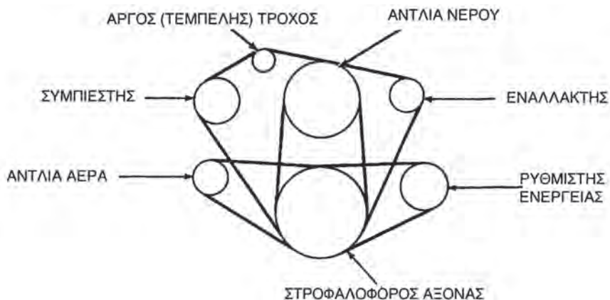
Σχήμα 6.12: Ο συμπίεστές κινείται από το στροφαλοφόρο άξονα με ρύθμιση των ιμάντων από μια αργοκίνητη τροχαλία.
