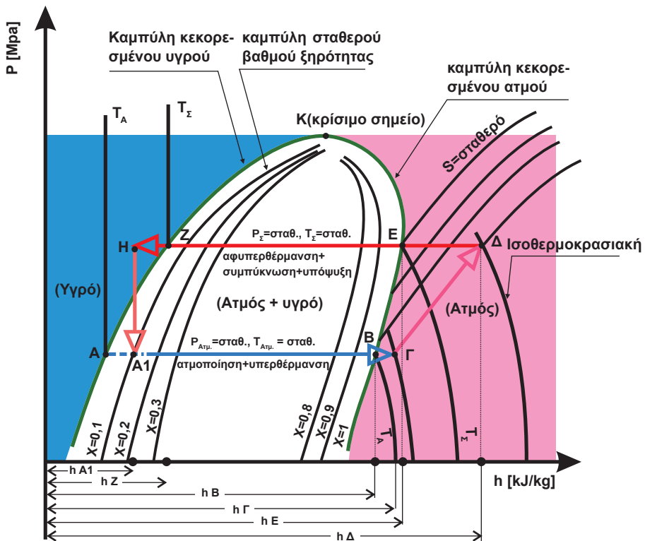
Σχήμα 2.1: Σχηματική παράσταση ψυκτικού κύκλου στο διάγραμμα p-h , όπου Α,Β=Ατμοποίηση, ΒΓ= Υπερθέρμανση, ΓΔ= Συμπύκνωση, ΔΕ= Αφυπερθέρμανση, ΕΖ=Συμπύκνωση, ΖΗ=υπόψυξη, Η Α 1 =εκτόνωση.
