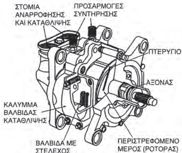
Σχήμα 6.9: Περιστροφικός συμπίεστής με πτερύγια.
