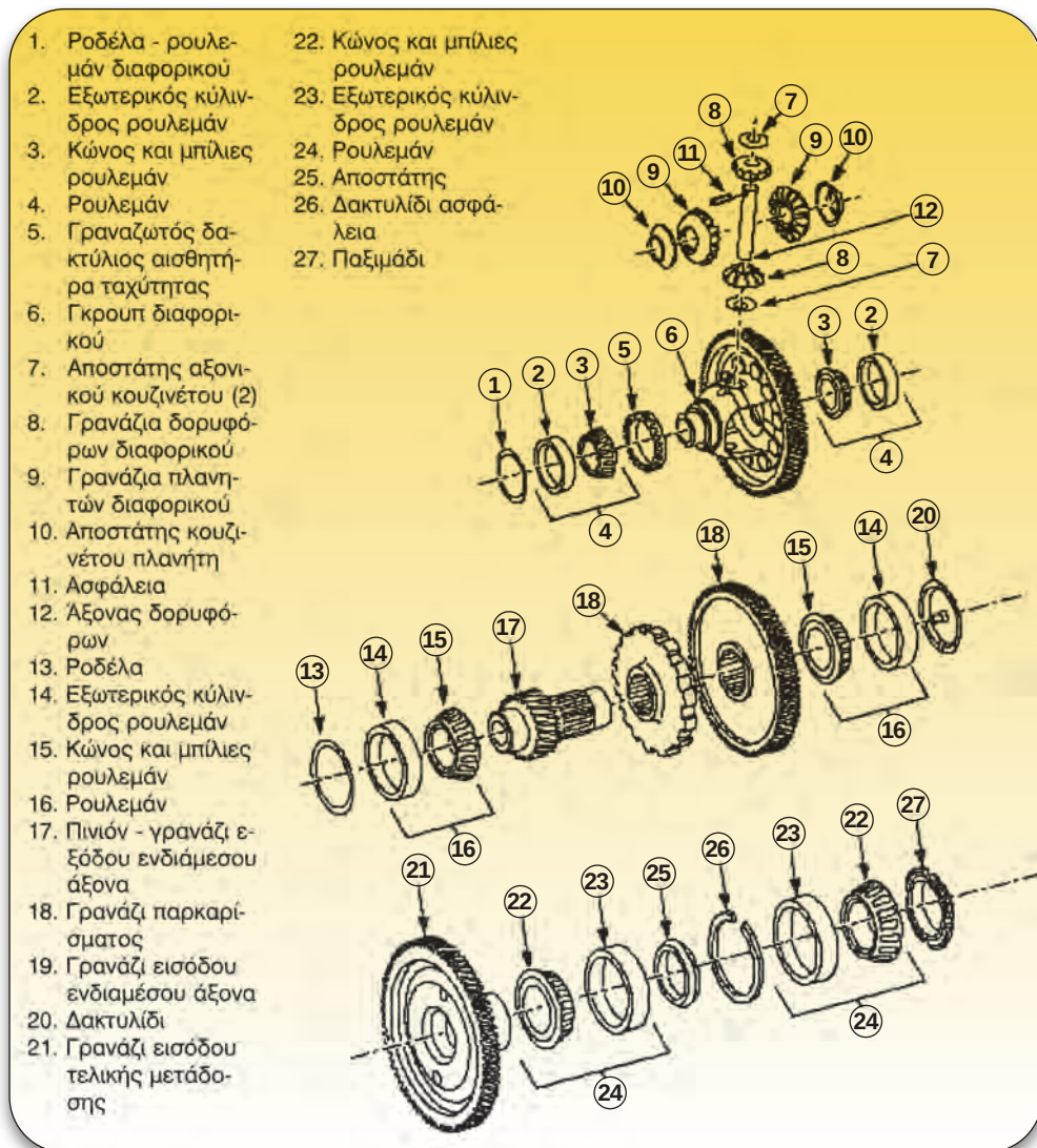
Σχήμα 1.27: Συγκρότημα διαφορικού.
