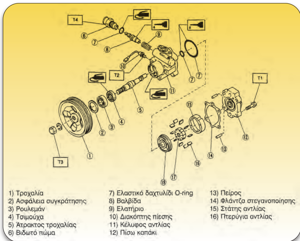
Σχήμα 2.90: Εξαρτήματα της αντλίας του συστήματος διεύθυνσης με υδραυλική υποβοήθηση.
