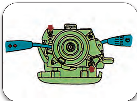
Σχήμα 2.29: Αφαίρεση διακοπών.
