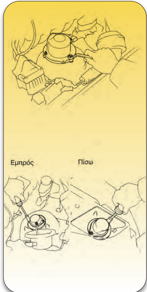
Σχήμα 3.15: Αφαίρεση ενεργοποιητών.
