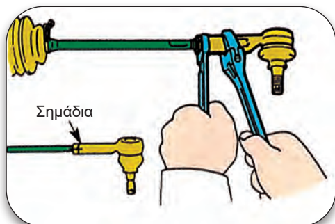
Σχήμα 2.37: Σημάδεμα και αφαίρεση ακρόμπαραυ.
