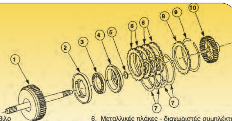
Σχήμα 1.23: Μετατροπέας ροπής και αντλία λαδιού.
