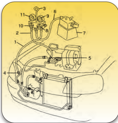
Σχήμα 6.9: Συνδεσμολογία οργάνων και αντλία εκκένωσης ψυκτικού.
