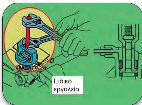
Σχήμα 2.52: Αφαίρεση κουζινέτου.
