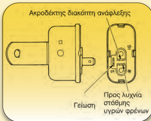
Σχήμα 5.14: Έλεγχος της καλής λειτουργίας του αισθητήρα.
