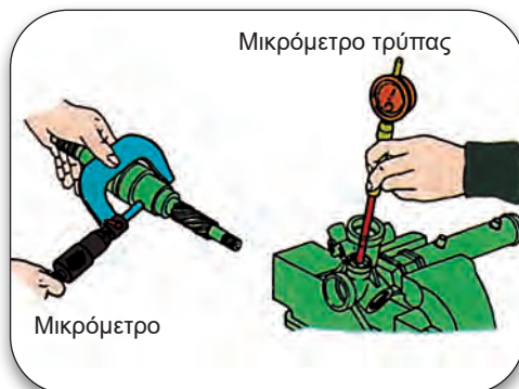
Σχήμα 2.51: Έλεγχος ανοχών άξονα και βαλβίδας ελέγχου.
