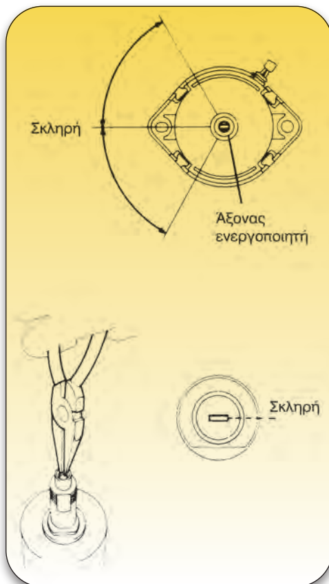
Σχήμα 3.17: Τοποθέτηση ενεργοποιητή.
