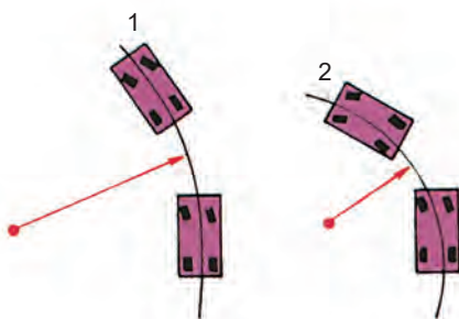
Σχήμα 2.98: Χαρακτηριστικά κίνησης αυτοκινήτου με 4-διεύθυνση.
