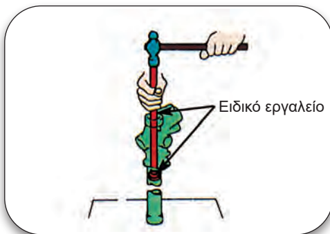
Σχήμα 2.49: Αφαίρεση οδοντωτού κανόνα.
