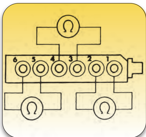
Σχήμα 4.12: Μέτρηση της ωμικής αντίστασης των ηλεκτρομαγνητικών βαλβίδων.
