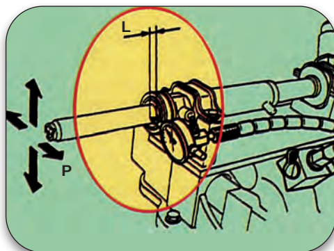
Σχήμα 2.65: Έλεγχος ακτινικής χάρης κανόνα (στροφή δεξιά).
