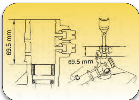
Σχήμα 2.54: Τοποθέτηση κουζινέτων.
