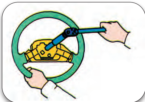
Σχήμα 2.26: Αφαίρεση τιμονιού.
