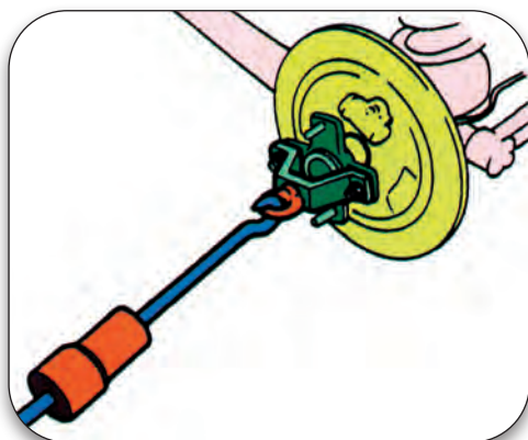
Σχήμα 1.31: Αφαίρεση ημιαξονίου.
