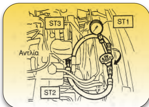
Σχήμα 2.97: Έλεγχος της πίεσης ανακούφισης.
