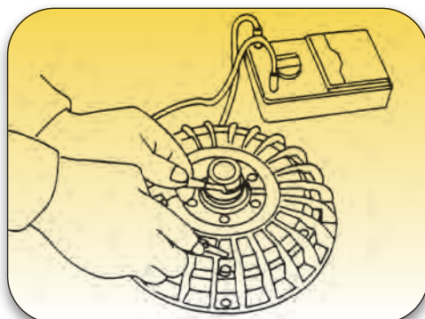
Σχήμα 1.7: Έλεγχος μόνωσης κελύφους του ηλεκτρομαγνητικού συμπλέκτη.
