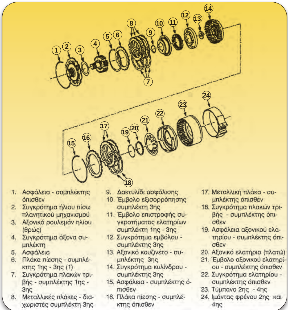
Σχήμα 1.26: Συγκρότημα συμπλέκτη όπισθεν και 1ης - 3ης και φρένου (ταινιοπέδη) 2ης / 4ης.
