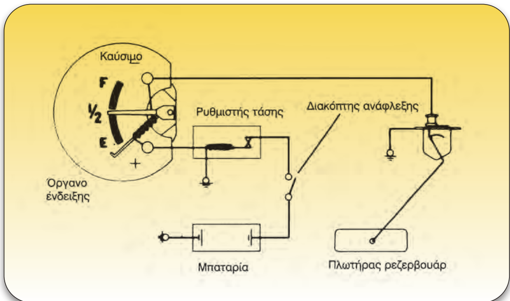
Σχήμα 5.1: Συνδεσμολογία ηλεκτρικού κυκλώματος οργάνου ένδειξης της στάθμης καυσίμου.
