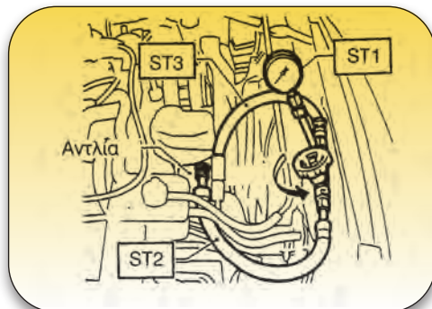
Σχήμα 2.96: Έλεγχος της πίεσης του ρυθμιστή.
