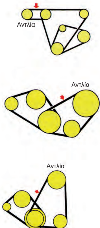
Σχήμα 2.5: Θέση ρύθμισης σε διάφορες διατάξεις τροχαλιών.
