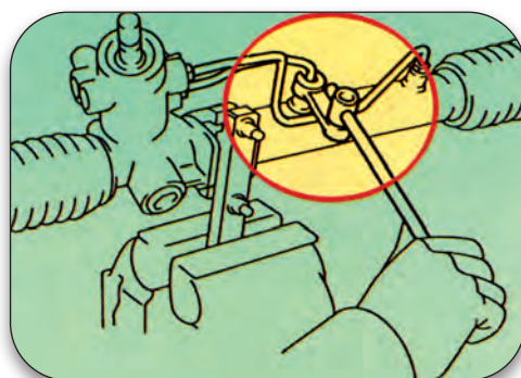
Σχήμα 2.36: Αφαίρεση σωληνώσεων υψηλής πίεσης.
