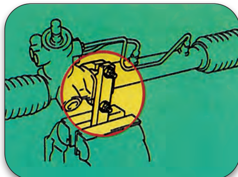
Σχήμα 2.35: Στήριξη κρεμαγιέρας με ειδικό εργαλείο.
