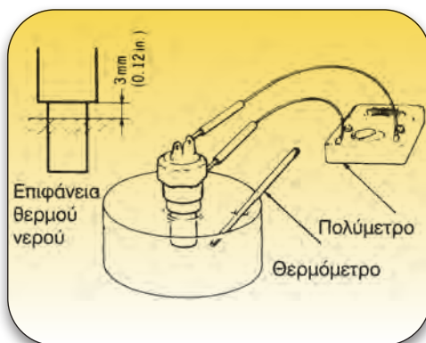
Σχήμα 5.7: Έλεγχος του στοιχείου ένδειξης (θερμίστορ).
