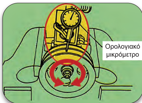
Σχήμα 2.94: Έλεγχος ακτινικής απόκλισης αυλακών τροχαλίας.
