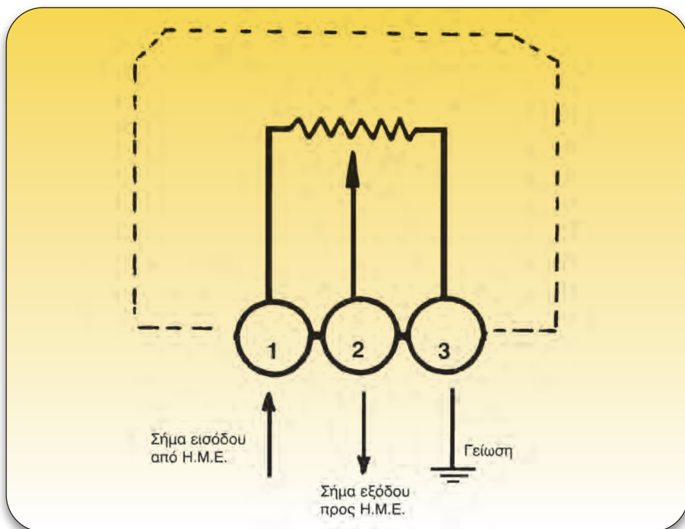
Σχήμα 2.100: Έλεγχος του αισθητήρα γωνίας περιστροφής.
