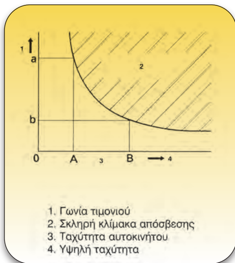
Σχήμα 3.12: Γράφημα σχέσης αισθητήρα γωνίας τιμονιού - αισθητήρα ταχύτητας και απόσβεσης.
