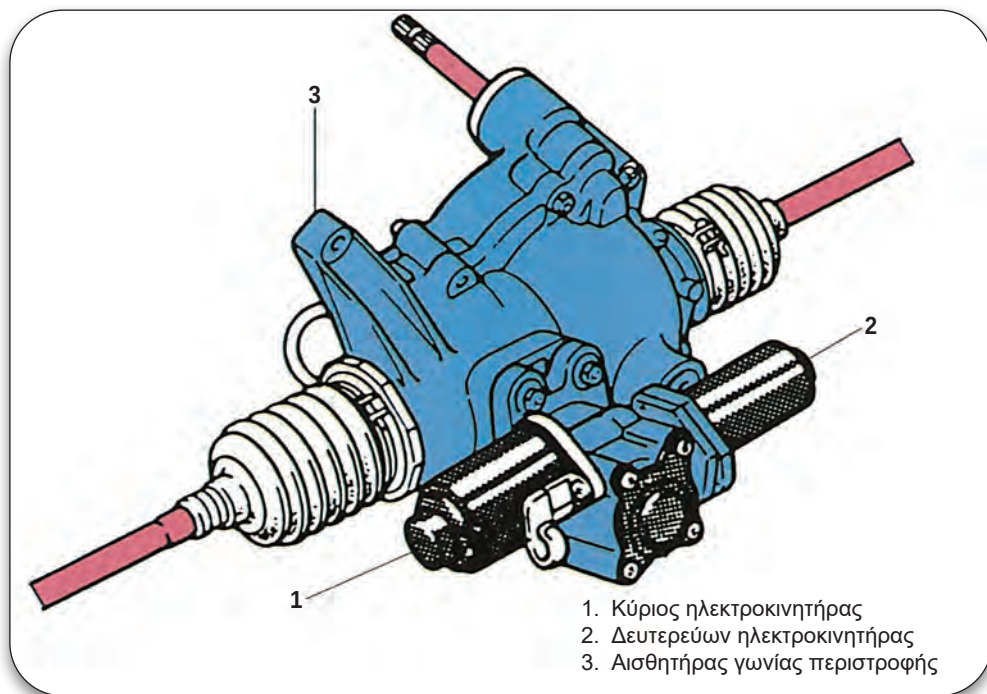
Σχήμα 2.101: Ενεργοποιητές.
