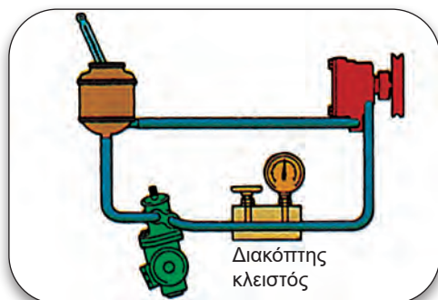
Σχήμα 2.21: Έλεγχος της πίεσης με κλειστό διακόπτη στο υδραυλικό κύκλωμα.
