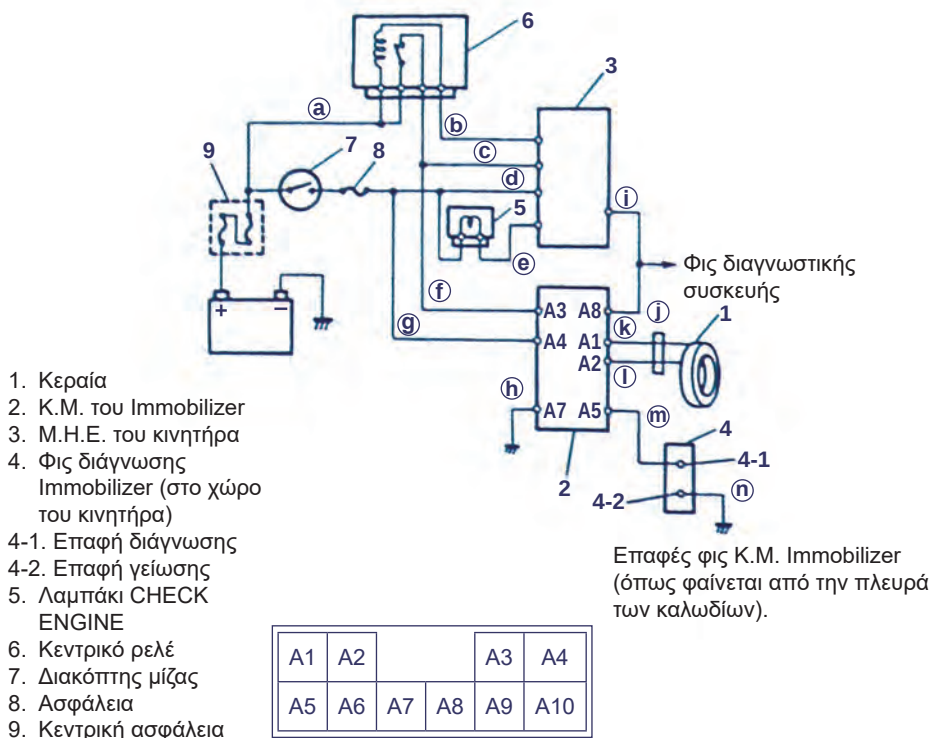
Σχήμα 8.2: Ηλεκτρολογικό Διάγραμμα κυκλώματος Immobilizer.
