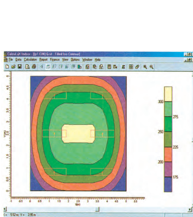
Σχήμα 8γ. Η ένταση φωτισμού της επιφάνειας εργασίας με ισοδυναμικές γραμμές και χρωματικό κωδικό
