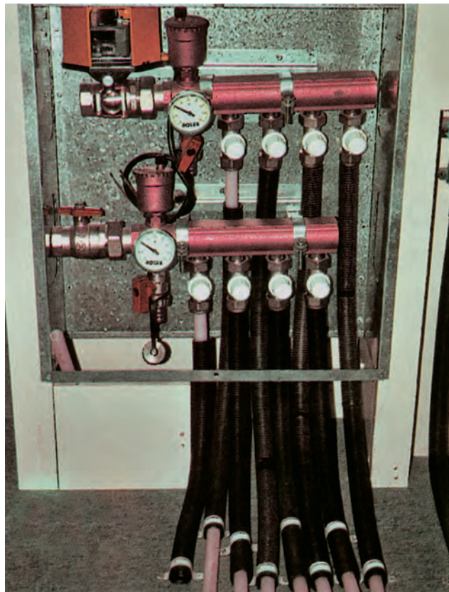
Πίνακας αυτονομίας
