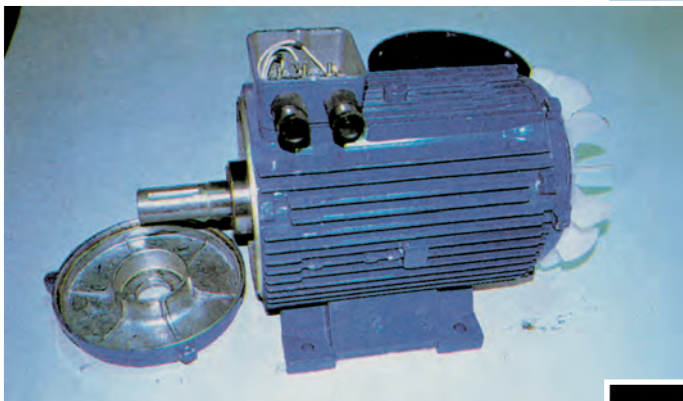
Κινητήρας μετά την αφαίρεση πλαινίου καπακιού
