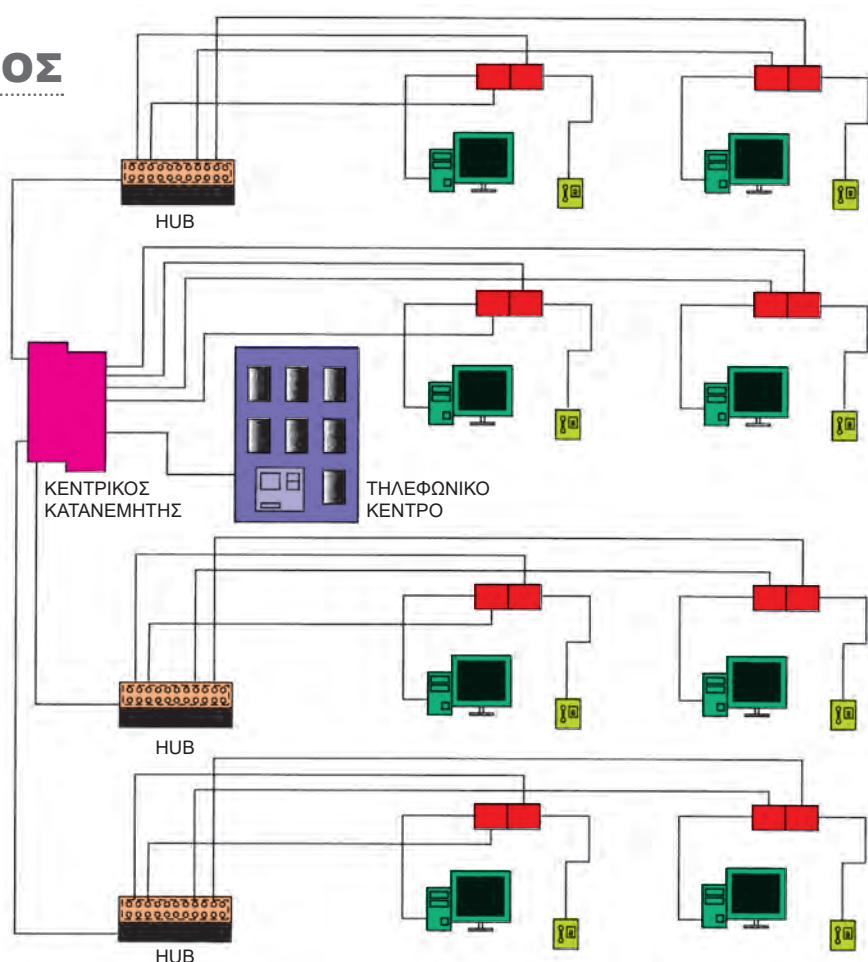
Ιεραρχία δικτύου δομημένης καλωδίωσης
