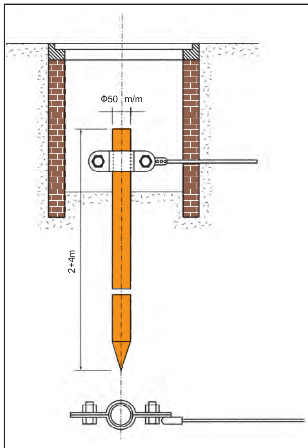
Ηλεκτρόδια γειώσεων
