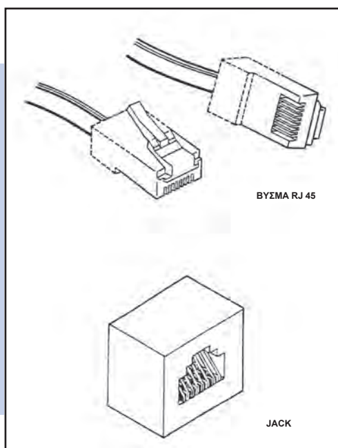
Jack και βύσμα RJ 45, 4 ζευγών όπως εικονίζεται στο πρότυπο ISO 8877Q: 1987
