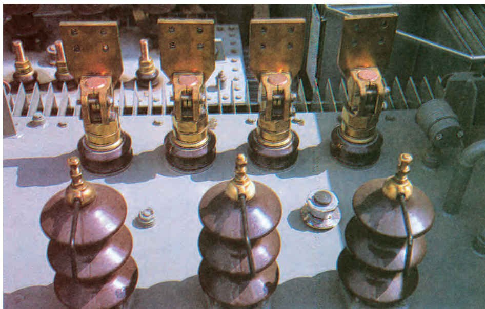
Ακροδέκτες τριφασικού Μ/Σ τρίγωνο - αστέρας (Δ - Υ)
