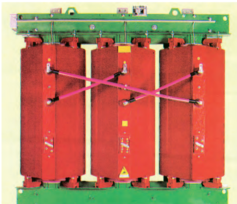
Τριφασικός Μ/Σ με χυτετή ρητίνη
