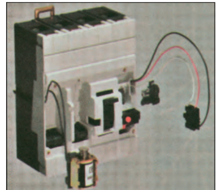
Βοηθητικές επαφές και πηνίο ελλείψεως τάσης
