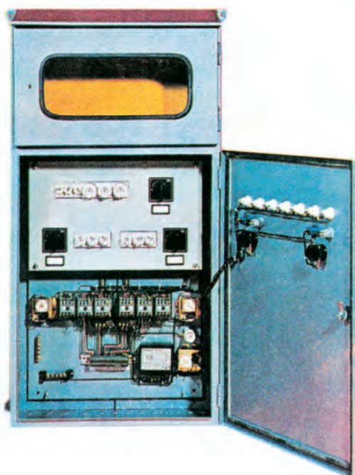
Πίνακας κίνησης
