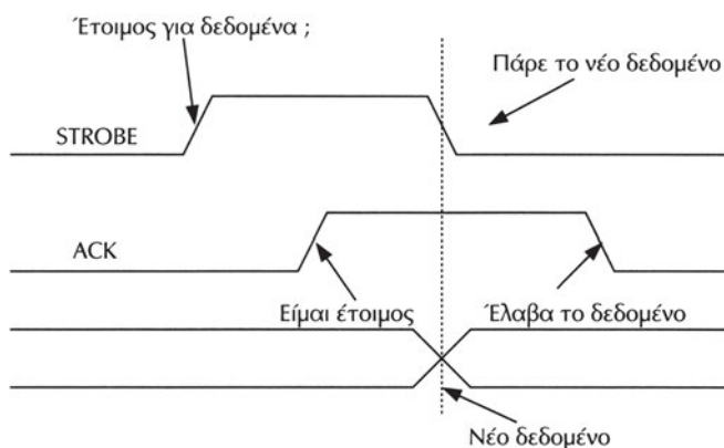
Σχήμα 3.9.4 Διπλή χειραψία
