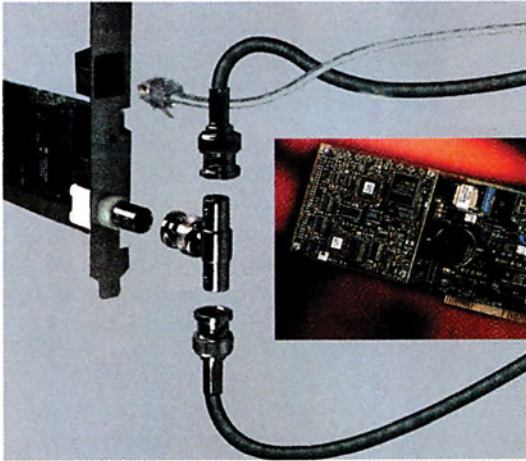
Σχήμα 5.3.5 Κάρτα δικτύου
