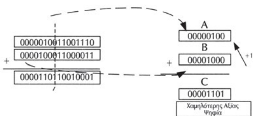
Σχήμα 3.3.4 Πρόσθεση με 8-bit καταχωρητές. Βήμα 2°
