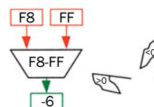
Σχήμα 3.2.7 Η ALU εκτελεί την αφαίρεση 248-254
