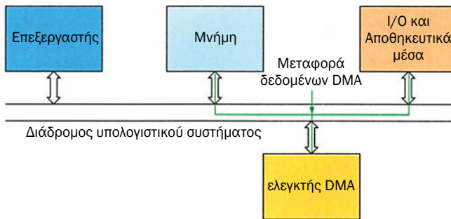
Σχήμα 3.8.4 Ελεγκτής DMA
