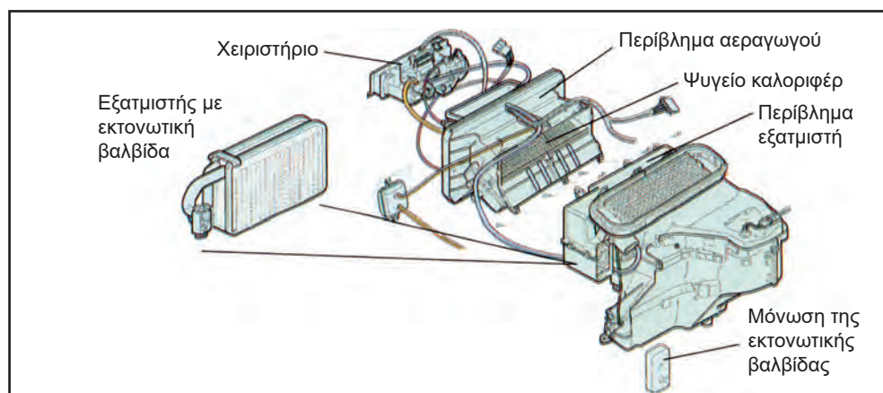
Σχήμα 6.12: Εβαπορέτα κλιματισμού.
