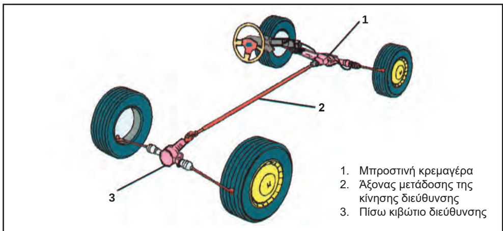
Σχήμα: 2.26: Μηχανικό σύστημα ενεργητικής τετραδιεύθυνσης.
