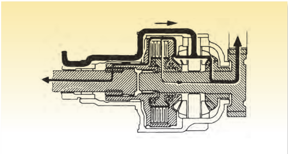
Σχήμα 1.85: Λειτουργία του συνεκτικού συμπλέκτη σε στροφή του αυτοκινήτου με χαμηλή ταχύτητα.
