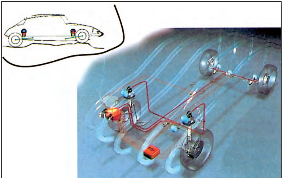
Σχήμα 3.8: Η εξέλιξη της υδροπνευματικής ανάρτησης.
