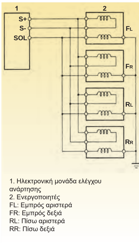
Σχήμα 3.20: Σύνδεση των ενεργοποιητών με την ηλεκτρονική μονάδα ελέγχου της ανάρτησης.
