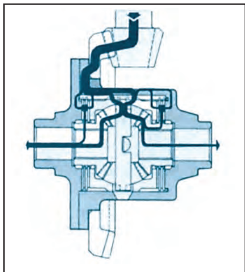
Σχήμα 1.63: Λειτουργία του μπλοκέ διαφορικού σε στρόφη.
