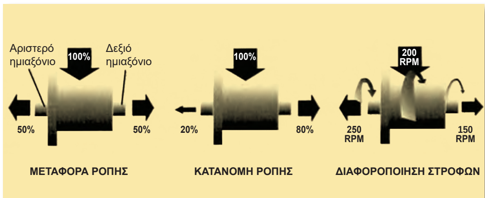
Σχήμα 1.68: Οι τρεις φάσεις λειτουργίας στο διαφορικό Torsen. Το διαφορικό Torsen μπορεί να μεταφέρει τη ροπή, να κατανομεί τη ροπή και να διαφοροποιήσει τις στροφές των κινητήριων τροχών (λειτουργία διαφορικού).
