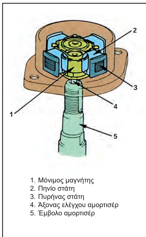
Σχήμα 3.18: Δομή ενεργοποιητή.
