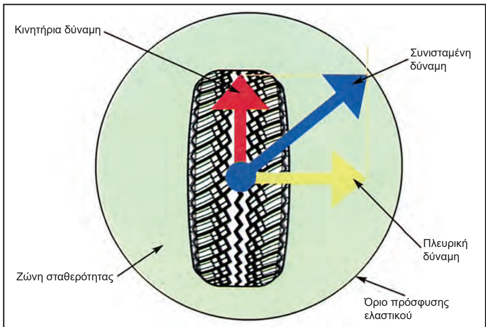
Σχήμα 4.3: Κύκλος ισορροπίας δυνάμεων ή κύκλος Kammt.
