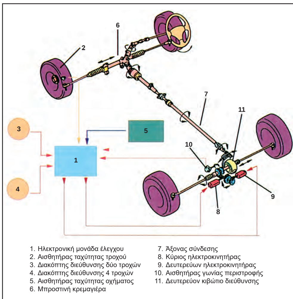
Σχήμα 2.32: Ηλεκτρονικά - μηχανικά ελεγχόμενο σύστημα τετραδιεύθυνσης.
