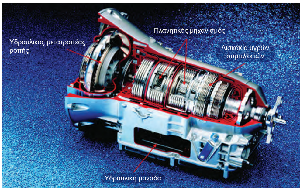
Σχήμα 1.2: Κλασσικό Αυτόματο κιβώτιο (Mercedes).
