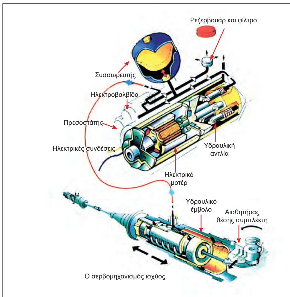
Σχήμα 1.11: Υδραυλική μονάδα ενεργοποίησης συμπλέκτη - σερβομηχανισμός.
