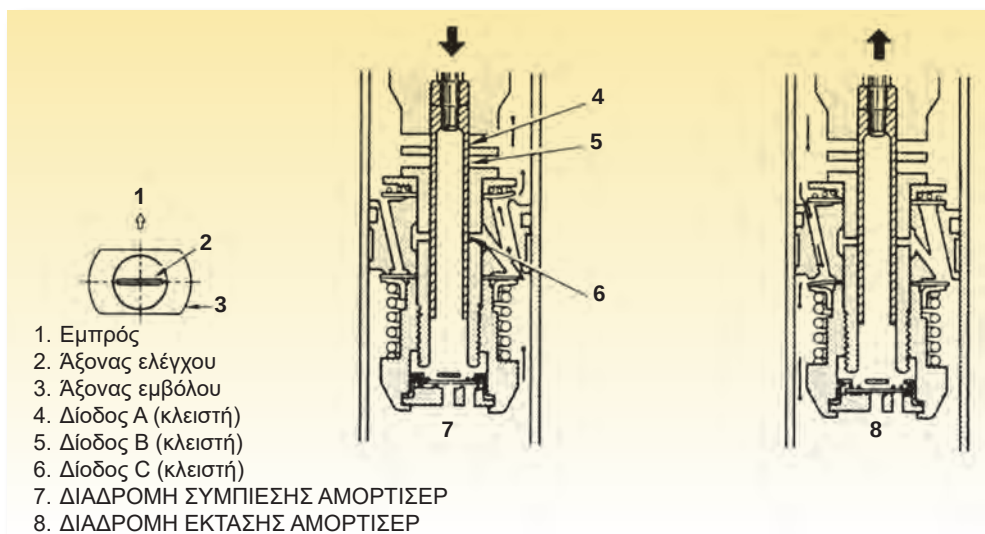
Σχήμα 3.27: Διαδρομή του λαδιού του αμορτισέρ από τις πρόσθετες διόδους όταν έχει επιλεγεί η σκληρή κλίμακα απόσβεσης.
