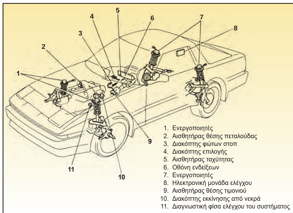
Σχήμα 3.16: Θέση εξαρτημάτων του συστήματος της ηλεκτρονικά ελεγχόμενης ανάρτησης.
