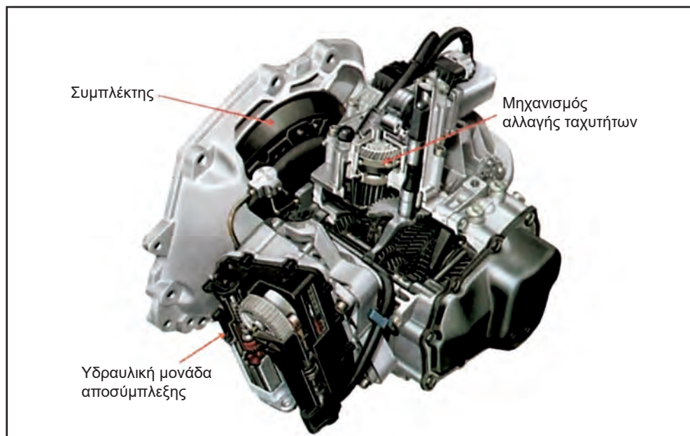
Σχήμα 1.16: Opel Easytronic.
