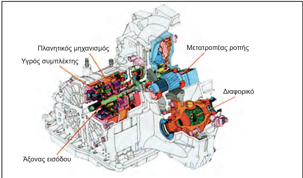
Σχήμα 1.33: Αυτόματο κιβώτιο σε τομή (μπροστινή κίνηση).
