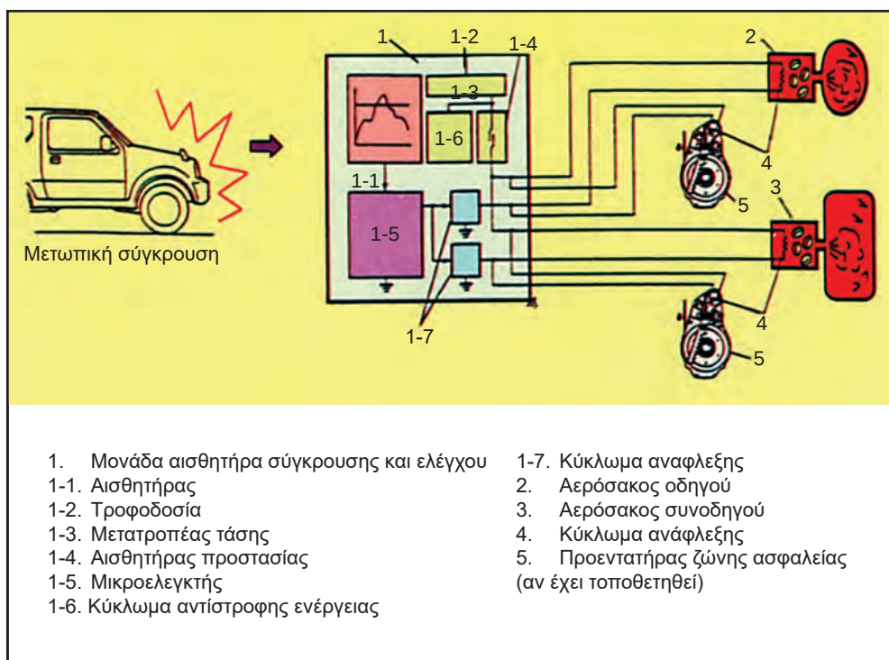
Σχήμα 7.7: Λειτουργία του συστήματος του αερόσακου σε σύγκρουση.
