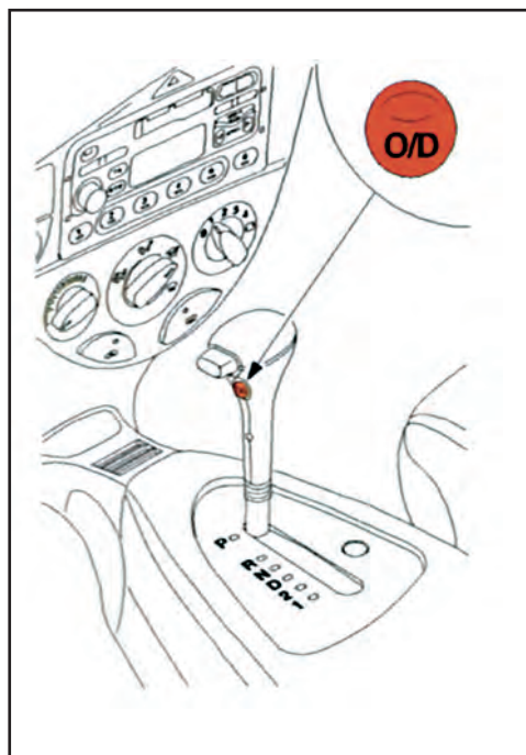
Σχήμα 1.34: Επιλογέας ταχυτήτων αυτομάτου κιβωτίου με O/D και ενδεικτική λυχνία.
