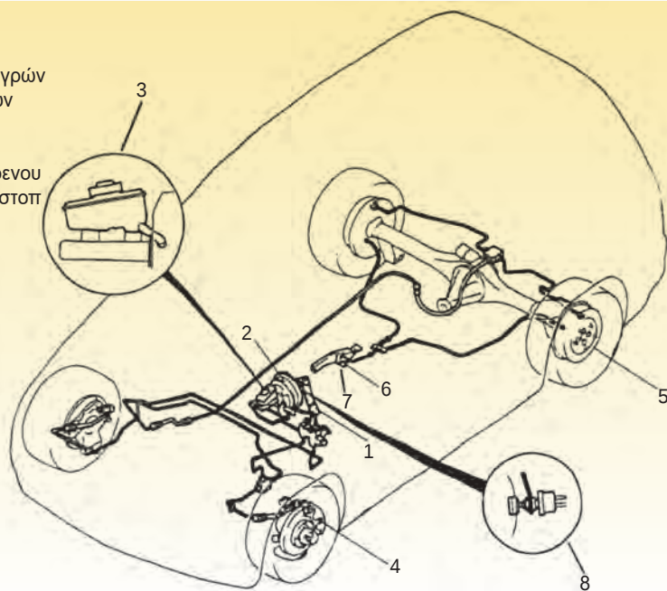
Σχήμα 4.1: Διάγραμμα κυκλώματος συμβατικού υδραυλικού συστήματος πέδησης.
