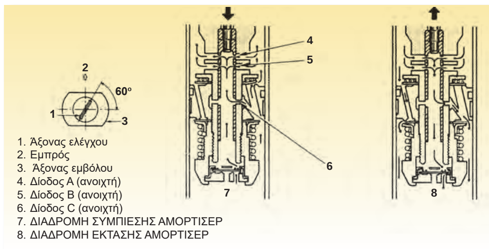
Σχήμα 3.25: Διαδρομή του λαδιού του αμορτισέρ από τις πρόσθετες δίοδους όταν έχει επιλεγεί η μαλακή κλίμακα απόσβεσης.
