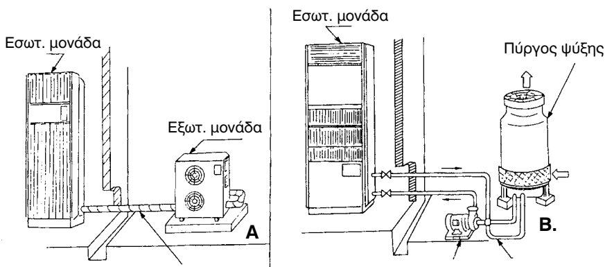
Σχήμα 1-6. (Α) Ημικεντρική μονάδα διαιρούμενου τύπου (Split Type) με αερόψυκτο συμπυκνωτή.
