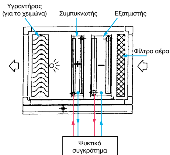
Σχήμα 9-13: Παράδειγμα συστήματος ελέγχου της υγρασίας του προκλιματιζόμενου αέρα
