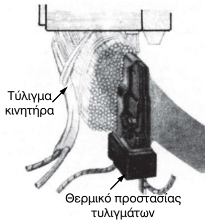
Σχήμα 10-2. Θερμικό αυτόματος προστασίας του ηλεκτροκινητήρα από υπερένταση που τοποθετείται στα τυλίγματα του ηλεκτροκινητήρα.
