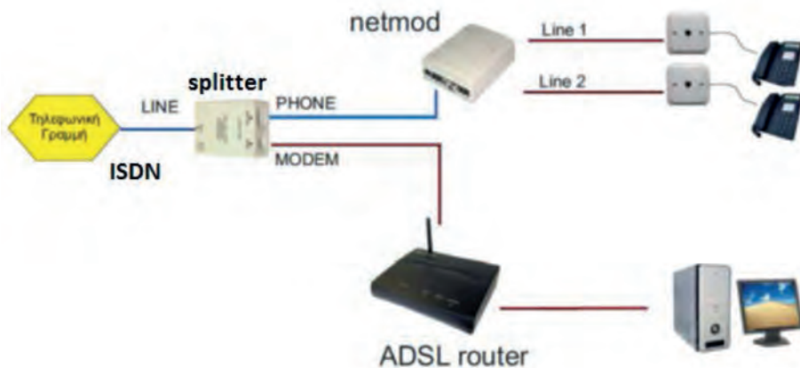
Σχήμα 5.1.4.2.δ. Σύνδεση ADSL σε γραμμή ISDN με χρήση διαχωριστή σήματος (splitter-based) (Πηγή: http://users.sch.gr//iliaslamprou/images/stories/askiseis_electrikwn_egkatasasewn/phones_and_lan_ins_tallation_diagram.pdf )
