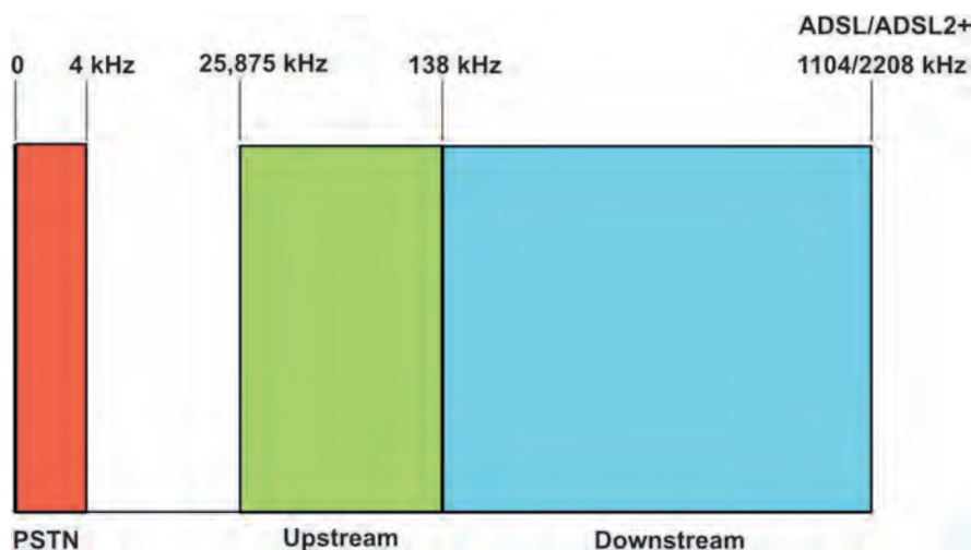
Σχήμα 5.1.4.β: Χρήση συχνοτήτων PSTN
