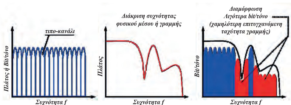
Εικόνα Π.3.α: Διαμόρφωση Διακριτής Πολυτονίας (DMT)
