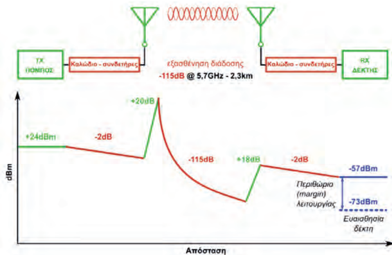
Εικόνα Π.2.α: Προϋπολογισμός ζεύξης (Link budget)
