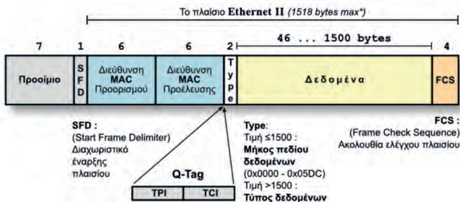
Εικόνα 2.4.2.β: Δομή πλαισίου Ethernet
