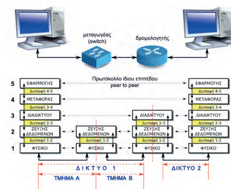
Εικόνα 3.1.α: Δίκτυα και Διαδίκτυο
