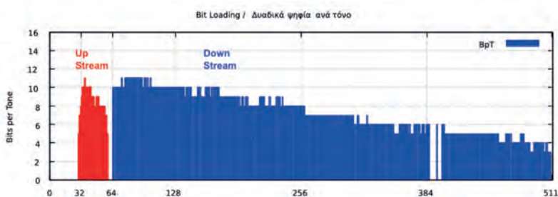
Εικόνα 2.3.β: Μετάδοση σε γραμμή ADSL (over ISDN) - 512 τόνοι/κανάλια των 4,3125kHz.
