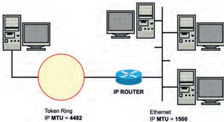
Εικόνα 3.2.β: Δίκτυα με διαφορετικό MTU
