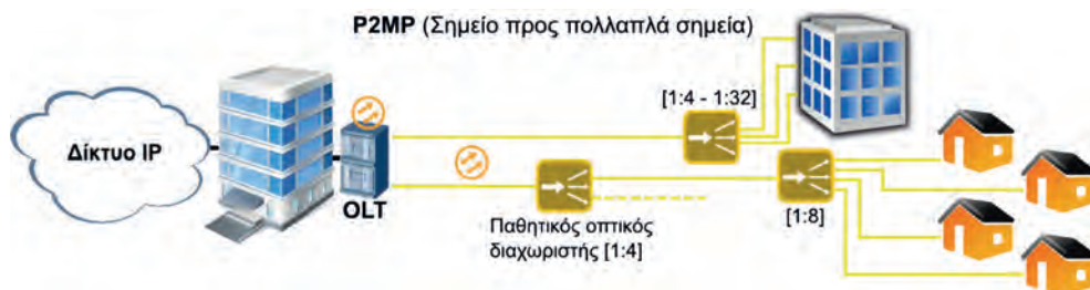
Εικόνα 5.2.δ: Αρχιτεκτονική «σημείο προς σημεία»
