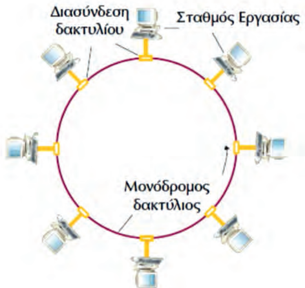
Σχήμα Π.1.δ. Δίκτυο δακτύλιου με κουπόνι
