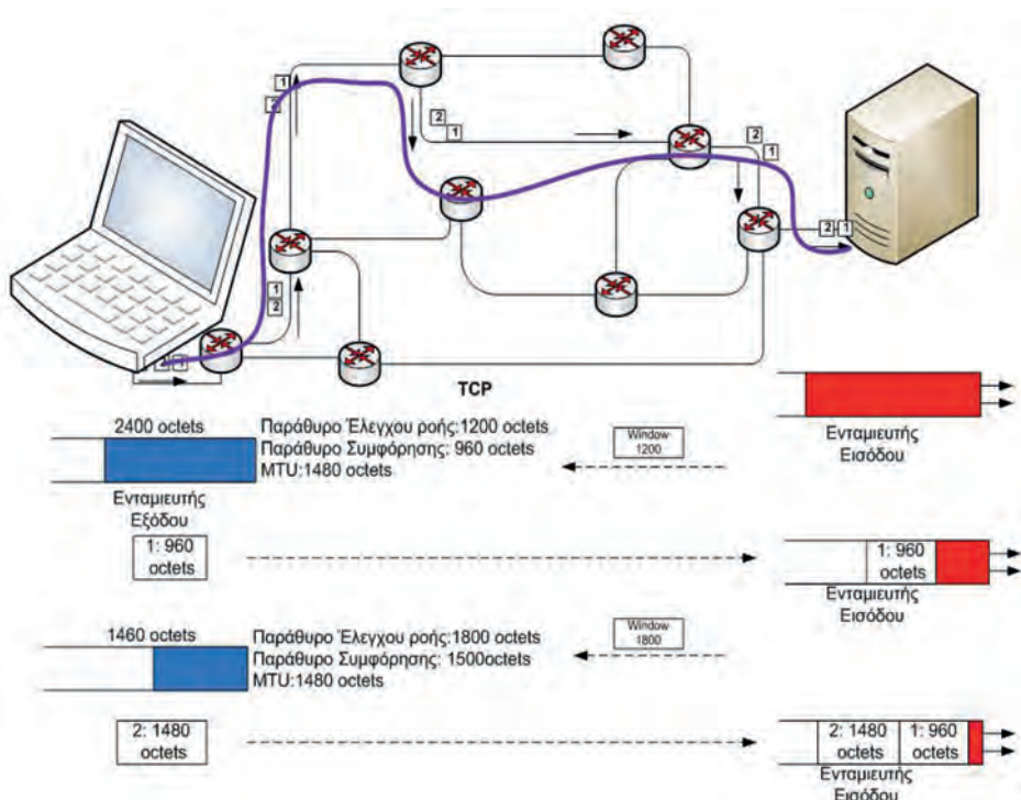
Εικόνα 4.1.4.β: Εγκατάσταση νέας Σύνδεσης με τριμερή χειραψία.
