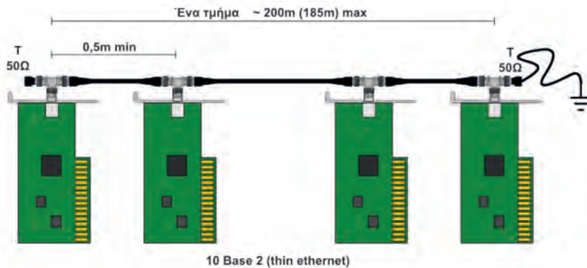
Εικόνα 2.4.1.γ: Δίκτυο Thin Ethernet (10Base2).
