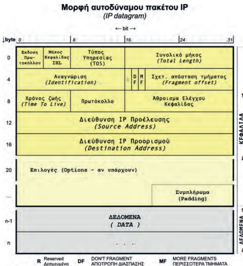
Εικόνα 3.2.α: Το αυτοδύναμο πακέτο IP (IP datagram)
