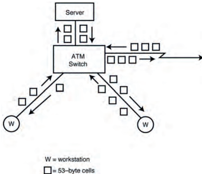
Σχήμα 2.6.β: Μεταφορά κυψελίδων ATM (cells)
