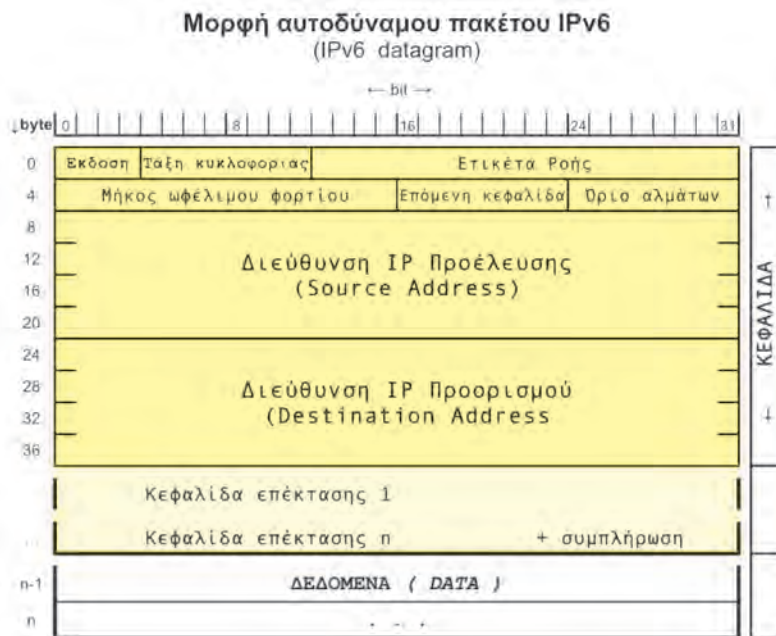
Εικόνα 3.5.α: Μορφή αυτοδύναμου πακέτου IPv6
