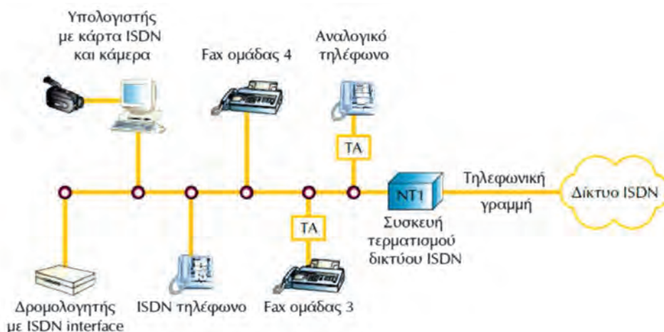
Σχήμα 5.1.3.β. Ο εξοπλισμός του ISDN
