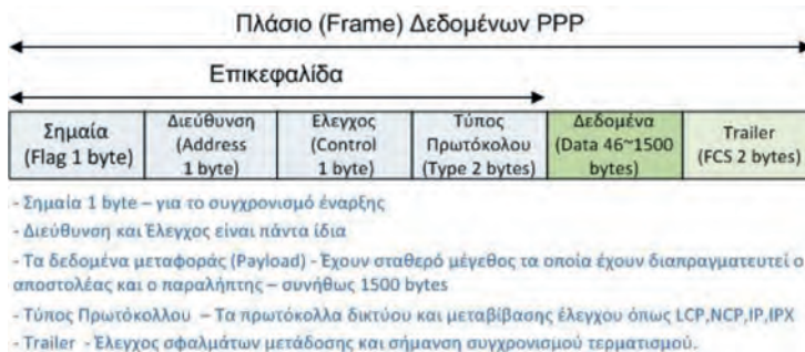
Εικόνα 2.7.β: Πλάσιο PPP
