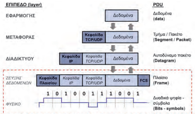
Εικόνα 1.3.α: Ενθυλάκωση
