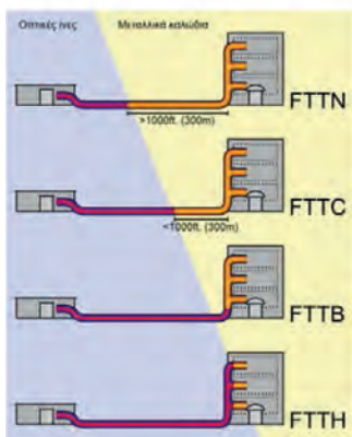
Εικόνα 5.2.α: Τεχνολογίες FttX (πηγή: wikipedia)
