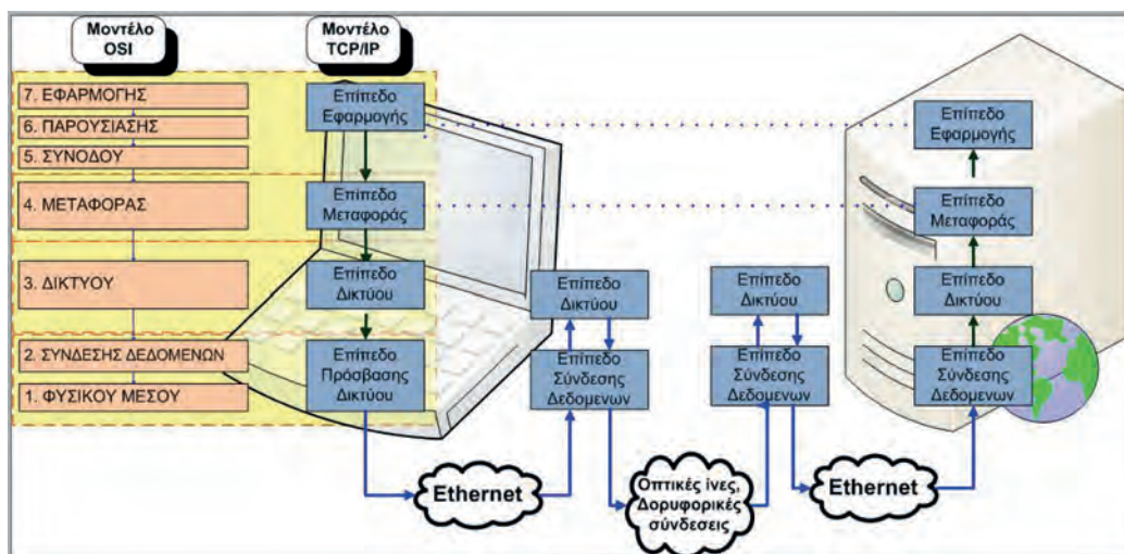
Εικόνα 4.1.α: OSI – TCP Διαστρωμάτωση
