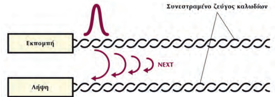
Εικόνα 2.4.1.ι: Παραδιαφωνία NEXT (Near End CrossTalk)
