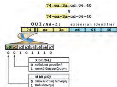
Εικόνα 2.4.2.α: Δομή διεύθυνσης MAC στο Ethernet
