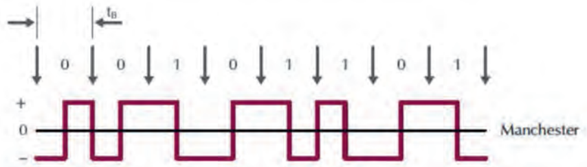
Σχήμα 2.2.1.α: Κωδικοποίηση Manchester.
