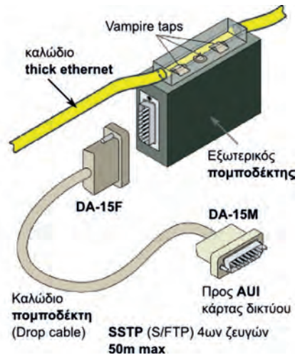
Εικόνα 2.4.1.β: Εξ. πομποδέκτης Thick Ethernet.
