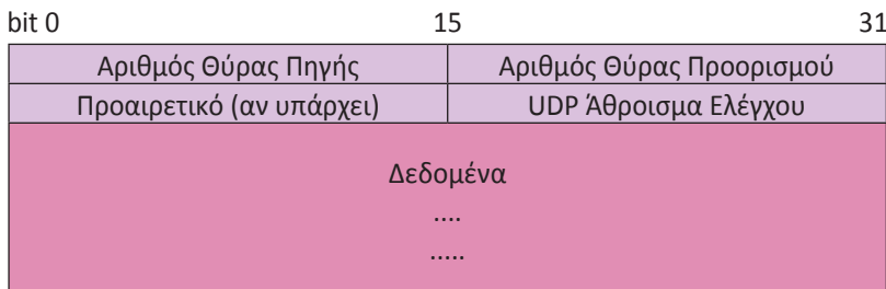
Εικόνα 4.1.2.α: Πεδία της επικεφαλίδας ενός UDP τμήματος.
