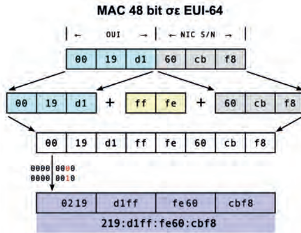
Εικόνα 3.5.1.α: Μεταγραφή διεύθυνσης MAC 48 bit σε EUI-64
