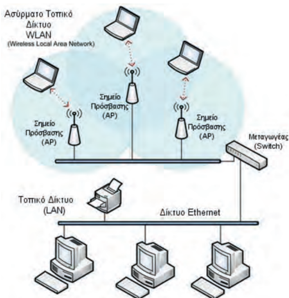
Σχήμα 2.5.β: Ασύρματο τοπικό δίκτυο συνδεδεόμενο με ενσύρματο τοπικό δίκτυο (Προσαρμοσμένη από Πηγή: http://bb-smartworx.com/make-tablets-smart-phones-smarter-add-serial-capability-seriously-remote-data/ )
