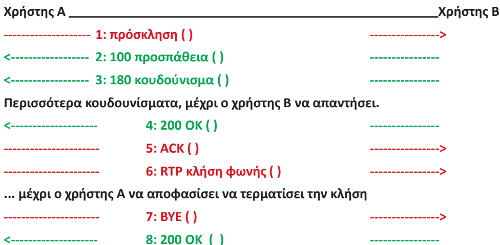
Σχήμα Π.5.α: Βήματα SIP κλήσης
