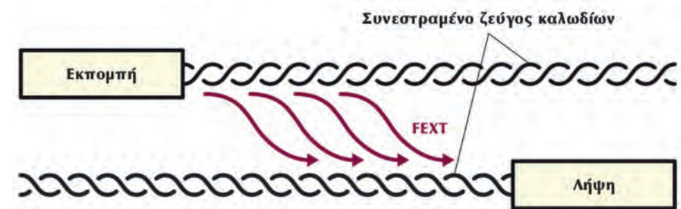
Εικόνα 2.4.1.κ: Παραδιαφωνία FEXT (Far End CrossTalk).
