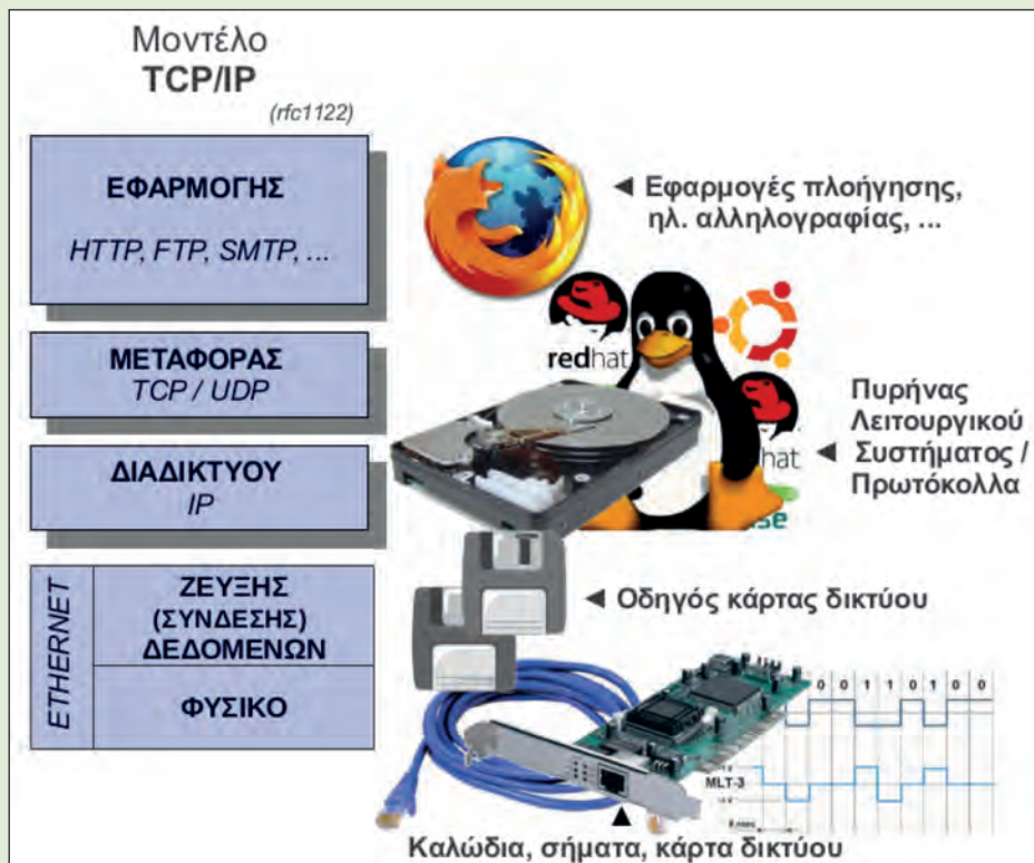
Εικόνα 1.2.2.β: Επίπεδα TCP/IP και αντίστοιχο Υλικό - Λογισμικό
