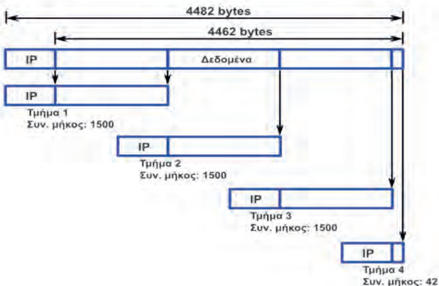
Εικόνα 3.2.γ: Κατάτμηση αυτοδύναμου πακέτου IPv4
