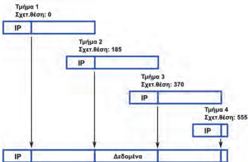
Εικόνα 3.2.δ: Επανασύνθεση κατατμημένου πακέτου IPv4
