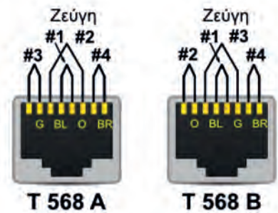
Εικόνα 2.4.1.α: Συρμάτωση
