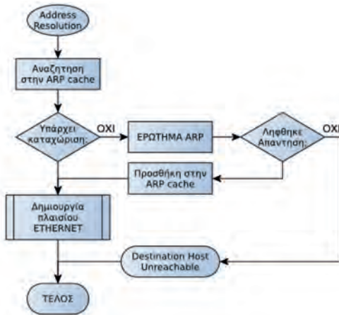
Εικόνα 3.3.ε: Ανάλυση διευθύνσεων ARP
