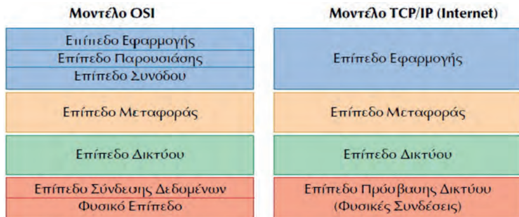
Σχήμα 2.1.α: Μοντέλα OSI και TCP/IP.
