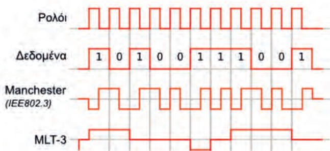
Εικόνα 2.4.1.κζ: Κωδικοποίηση Manchester, MLT-3
