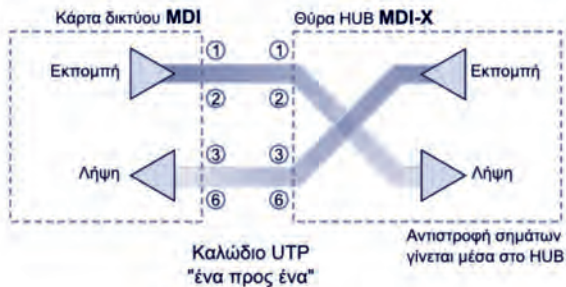
Εικόνα 2.4.3.α: MDI/MDI-X
