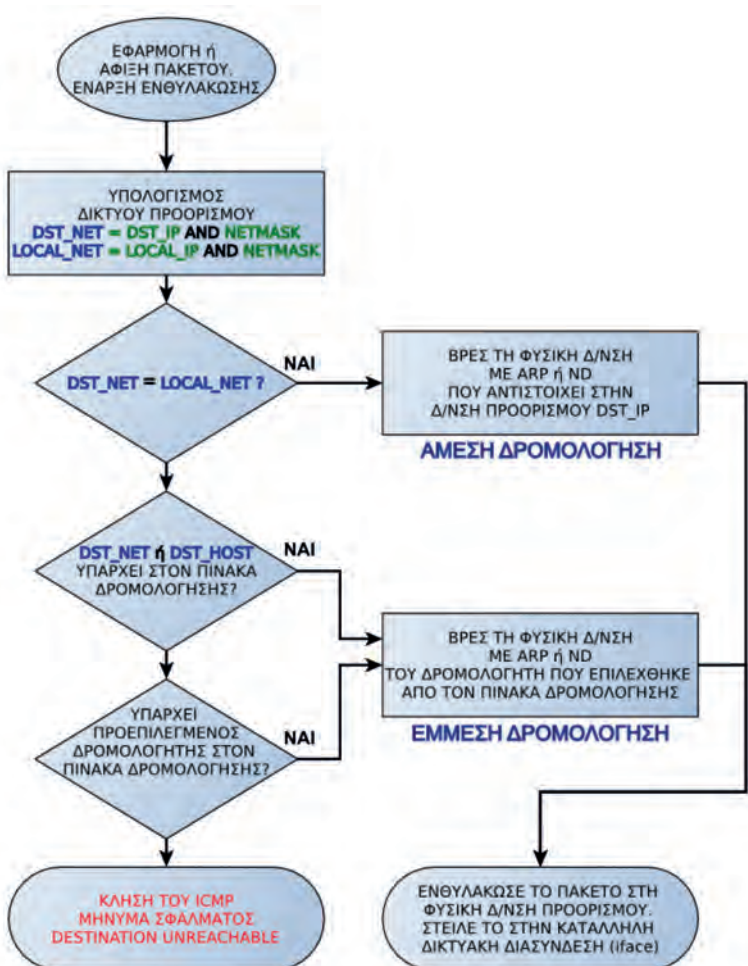
Σχήμα 3.6.1.α: Διαδικασία δρομολόγησης αυτοδύναμου πακέτου
