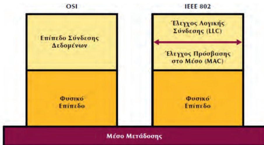
Σχήμα 2.2.α: Σχέση μοντέλων αναφοράς OSI και IEEE 8.
