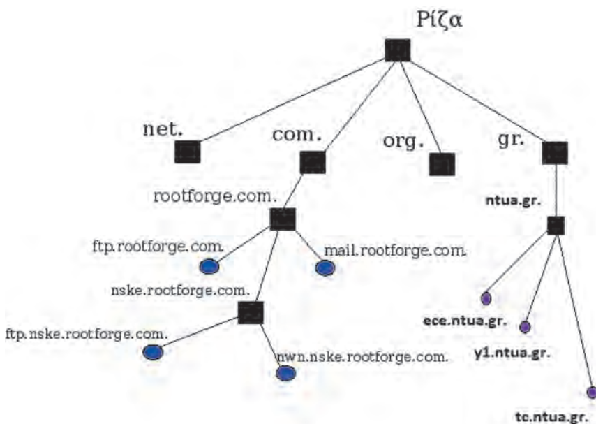
Σχήμα 6.1.1.β: Ιεραρχική οργάνωση χώρου ονομάτων DNS
