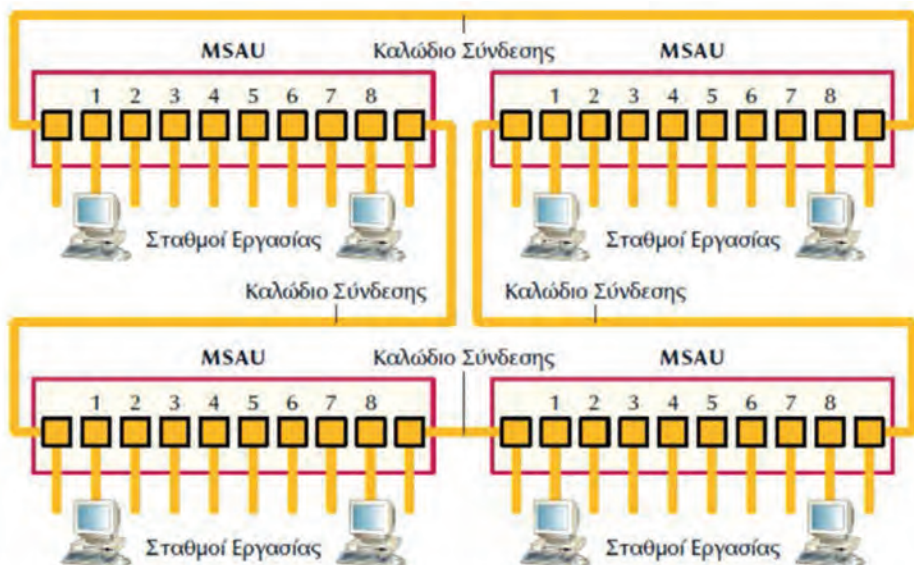
Σχήμα Π.1.γ: Σύνδεση των MSAU για τη δημιουργία ενός μεγάλου δακτυλίου με κουπόνι
