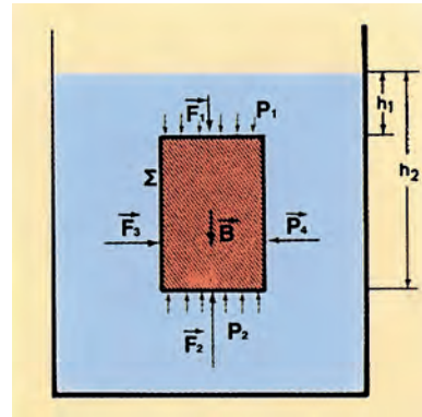
Εικόνα 7.23: Υπολογισμός της άνωσης
