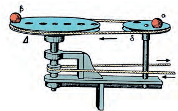
Εικόνα 6.3: Περιφερειακή μετάδοση κίνησης
