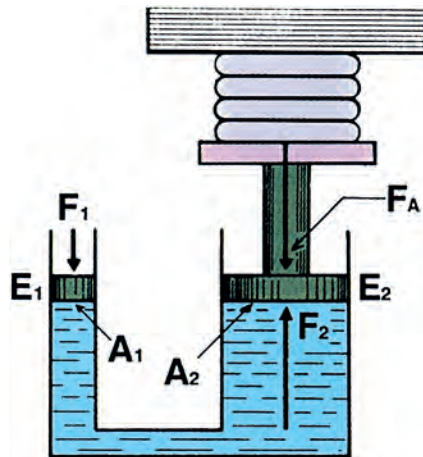
Εικόνα 7.13 Υδραυλικό πιεστήριο
