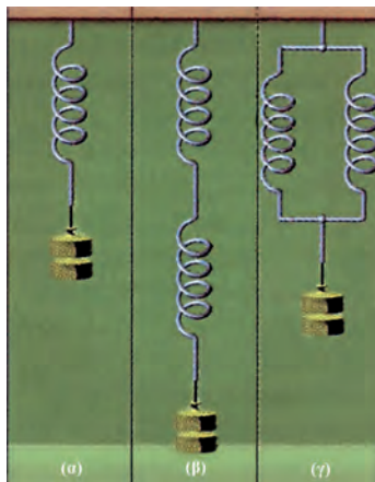
Εικόνα 2.18 Σύστημα ελατηρίων
