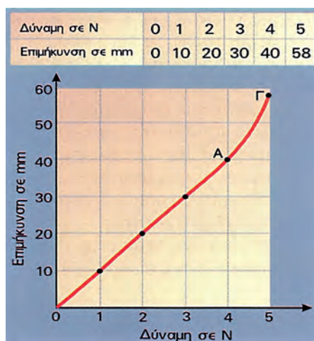
Εικόνα 2.17 Χαρακτηριστική ελατηρίου
