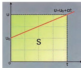
Εικόνα 4.34 Διάγραμμα για την απόδειξη της σχέσης s=f(t) στην ευθύγραμμη ομαλά επιταχυνόμενη κίνηση
