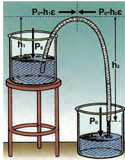
Εικόνα 7.32: Ο σίφωνας
