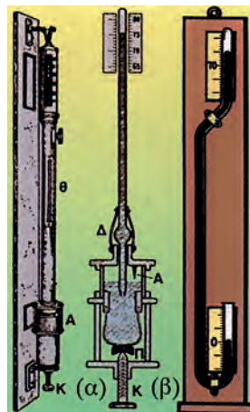
Εικόνα 7.36: Βαρόμετρα
