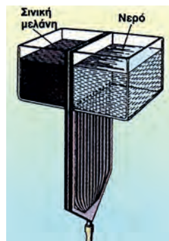
Εικόνα 7.39: Γραμμές ροής για δύο υγρά
