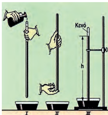
Εικόνα 7.27: Προσεγγίζοντας το πείραμα Toricelli
