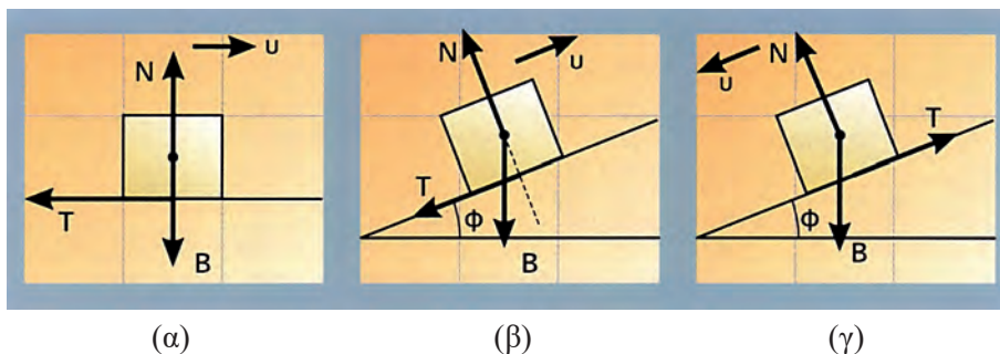
Εικόνα 5.12: Έργο τριβής
