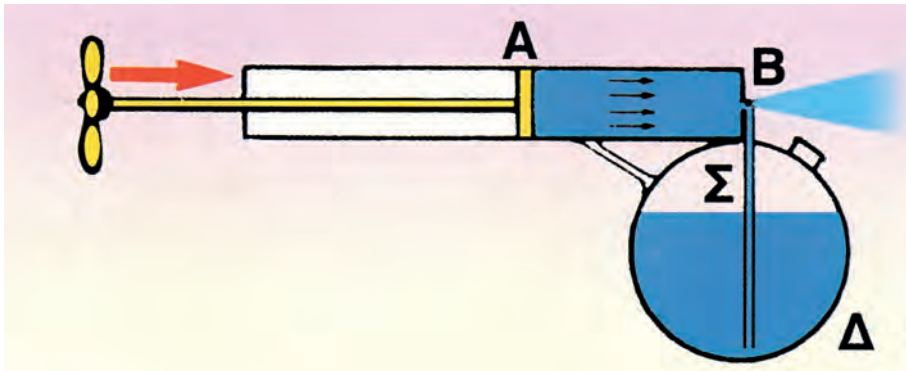
Εικόνα 7.44 (γ) Ψεκαστήρας
