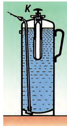
Εικόνα 7.34: Ο πυροσβεστήρας
