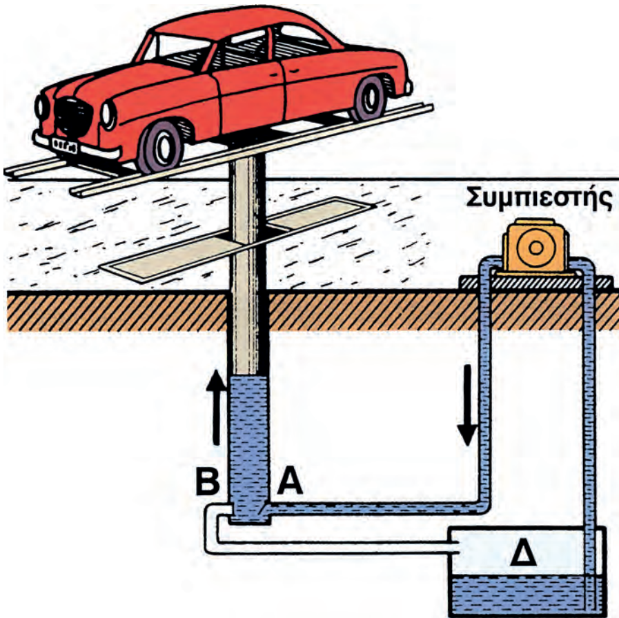
Εικόνα 7.14: Υδραυλικός ανυψωτήρας
