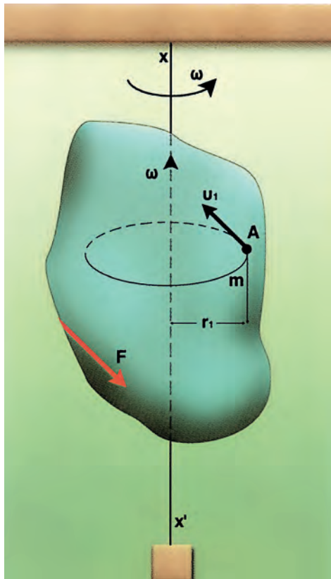
Εικόνα 6.11: Περιστροφή στερεού
