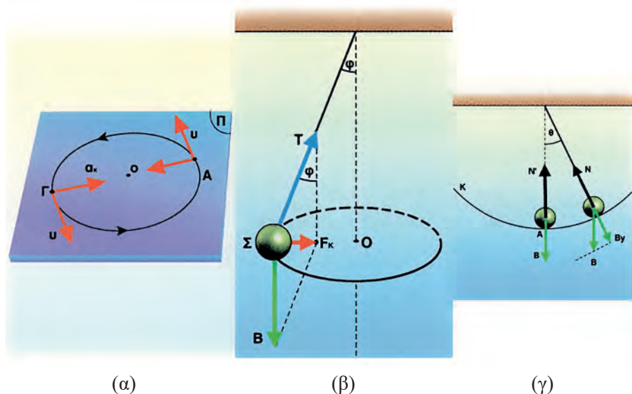
Εικόνα 6.2: Η κεντρομόλος δύναμη είναι η ακτινική συνισταμένη των δυνάμεων που ασκούνται στο σώμα.
