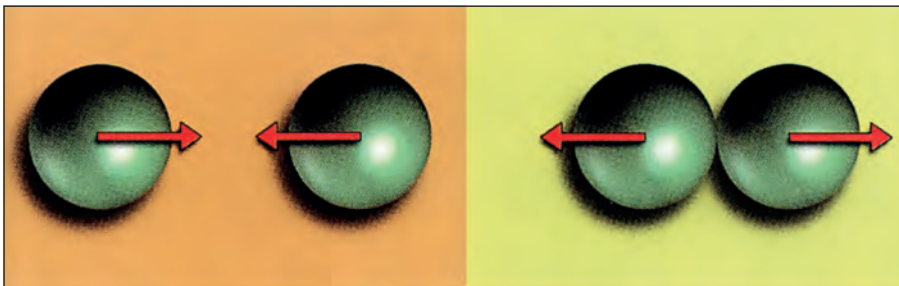
Εικόνα 2.10 Ελκτικές και απωστικές δυνάμεις μεταξύ των μορίων
