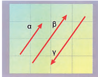
Εικόνα 1.11 Συγγραμμικά διανύσματα
