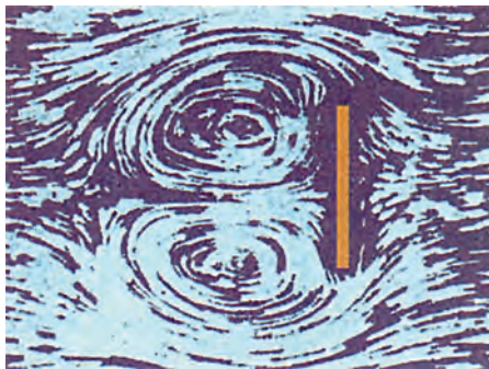
Εικόνα 7.50: Πραγματική ροή γύρω από πλάκα και σφαίρα
