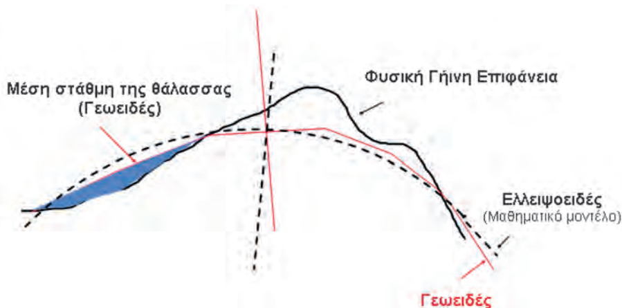
Εικόνα 6: Γεωειδές, ελλειψοειδές και επιφάνεια της γης
