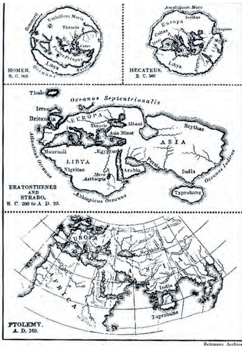
Εικόνα 3: Αντίληψη των αρχαίων Ελλήνων για την γη.
