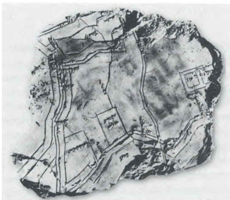
Εικόνα 2: Τοπογραφικός χάρτης της πόλης Νιμπούρ
