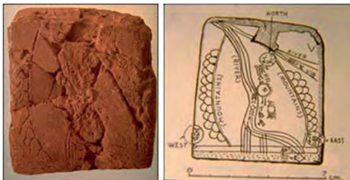
Εικόνα 1: Χάρτης Ακκαντιαν (Akkadian), 2500π.Χ.
