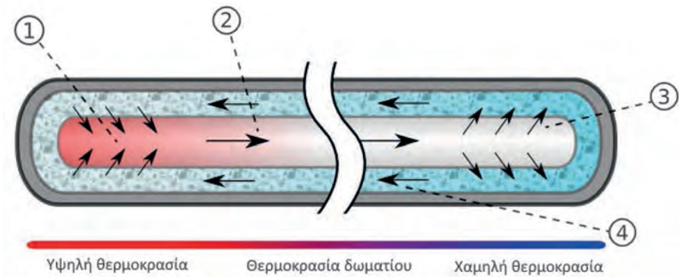
Εικόνα 2.8: Αρχή λειτουργίας θερμοαγωγού
