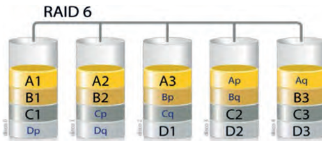
Εικόνα 3.6. Συστοιχία RAID 6.
