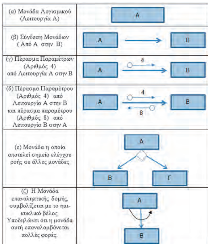
Σχήμα 4.1: Συμβολισμοί Διαγράμματος Δομής
