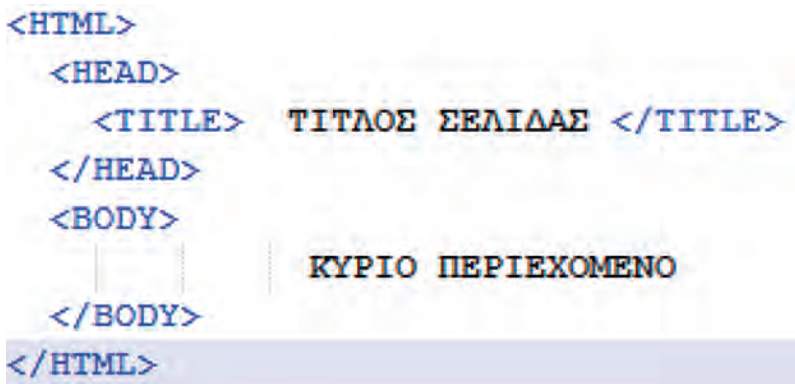
Σχήμα 5.7: Βασική δομή αρχείου HTML
