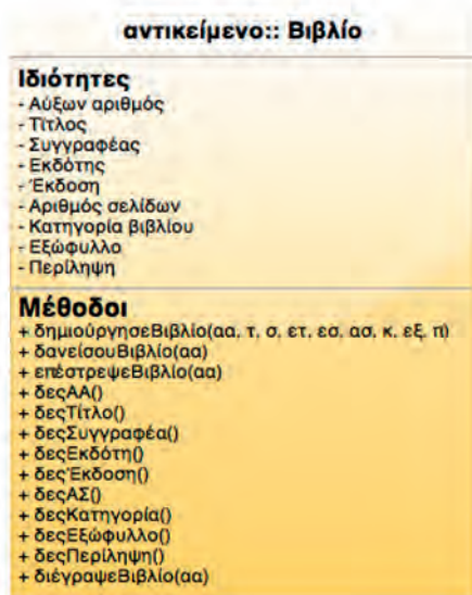
Σχήμα 3.12: Το αντικείμενο βιβλίο: Ιδιότητες και Μέθοδοι
