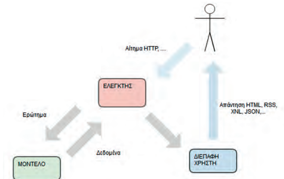
Σχήμα 5.25: Ένα βασικό MVC αίτημα
