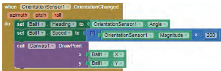
Εικόνα 17.3.1. Αισθητήρας θέσης.
