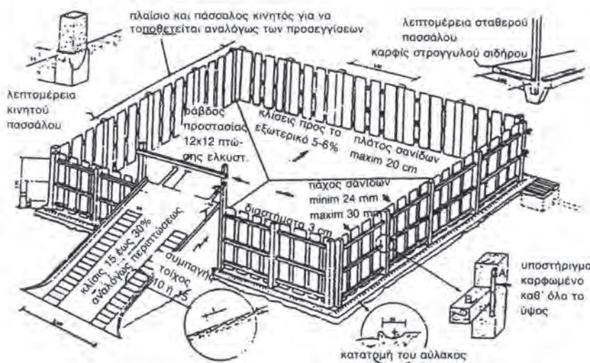
Εικόνα 3.34. Διάταξη κοπροσωρού ή ημιστερεών αποβλήτων
