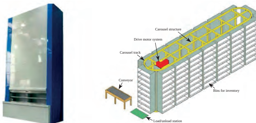
Εικόνες 9.23 και 9.24: Κάθετα και οριζόντια carousel
