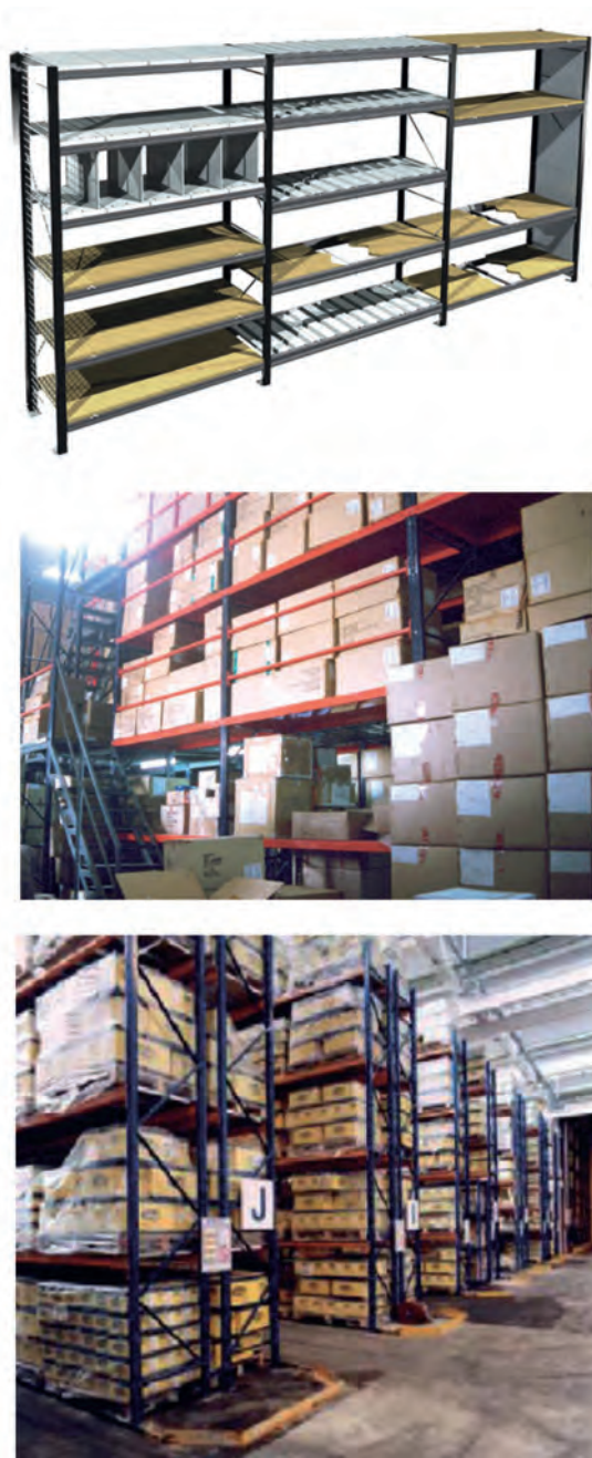
Εικόνες 9.7, 9.8 και 9.9: Παραδείγματα ραφιών για αποθήκευση προϊόντων διαφορετικού βάρους
