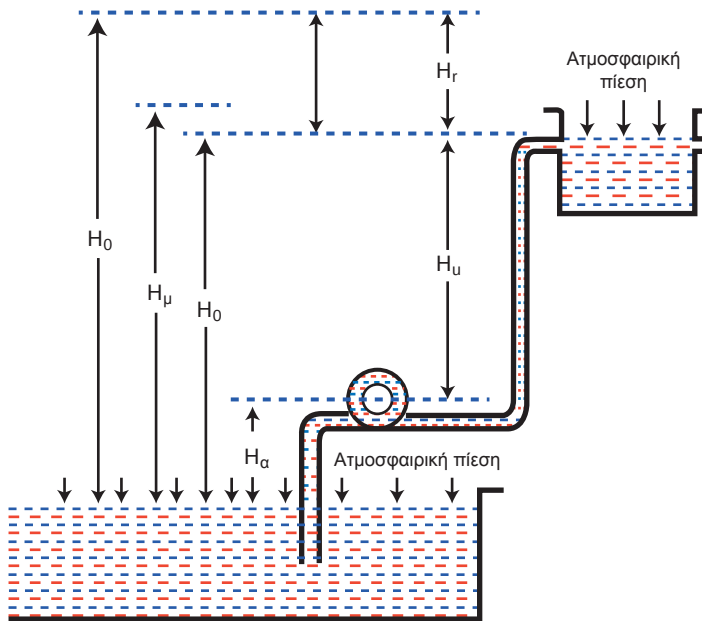
Σχήμα 10.6: Ύψη αντλίας
