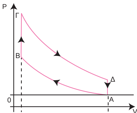
Σχήμα 3.11.β. Θεωρητικός θερμοδυναμικός κύκλος έργου βενζινομηχανής.
