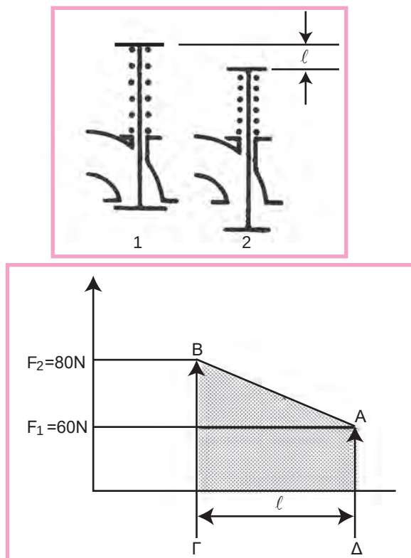
Σχήμα 4.4.1.δ. Διάγραμμα ελατηρίου
