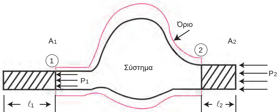
Σχήμα 4.6.α. Ανοικτό σύστημα σταθερής ροής - έργο ροής
