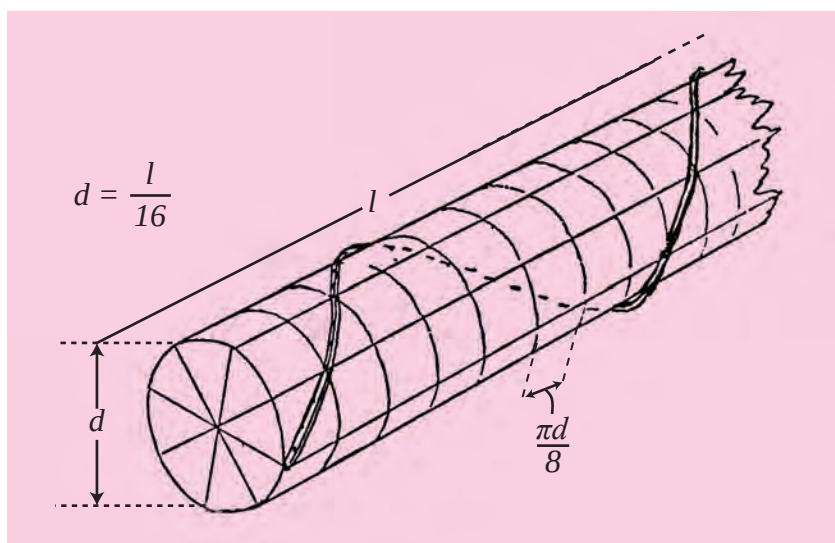
Σχήμα 10.2: Τεχνικά χαρακτηριστικά για την κατασκευή του κοχλίου.
