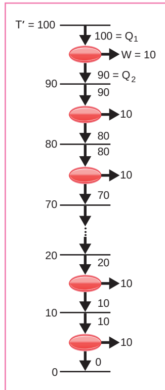
Σχήμα 8.2.2.α Κλίμακα θερμοκρασιών Kelvin
