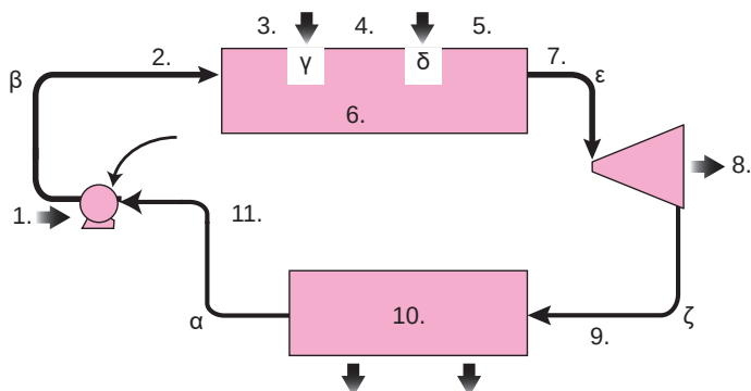
Σχήμα 9.3.2.γ 1. Συμπίεση, 2. Υγρό, 3. Θέρμανση, 4. Βρασμός, 5. Υπερθέρμανση, 6. Βραστήρας, 7. Ατμός, 8. Παραγόμενο έργο, 9. Ατμός, 10. Συμπυκνωτής, 11. Υγρό.
