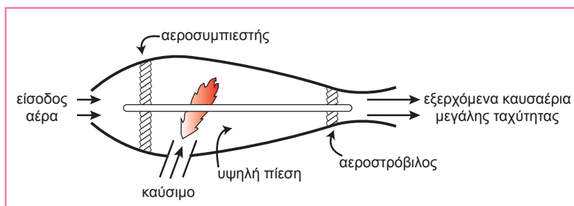
Σχήμα 9.4.8.α: Κινητήρας Turbo-Jet
