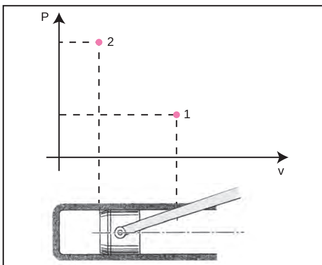
Σχήμα 3.4.β. Διάταξη εμβόλου-κυλίνδρου και καταστατικό διάγραμμα (P-V).
