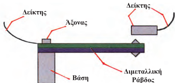
Εικόνα 6: Αρχή λειτουργίας του Διμεταλλικού Θερμόμετρου
