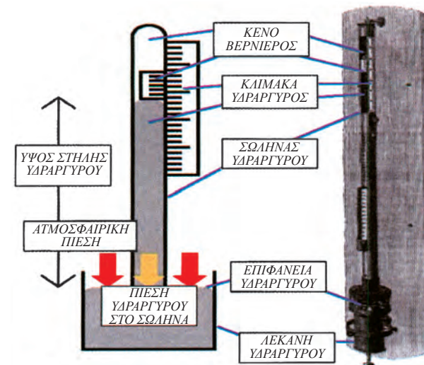
Εικόνα 19: Αρχή λειτουργίας του Υδραργυρικού Βαρόμετρου.
