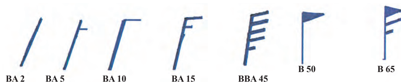
Εικόνα 79: Διανύσματα Ανέμου
