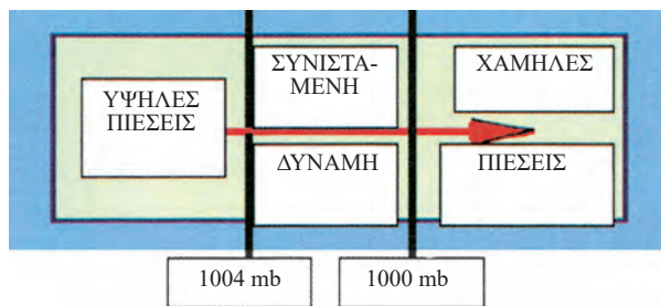
Εικόνα 22: Δύναμη Βαροβαθμίδας
