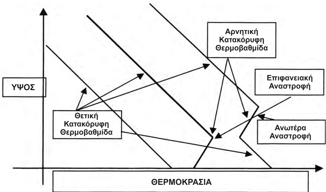
Εικόνα 11: Μεταβολή της Θερμοκρασίας του αέρα με το ύψος στην περίπτωση Θετικής Κατακόρυφης Θερμοβαθμίδας, και στην περίπτωση θερμοκρασιακής αναστροφής (Επιφανειακής και Ανωτέρας). Στη δεύτερη περίπτωση, παρατηρούμε ότι ενώ η θερμοβαθμίδα είναι θετική, σε κάποιο στρώμα αναστρέφεται και γίνεται αρνητική για κάποιο ύψος. Θα δούμε παρακάτω ότι αυτό μπορεί να οφείλεται σε γρήγορη ψύξη του εδάφους μαζί με μικρό στρώμα αέρα. Στην τρίτη περίπτωση, η αναστροφή εμφανίζεται υψηλότερα από το έδαφος και μπορεί να οφείλεται σε θερμό στρώμα αέρα που μεταφέρεται και εναποτίθεται πάνω από το ψυχρότερο.
