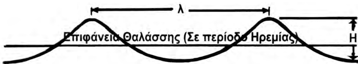
Εικόνα 96: Μήκος Κύματος ( \lambda ), και Ύψος Κύματος ( H ).
