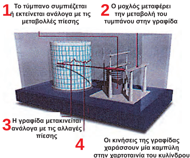
Εικόνα 21: Βαρογράφος
