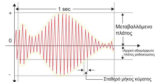
3. Διαμορφωμένο ραδιοκύμα κατά πλάτος - AM
