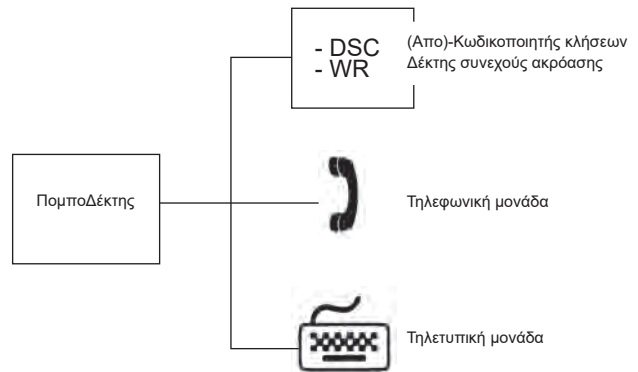
Σχήμα 3γ. Πλήρες σύγχρονο σύστημα συμβατικής ΤΛΦ και ΤΛΠ επικοινωνίας με κλήσεις DSC.
