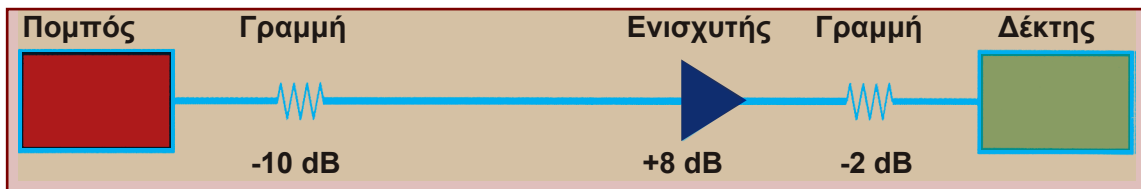
Σχήμα 3.1: Παράδειγμα χρήσης ενισχυτών και απωσβέσεων.
