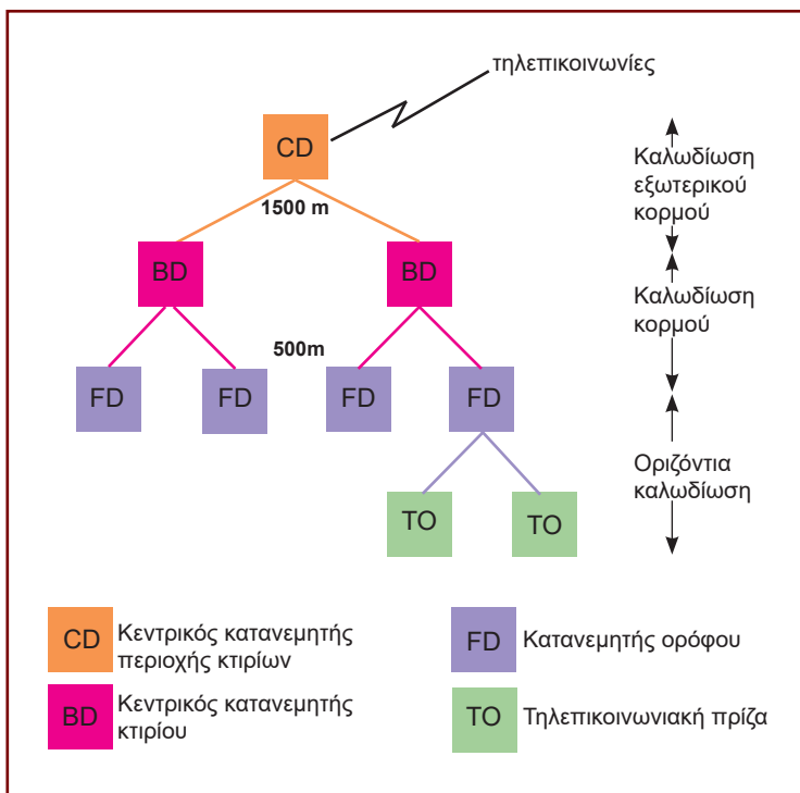
Σχήμα 1.2: Ιεραρχία στο δίκτυο δομημένης καλωδίωσης.
