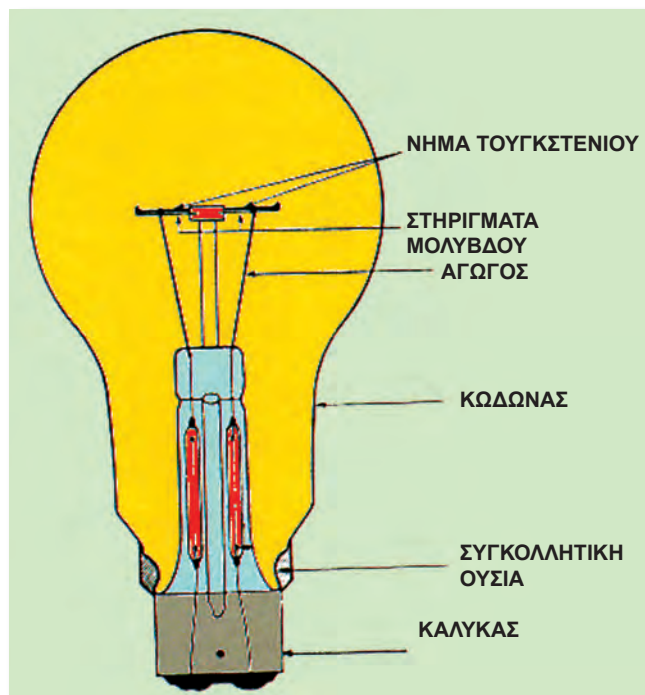
Σχήμα 3.1: Λαμπτήρας πυράκτωσης και τα μέρη που τον αποτελούν
