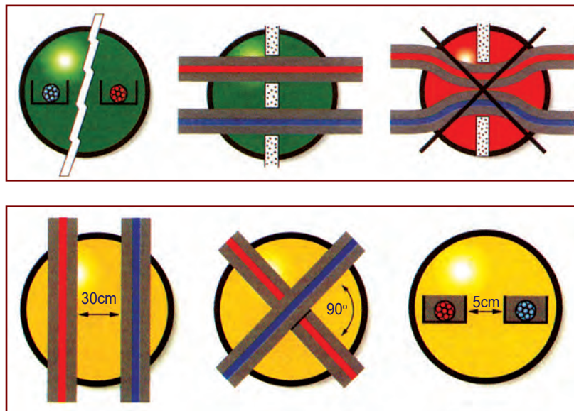
Σχήμα 6.5: Αποφυγή γεινίασης
