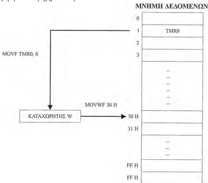
Σχήμα 5.32 Εγγραφή του περιεχομένου του καταχωρητή TMR0 στον καταχωρητή 30 H, με την διαδοχική εκτέλεση των εντολών MOVF TMR0, 0 και MOVWF 30 H.
