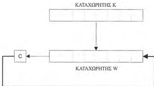
Σχήμα 5.25α Αριστερή περιστροφή του περιεχομένου του καταχωρητή K , μέσω σημαίας C , και αποθήκευση του αποτελέσματος στον καταχωρητή W , με την εντολή RLF K, 0 .
