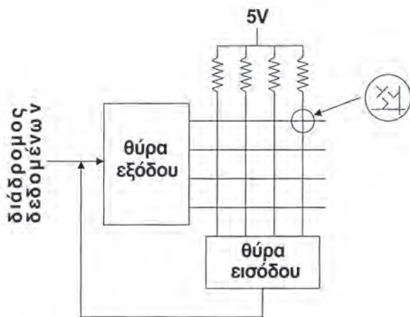
Σχήμα 4.12 Οδήγηση πληκτρολογίου ορθογώνιας διάταξης
