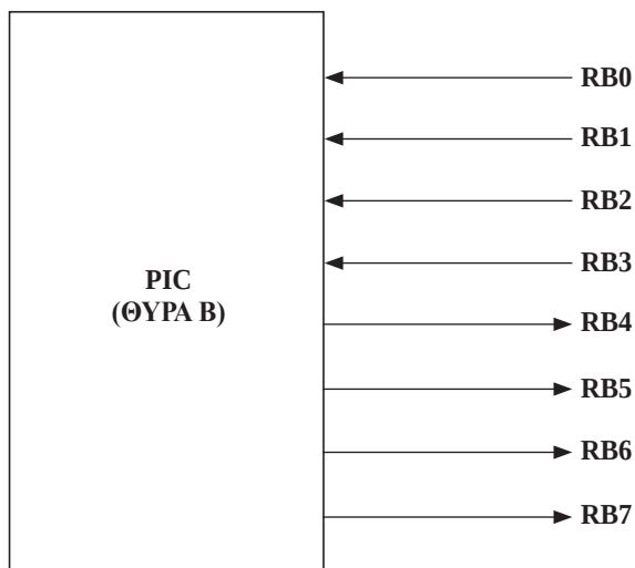
Σχήμα 6.3 Η θύρα B με ορισμό ακροδεκτών RB0 - RB3 ως εισόδοι και RB4 - RB7 ως εξόδοι.
