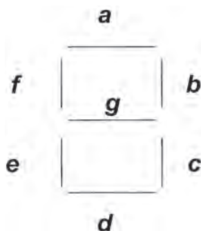
Σχήμα 4.15 Seven Segment Display
