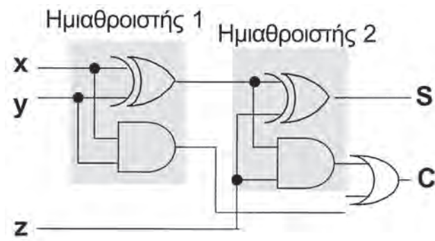
Σχήμα 2.24 Πλήρης αθροιστής υλοποιημένος με ημιαθροιστές
