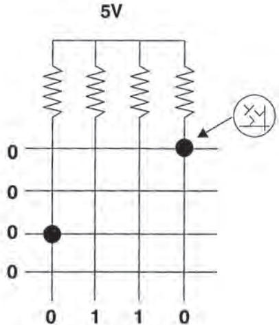
Σχήμα 4.10 Αναγνώριση ότι πατήθηκε πλήκτρο
