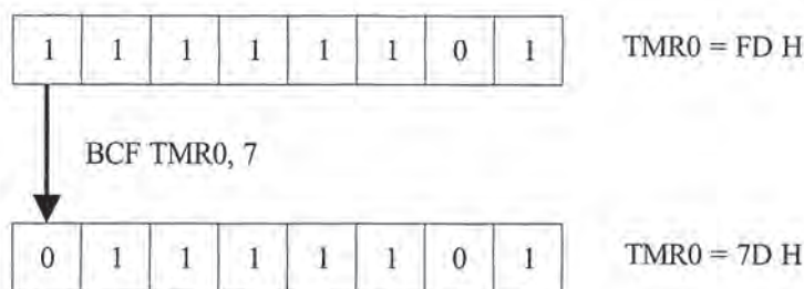
Σχήμα 5.29 Τοποθέτηση του 0 στο 7ο ψηφίο του καταχωρητή TMR0, με την εντολή BCF TMR0, 7.
