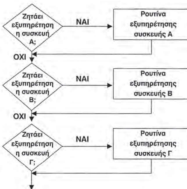
Σχήμα 4.4 Βρόγχος περίοδευσης
