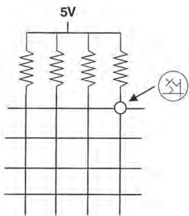
Σχήμα 4.9 Πληκτρολόγιο σε ορθογώνια διάταξη
