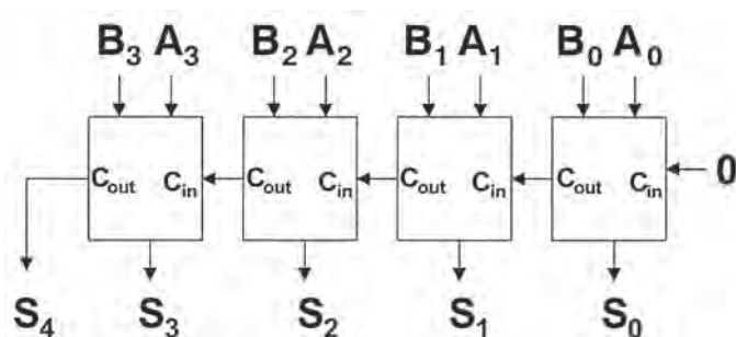
Σχήμα 2.25 Αθροιστής τεσσάρων (4) δυαδικών ψηφίων
