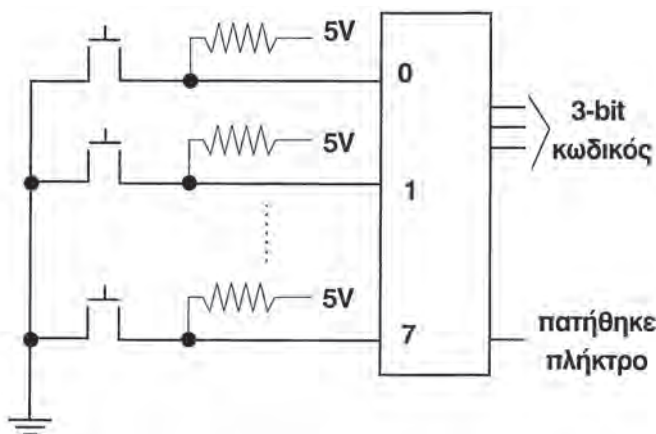
Σχήμα 4.8 Πληκτρολόγιο με γραμμική κωδικοποίηση των πλήκτρων
