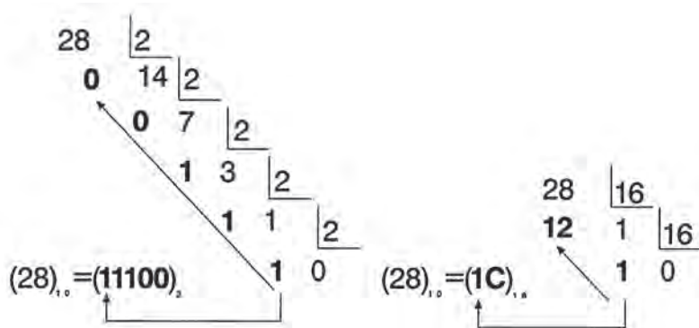
Σχήμα 1.1 Μετατροπή του αριθμού (28)_{10} στο δυαδικό και το δεκαεξαδικό σύστημα αρίθμησης
