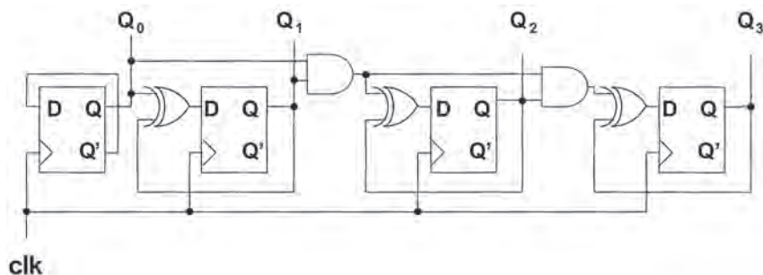
Σχήμα 2.39 Σύγχρονος δυαδικός απαριθμητής τεσσάρων βαθμίδων
