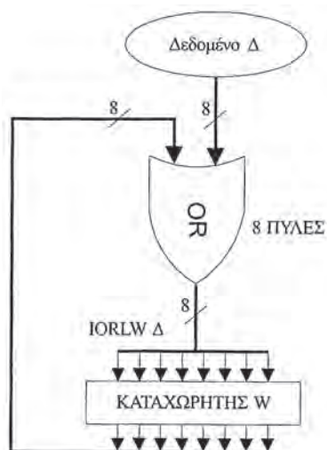
Σχήμα 5.20 Εκτέλεση της λογικής πράξης H μεταξύ του περιεχομένου του καταχωρητή W και του δεδομένου \Delta και αποθήκευση του αποτελέσματος στον W με την εντολή IORLW \Delta .
