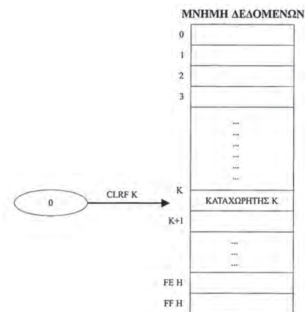
Σχήμα 5.11 Μηδενισμός καταχωρητή K με την εντολή CLRF K.
