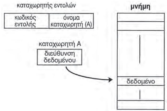
Σχήμα 3.13 Έμμεση αναφορά μέσω καταχωρητή
