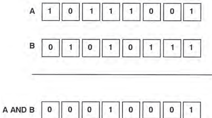
Σχήμα 3.9 Λογική πράξη AND μεταξύ δύο 8-ψήφιων δυαδικών αριθμών
