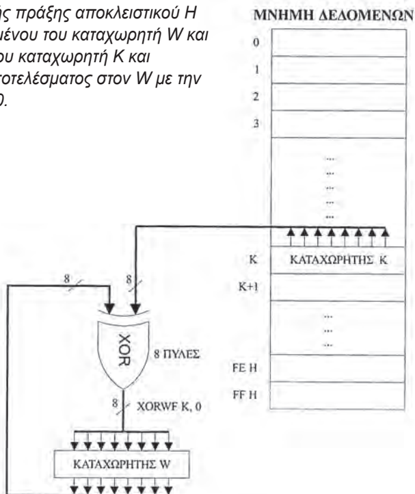
Σχήμα 5.23β Εκτέλεση της λογικής πράξης αποκλειστικού Η μεταξύ του περιεχομένου του καταχωρητή W και του περιεχομένου του καταχωρητή K και αποθήκευση του αποτελέσματος στον K με την εντολή XORWF K, 1.
