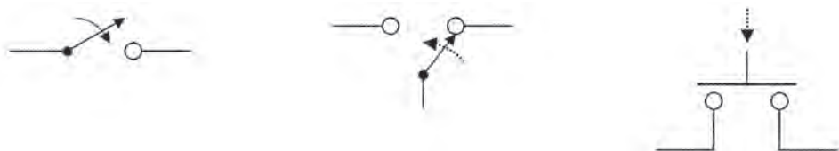
Σχήμα 4.6 Μηχανικοί Διακόπτες
