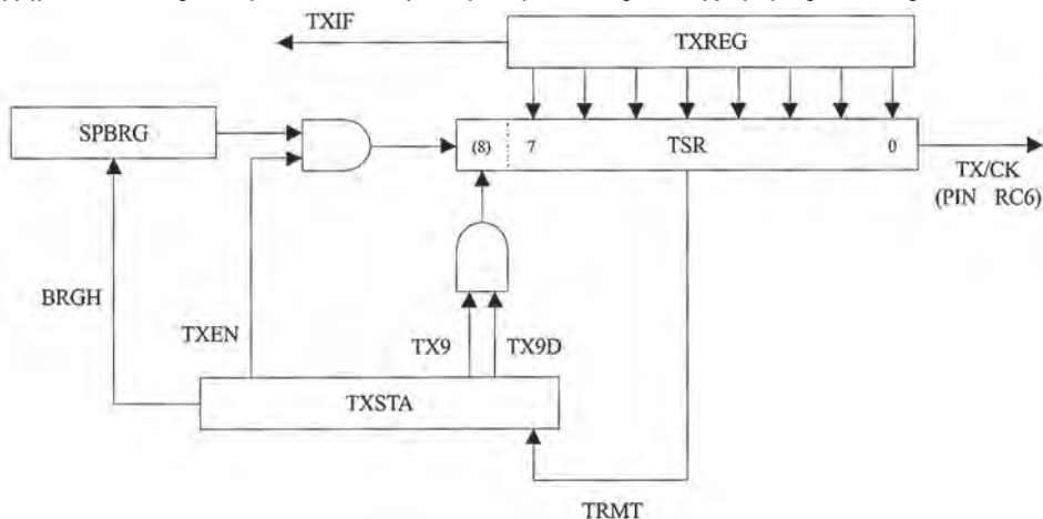
Σχήμα 6.19 Η μονάδα USART σε λειτουργία ασύγχρονης εκπομπής.
