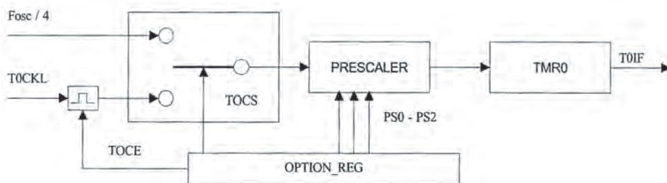
Σχήμα 6.10 Ο χρονιστής TIMER0.
