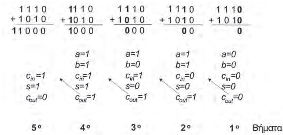
Σχήμα 1.4 Πρόσθεση στο δυαδικό σύστημα
