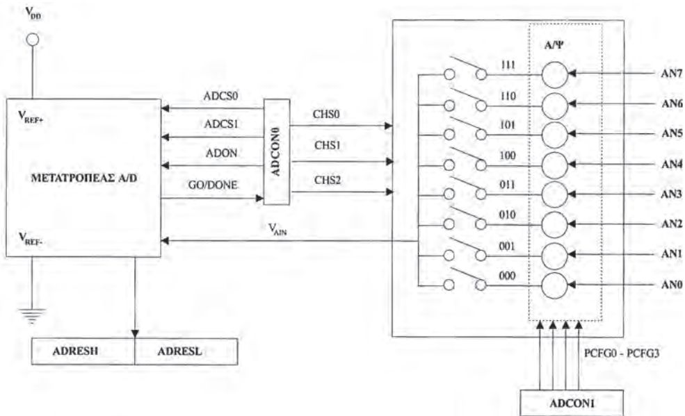
Σχήμα 6.27 Η μονάδα μετατροπής A/D.
