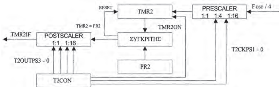
Σχήμα 6.13 Ο χρονιστής TIMER2.
