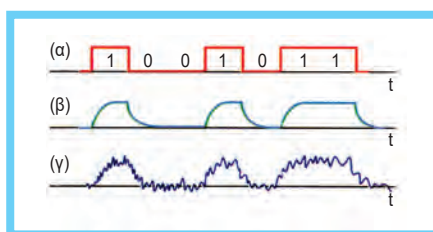
Σχήμα 5.4.2 Αλλοιώσεις κυματομορφής σε ψηφιακά συστήματα: (α) Τυπική μορφή ψηφιακών παλμών, (β) Παραμόρφωση κυματομορφής λόγω περιορισμένης χωρητικότητας καναλιού, (γ) Επίδραση προσθετικού θορύβου.
