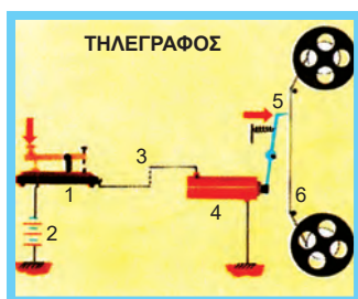
Σχήμα 2.4.2 Σύστημα τηλεγραφικής επικοινωνίας: (1) χειριστήριο, (2) συστοιχία ηλεκτρικών συσσωρευτών, (3) αγωγός σύνδεσης, (4) ηλεκτρομαγνήτης, (5) γραφίδα, (6) χαρτινή ταινία.
