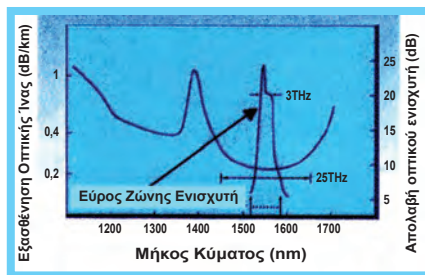
Σχήμα 4.6.1 Η εξασθένηση στην οπτική ίνα έχει ένα ελάχιστο μήκος κύματος 1550 nm, περιοχή στην οποία οι ενισχυτές ίνας προσμείξεων ερβίου εμφανίζουν τη μέγιστη απολαβή τους.
