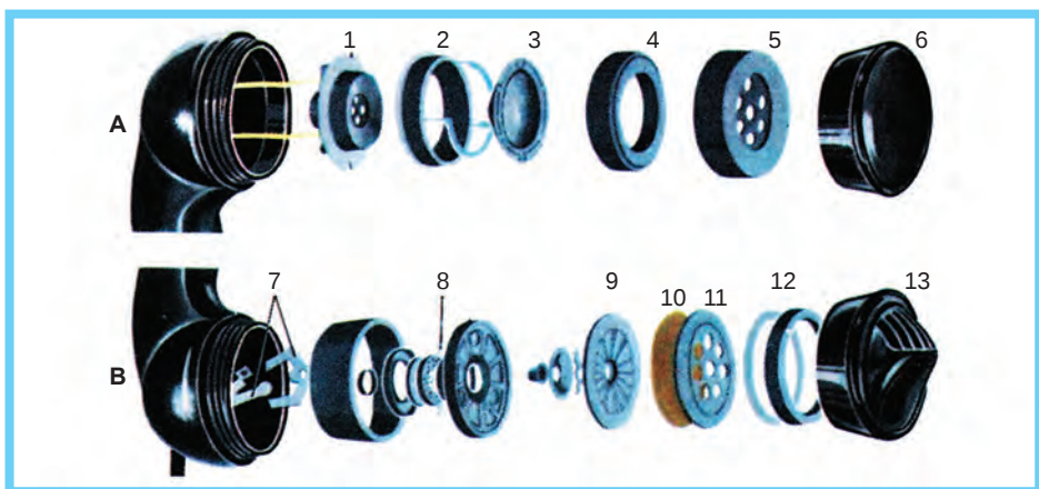
Σχήμα 6.1.3 Τα εξαρτήματα του μικροτηλέφωνου.
