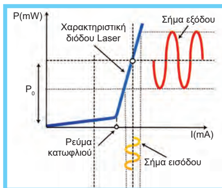
Σχήμα 4.4.8 Χαρακτηριστική οπτικής ισχύος εκπομπής - ρεύματος πόλωσης δίοδου Laser. Η διαμόρφωση του ρεύματος οδήγησης της Laser από το σήμα πληροφορίας μετατρέπεται από το γραμμικό τμήμα της καμπύλης σε αντίστοιχες διακυμάνσεις της οπτικής ισχύος εξόδου.
