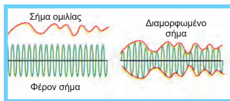
Σχήμα 6.2.1 Διαβίβαση ηλεκτρικού ρεύματος τηλεφωνικής ομιλίας πάνω σε ρεύμα υψηλής συχνότητας (φέρον σήμα).
