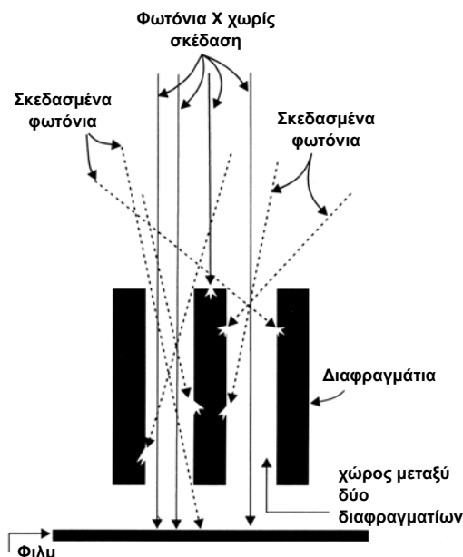
Σχήμα 7.6 Η αντισκεδαστική δράση των διαφραγμάτων. Ανεξάρτητα από το αν η κάθε ακτίνα έχει σκεδαστεί ή όχι, αν συναντήσει διαφραγμάτιο στην πορεία της, θα απορροφηθεί. (Δ. Κατσιφαράκης, Αρχές Ακτινογραφικής Απεικόνισης).
