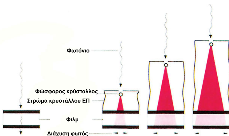
Σχήμα 8.4 Όσο αυξάνεται το πάχος του φθορίζοντος υλικού προκαλείται μεγαλύτερη διάχυση του φωτός, άρα και μεγαλύτερη απώλεια της απεικονιζόμενης λεπτομέρειας.
