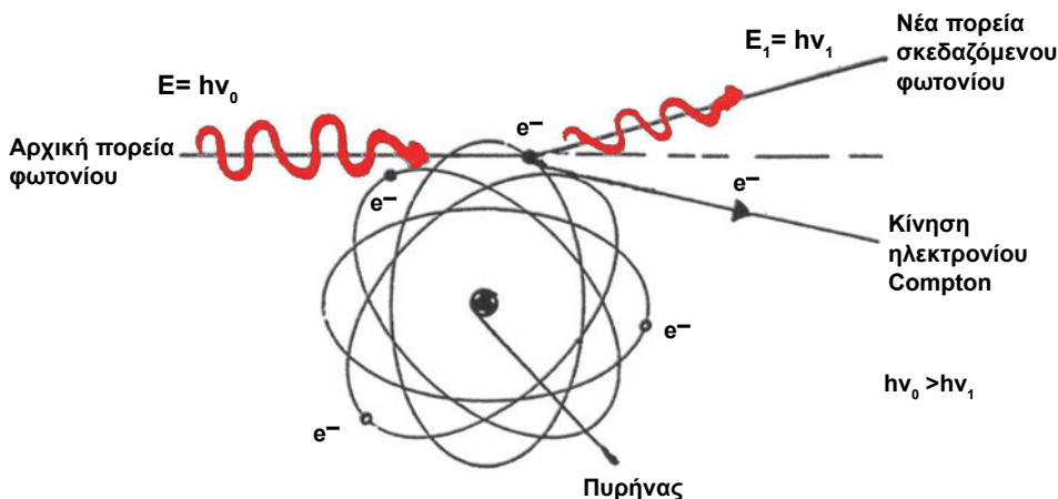
Σχήμα 3.3 Φαινόμενο Compton.
