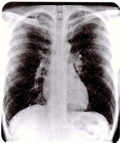
Εικόνα 12.16 Ακτινογραφία θώρακα.
