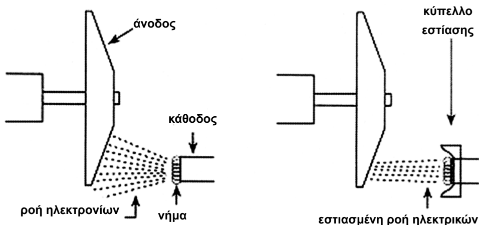
Σχήμα 5.5 Κύπελλο εστίασης.
