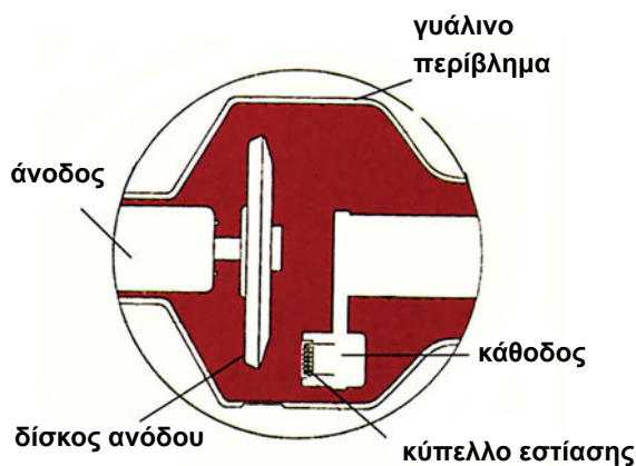
Σχήμα 5.6 Άνοδος.
