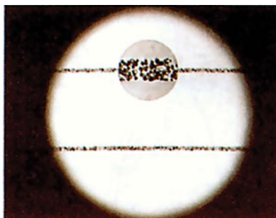
Σχήμα 8.5 Αριστερά σχηματική παράσταση της δομής του ακτινολογικού φιλμ. Στη δεξιά φωτογραφία, απεικονίζεται το φωτογραφικό γαλάκτωμα φιλμ διπλής επίστρωσης. Στην ένθετη κυκλική μεγέθυνση μια μικροφωτογραφία του γαλακτώματος.
