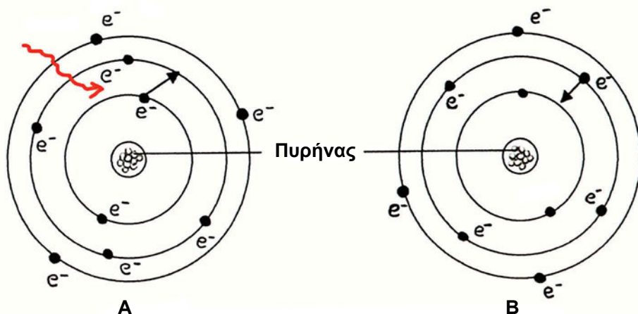
Σχήμα 1. 3 Διέγερση και αποδιέγερση του ατόμου.
