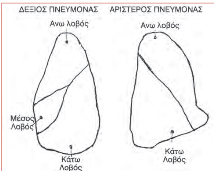
Σχήμα 12.2 Πνεύμονες
