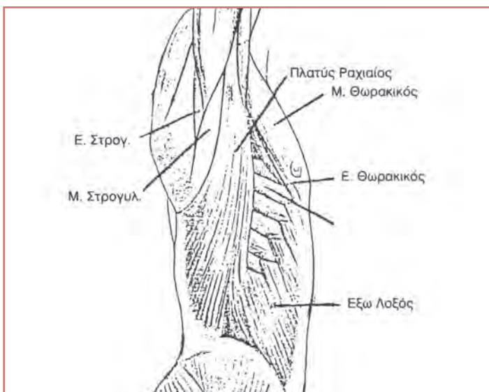
Σχήμα 12.1 Μύες αναπνοής
