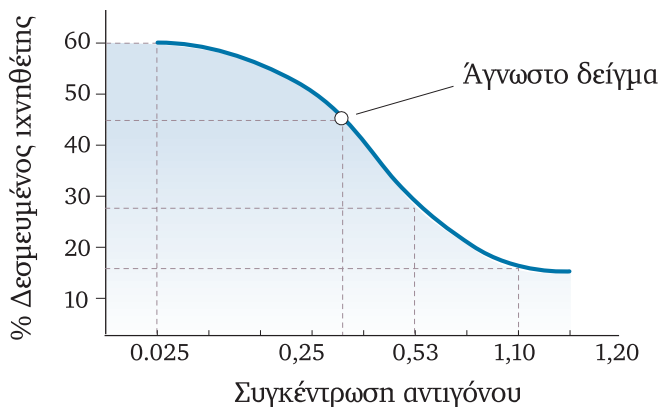
Εικόνα 15.4 Πρότυπη καμπύλη σε Ραδιοαναστολογική ανάλυση (RIA).
