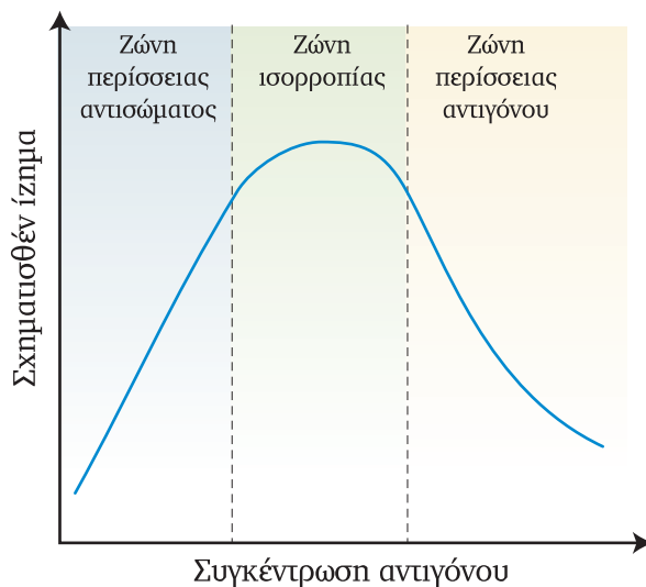
Σχήμα 11.1 Καμπύλη ποσοτικής ιζηματινοαντίδρασης (Heidelberger-Kendall).
