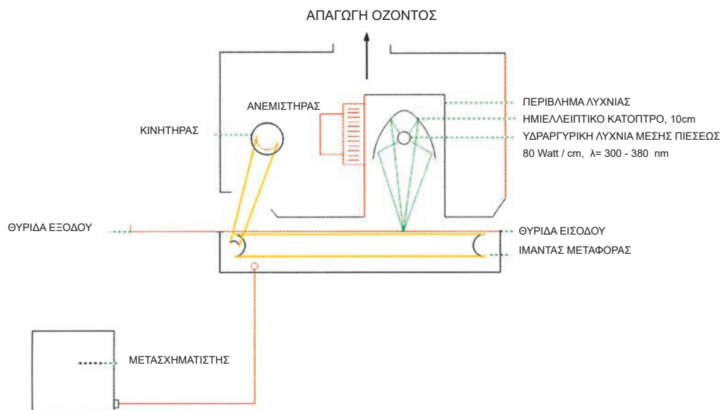
Σχήμα 12.1 Μονάδα υπεριώδους ακτινοβολίας (UV)
