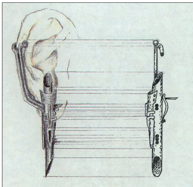
Εικ. 1.30 Σχέδιο για "καθιστά" σκουλαρίκια σε χρυσό. Κάτοψη και πλάγια όψη.
