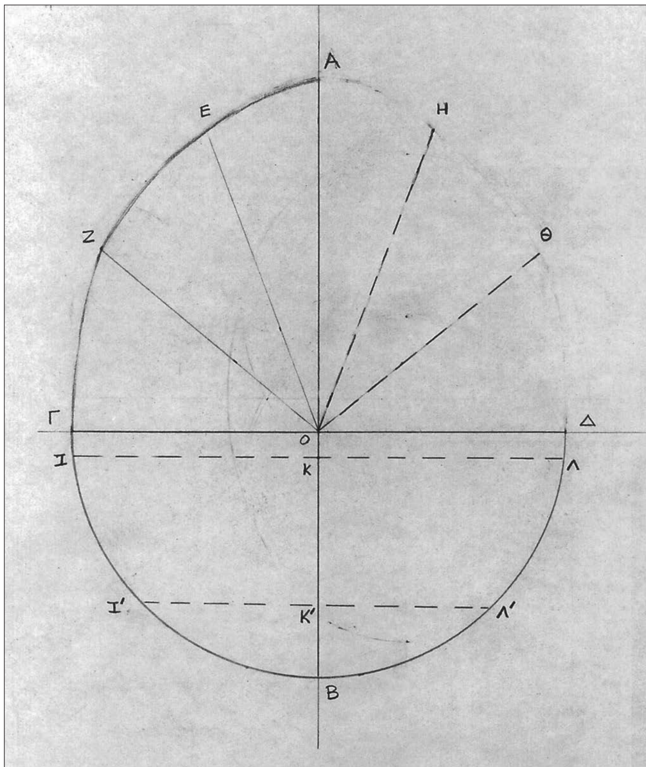
Εικ. 1.77 Γεωμετρική κατασκευή για ειδικό τύπο ωοειδούς περιδέραιον, σε φυσικό μέγεθος.
