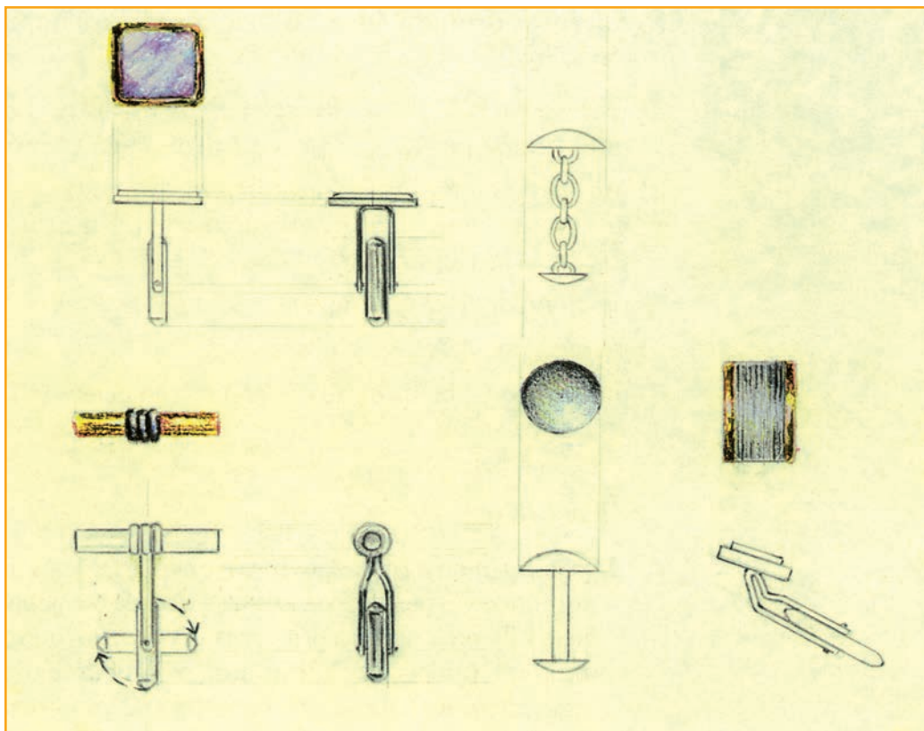
Εικ. 6.4 Σχέδια για μανικετόκουμπα, με πλάγιες όψεις.
