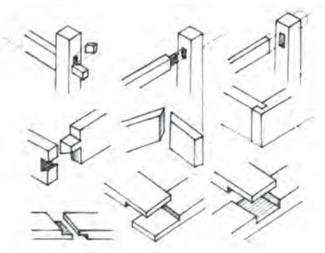
Σχήμα 8.5. Σχηματική παράσταση διάφορων παραδειγμάτων "σύνδεσης" ξύλινων τμημάτων
