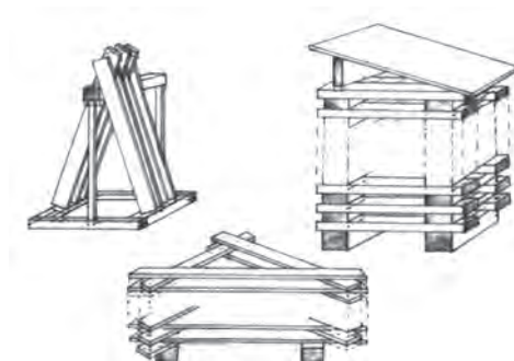
Σχήμα 8.4. Σχηματική παράσταση παραδειγμάτων φυσικής ξήρανσης ξυλείας
