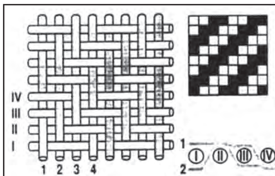
Σχήμα 9.6.: Ύφασμα με διαγώνιες ραβδώσεις (twill) παράγεται, όταν νήματα υφιδιού περνούν με εναλλαγή πάνω και κάτω από δύο ή περισσότερα στημόνια. Τα σημεία που διασταυρώνονται υφάδια και στημόνια σχηματίζουν διαγώνιες. Μπορούν έτσι να δημιουργηθούν διάφορες υφάνσεις αυτού του τύπου.
