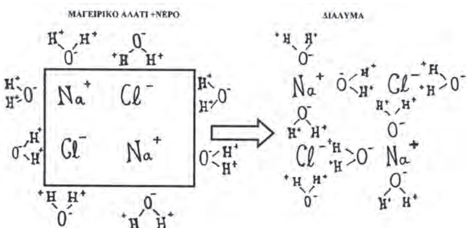
Σχήμα 6.1.: Διάλυμα μαγειρικού αλατιού ( \text{NaCl} ) σε νερό ( \text{H}_2\text{O} ). Τα μόρια του \text{H}_2\text{O} , που χαρακτηρίζονται από μεγάλη πολικότητα, διεισδύουν στον κρύσταλλο του \text{NaCl} , προσανατολισμένα με τον ηλεκτροθετικό πόλο τους προς το ηλεκτραρνητικό ιόν \text{Cl}^- και με τον ηλεκτραρνητικό πόλο τους προς το ηλεκτροθετικό ιόν του \text{Na}^+ . Οι δεσμοί ανάμεσα στα ιόντα \text{NaCl} σπάζουν και με την προσθήκη και άλλων μορίων \text{H}_2\text{O} ανάμεσα στα ιόντα \text{NaCl} επέρχεται η πλήρης διάλυση του μαγειρικού αλατιού ( \text{NaCl} ).
