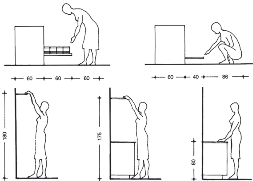
128. Χώρος προετοιμασίας του φαγητού. Μετρικές σχέσεις.
