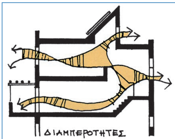
48. Δροσισμός και αερισμός, που εξασφαλίζονται από τη διαπεροπτικότητα του χώρου, χάρη στα ανοίγματα που υπάρχουν στις δύο αντίθετες πλευρές του.
