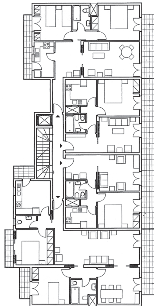
26. Η εμπορική πολυκατοικία. Κάτοψη.
