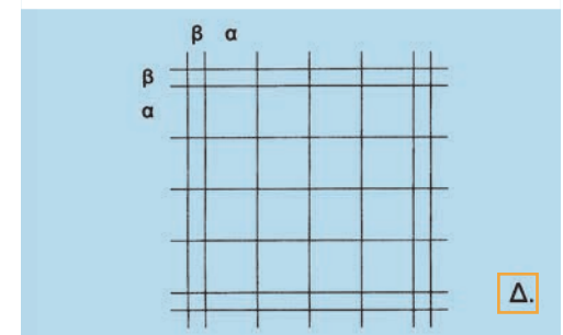
55. Τα είδη του κανάβου: Α. τετραγωνικός, Β. ορθογωνικός, Γ. τριγωνικός, Δ. με ζώνες υποστυλωμάτων.
