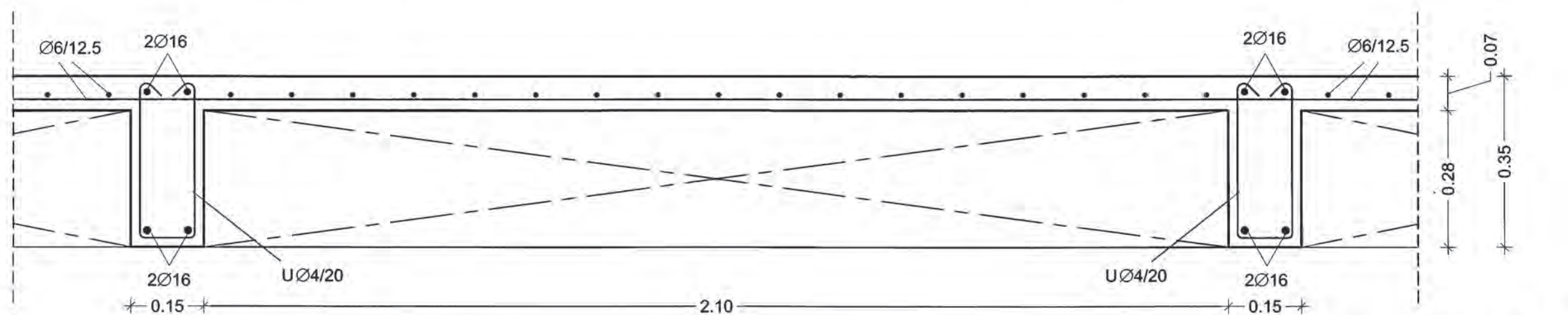
ΛΕΠΤΟΜΕΡΕΙΑ Β ΚΛ. 1:10
