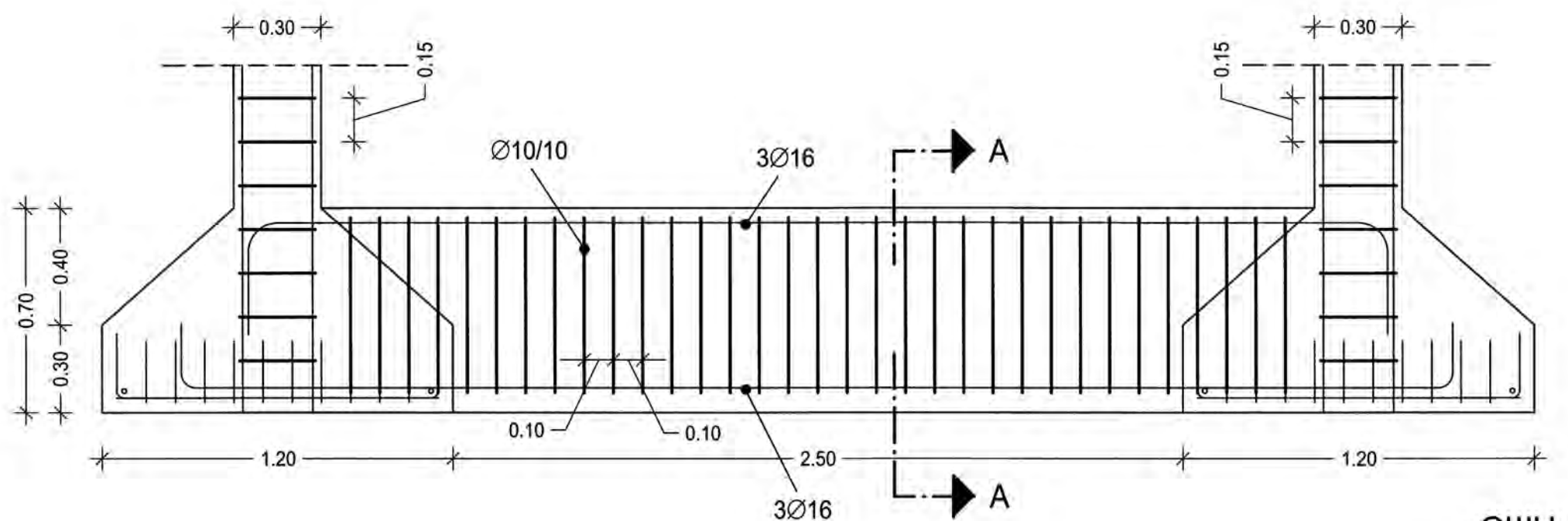
ΟΨΗ ΚΛ. 1:20
