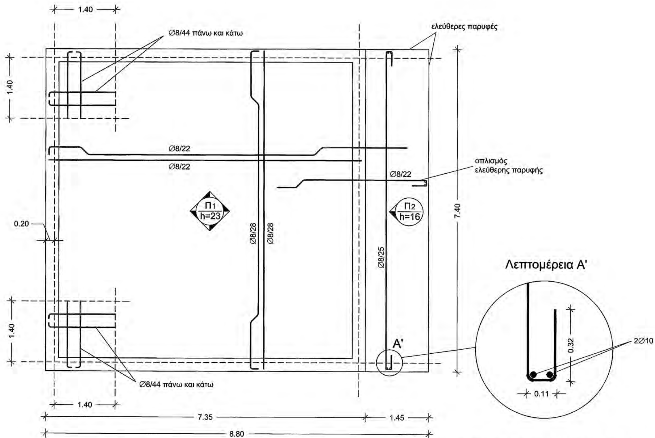
ΕΥΛΟΤΥΠΟΣ ΤΕΤΡΑΕΡΕΙΣΤΗΣ ΠΛΑΚΑΣ ΜΕ ΠΡΟΒΟΛΟ ΚΛΙΜΑΚΑ 1:50
