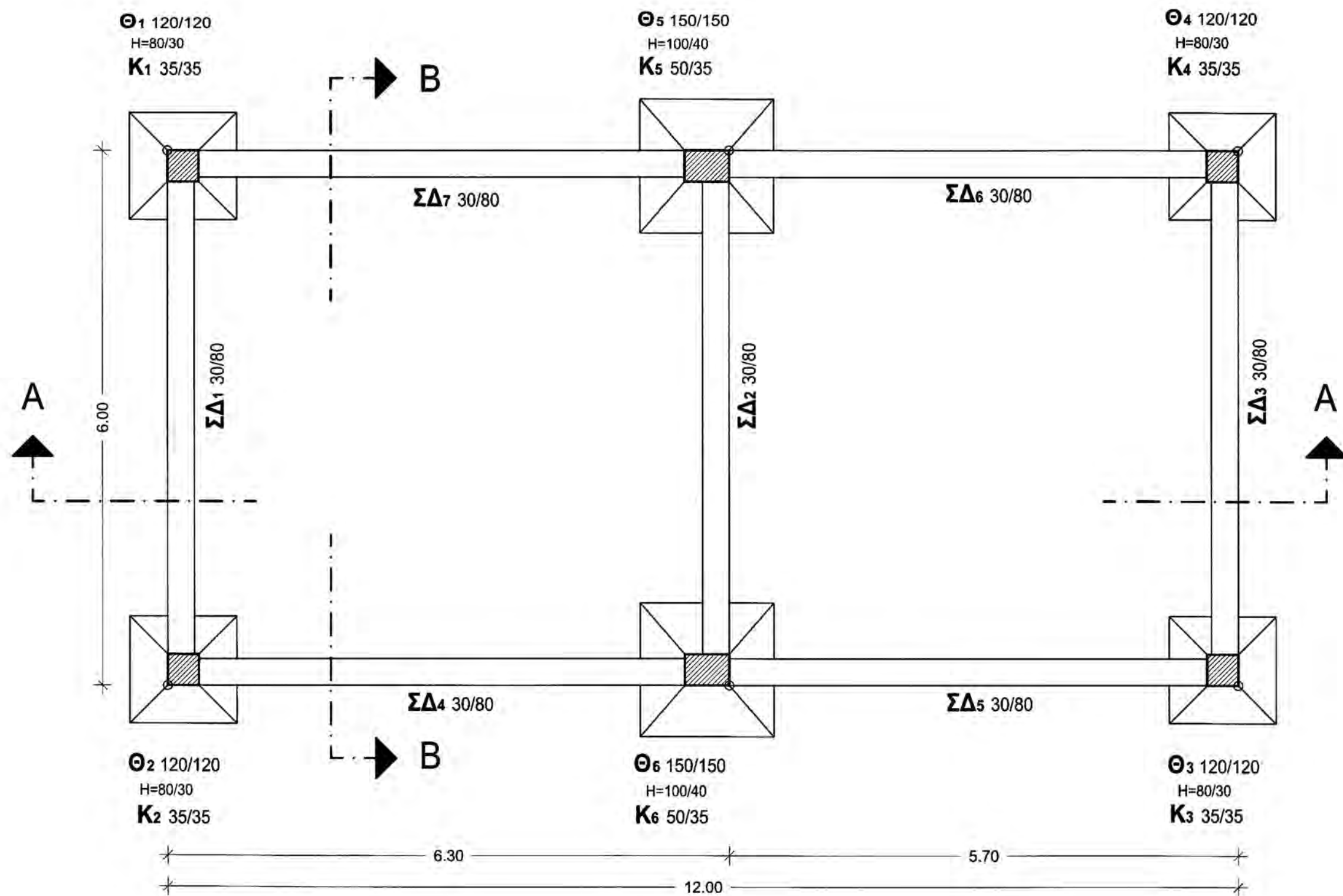
ΞΥΛΟΤΥΠΟΣ ΘΕΜΕΛΙΩΣΗΣ (ΜΑΡΑΓΚΟΥ) ΚΛΙΜΑΚΑ 1:50
