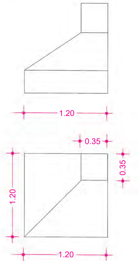
πέδιλο έκκεντρο κατά δύο κατευθύνσεις
