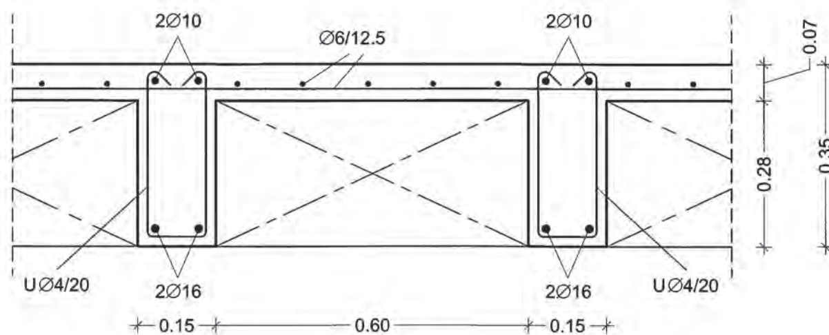
ΛΕΠΤΟΜΕΡΕΙΑ Α ΚΛ. 1:10
