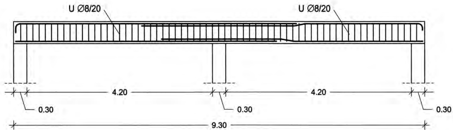
ΤΟΜΗ Κλίμακα 1:50
