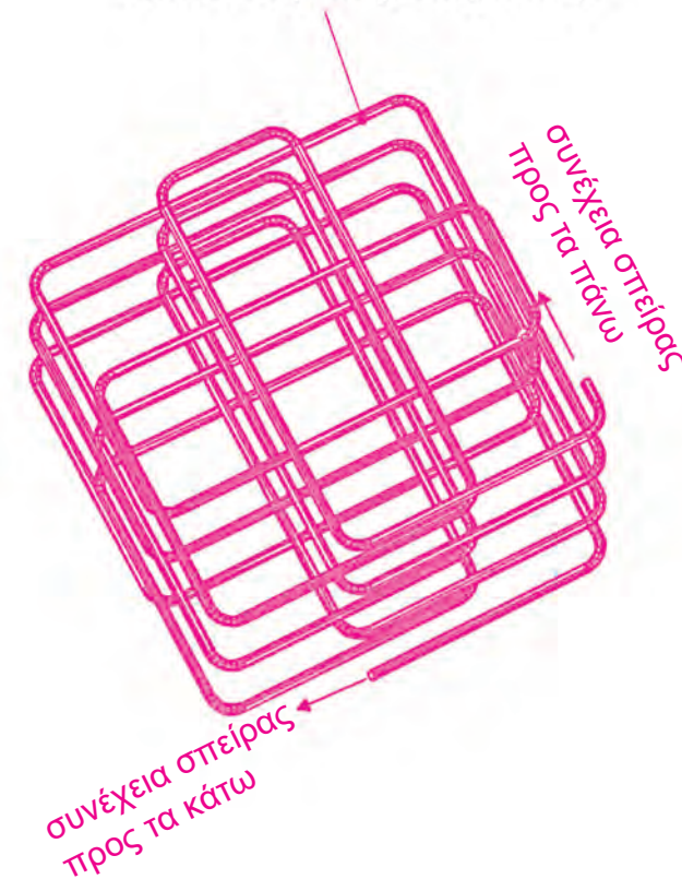
Αντισεισμικός Θώρακας
