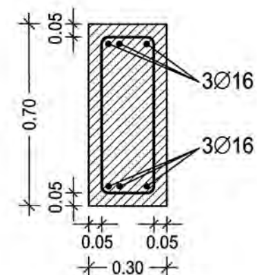
ΤΟΜΗ Α - Α ΚΛ. 1:20
